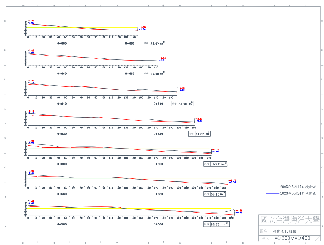
圖 4-5(b) 2023 年 6 月 24 日 B 監測區橫斷面比較圖
