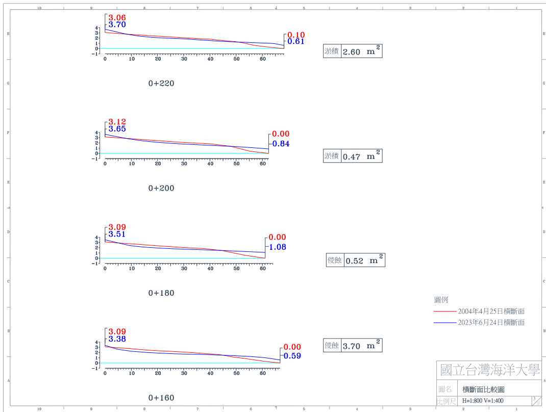
圖 4-4(h) 2023 年 6 月 24 日 A 監測區橫斷面比較圖
