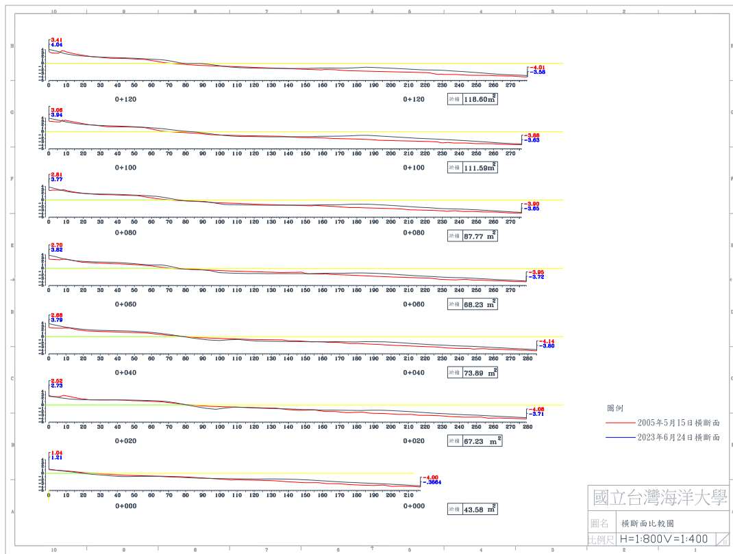
圖 4-5(f) 2023 年 6 月 24 日 B 監測區橫斷面比較圖
