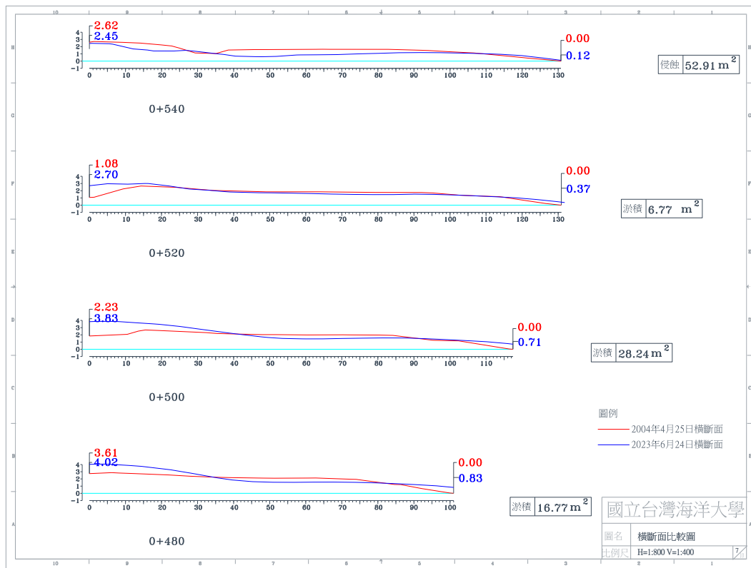
圖 4-4(d) 2023 年 6 月 24 日 A 監測區橫斷面比較圖
