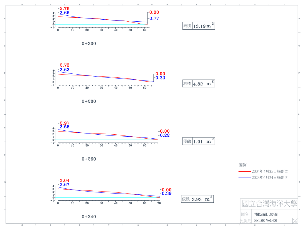
圖 4-4(g) 2023 年 6 月 24 日 A 監測區橫斷面比較圖
