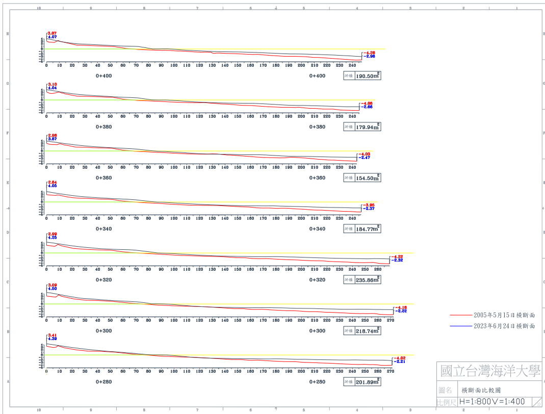
圖 4-5(d) 2023 年 6 月 24 日 B 監測區橫斷面比較圖
