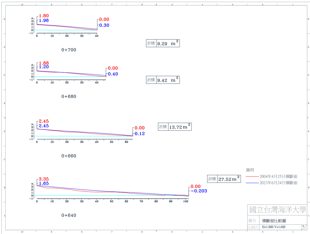
圖 4-4(b) 2023 年 6 月 24 日 A 監測區橫斷面比較圖
