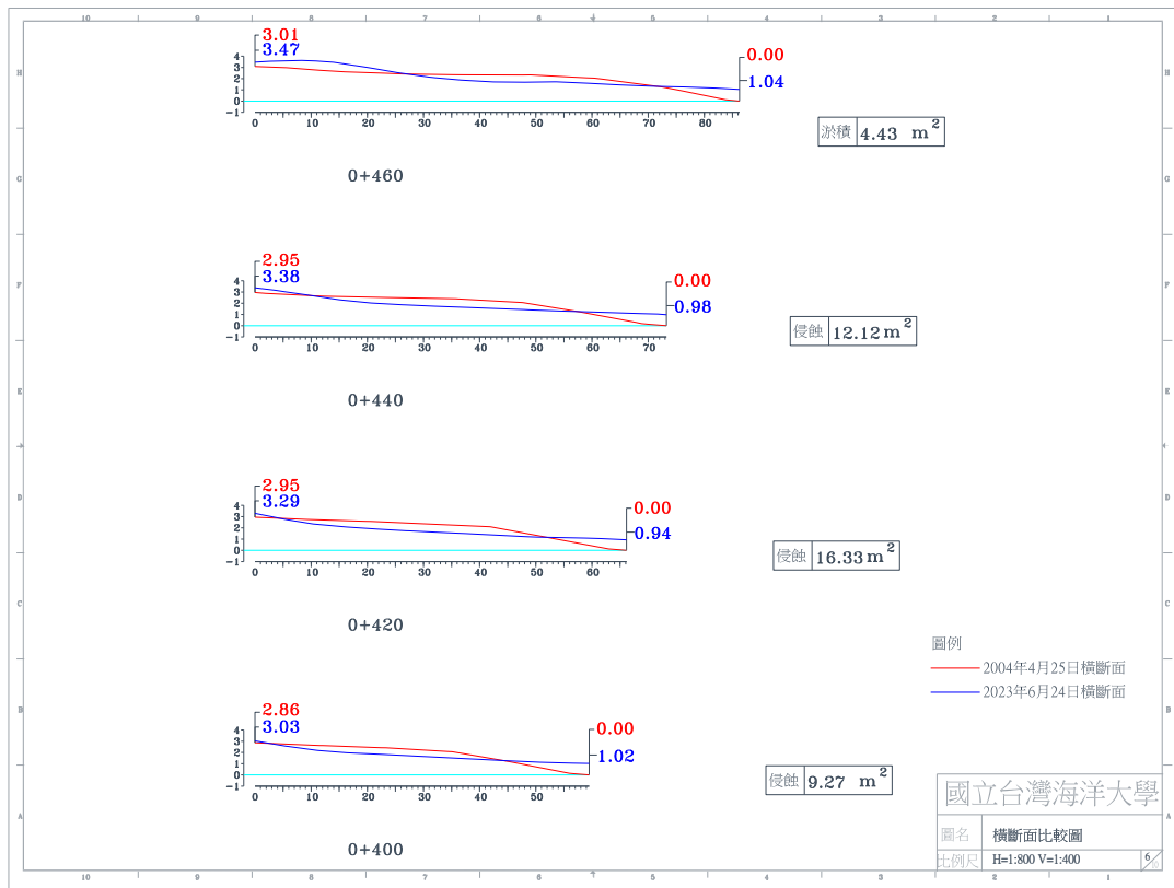
圖 4-4(e) 2023 年 6 月 24 日 A 監測區橫斷面比較圖
