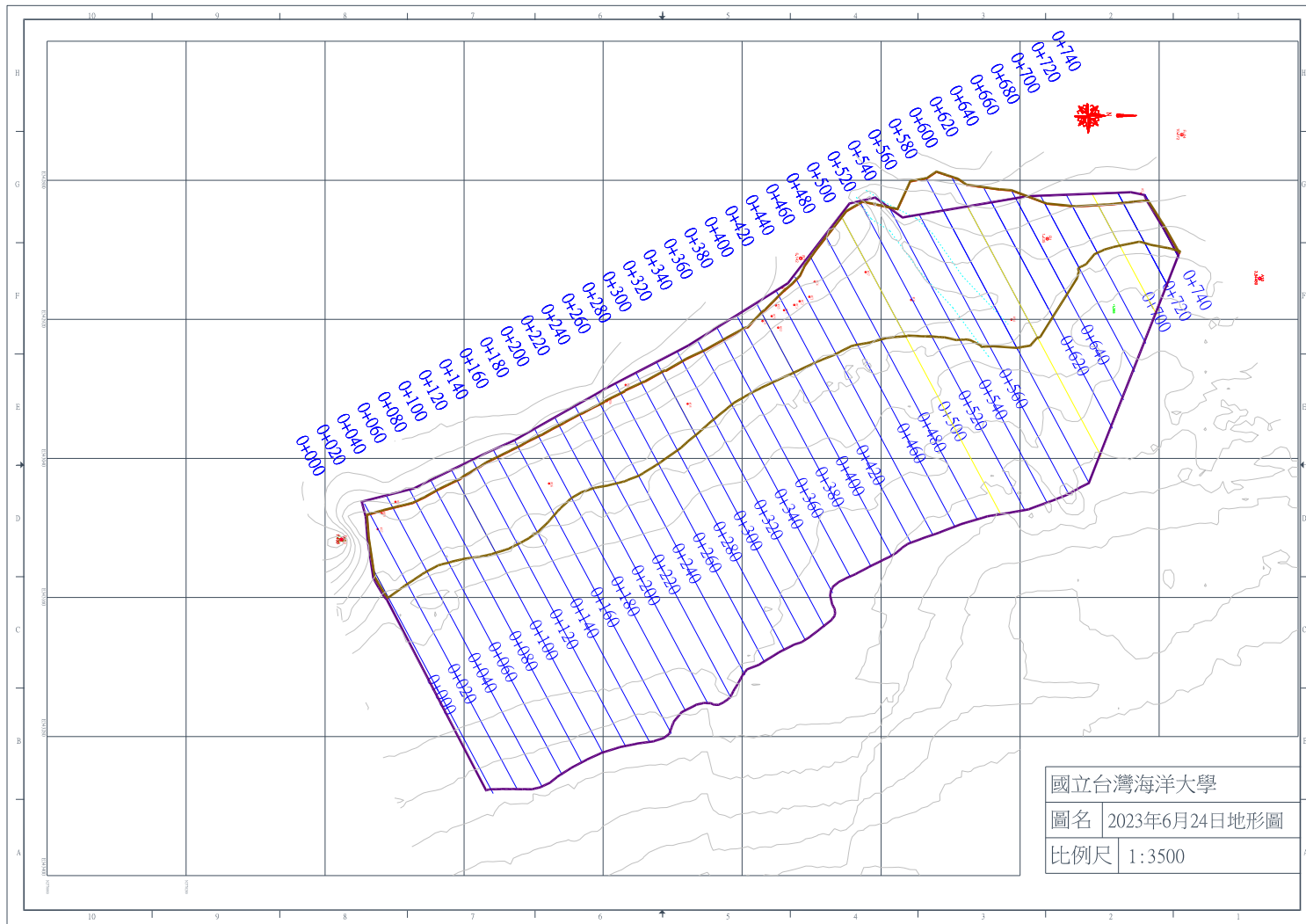
圖 4-1 2023 年 6 月 24 日監測地形
