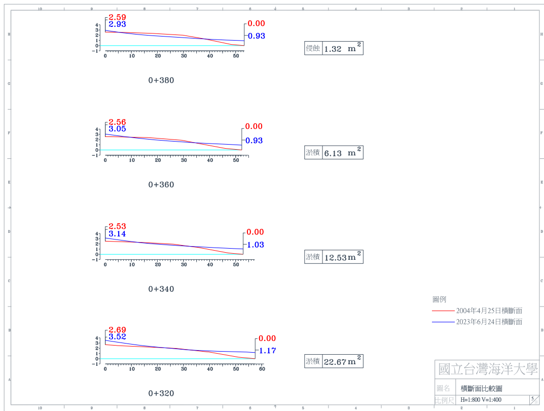
圖 4-4(f) 2023 年 6 月 24 日 A 監測區橫斷面比較圖
