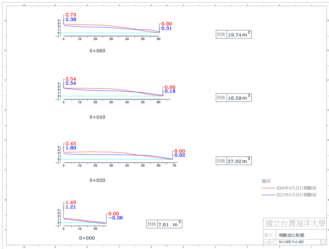
圖 4-4(j) 2023 年 6 月 24 日 A 監測區橫斷面比較圖
