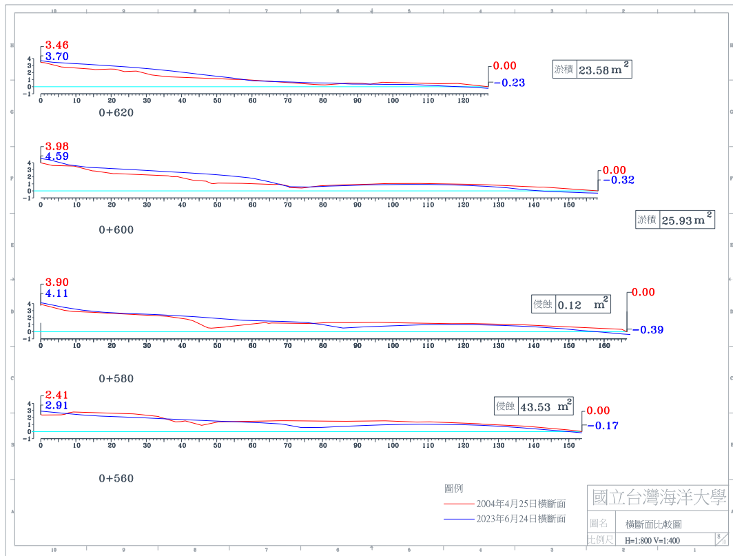
圖 4-4(c) 2023 年 6 月 24 日 A 監測區橫斷面比較圖
