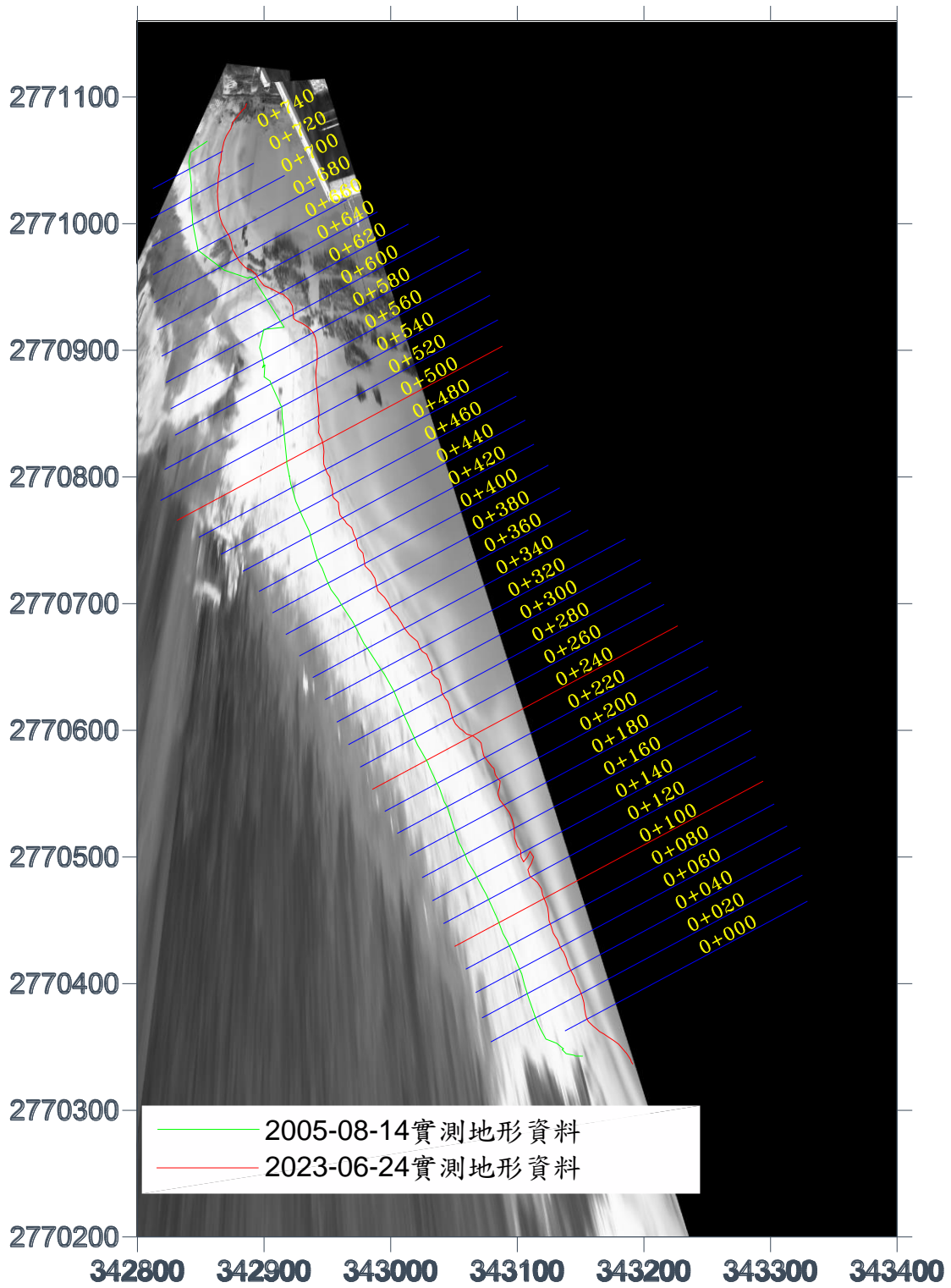
圖 4-22 長期實測 0 m 灘線比對平面示意圖(2023/06/24)
