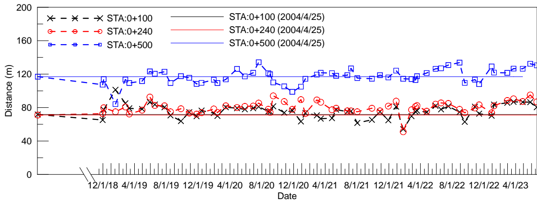
圖 4-21 岸線斷面沙灘寬度變化圖(2023/06/21)
