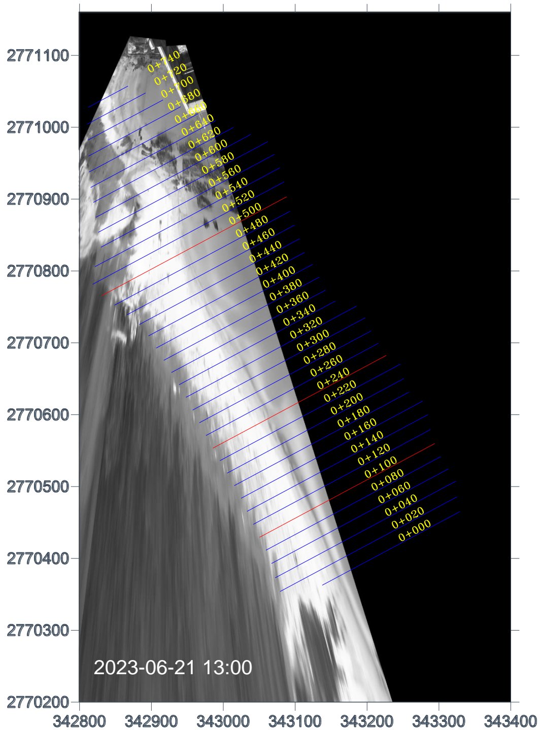
圖 4-19 鹽寮海岸地形影像全景圖(2023/06/21 13:00)
