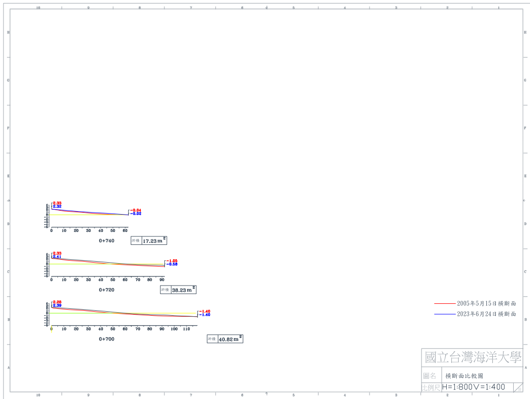
圖 4-5(a) 2023 年 6 月 24 日 B 監測區橫斷面比較圖
