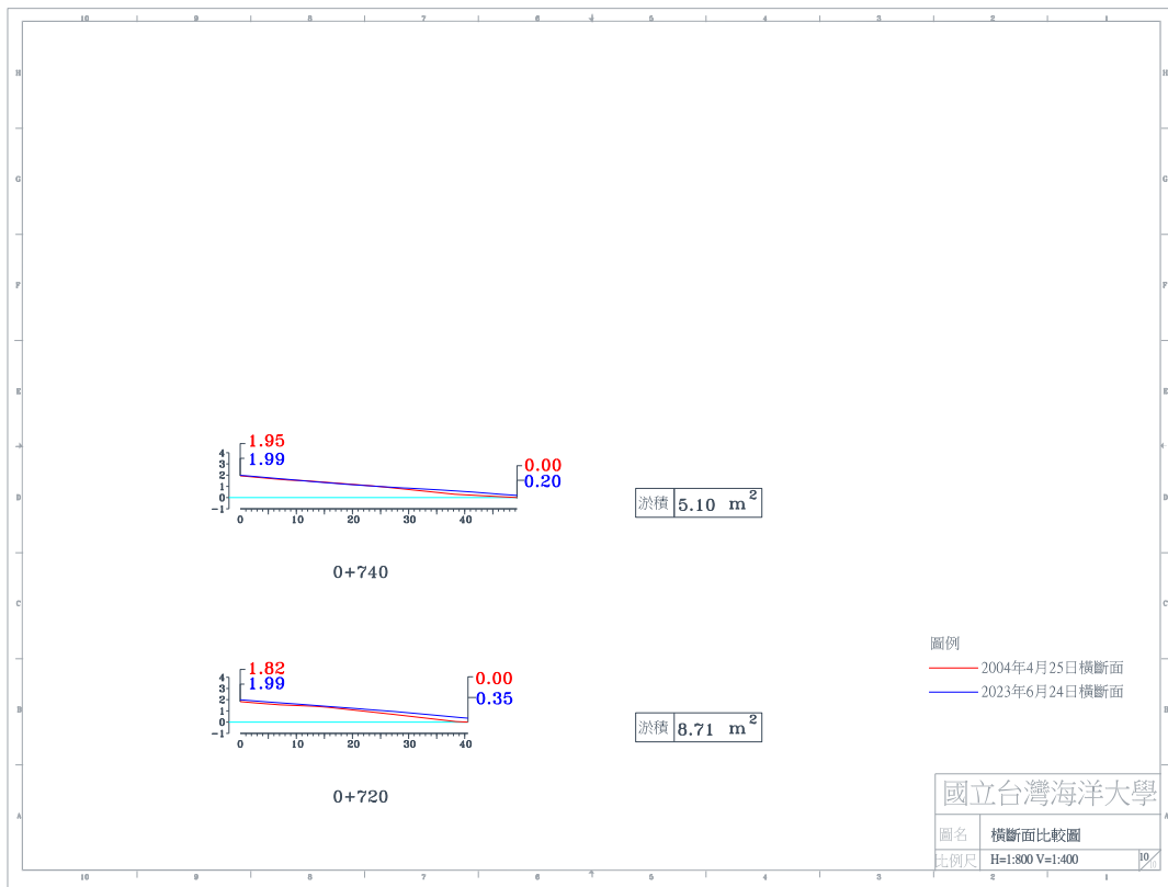
圖 4-4(a) 2023 年 6 月 24 日 A 監測區橫斷面比較圖
