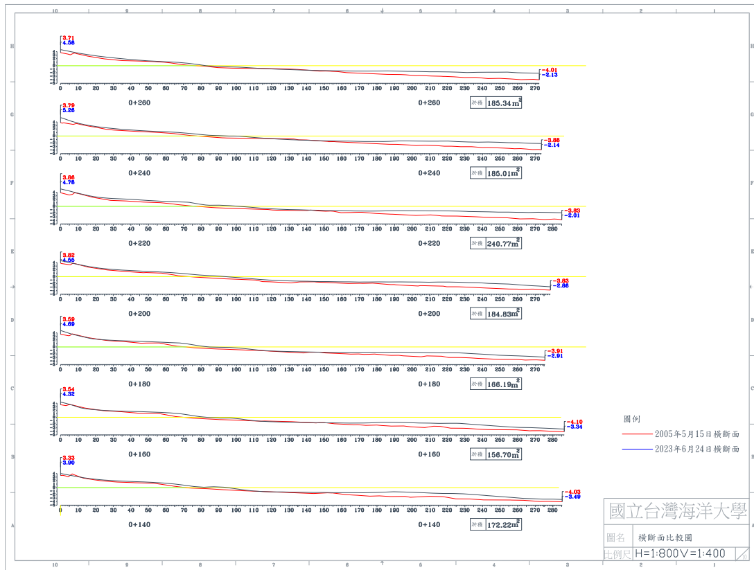
圖 4-5(e) 2023 年 6 月 24 日 B 監測區橫斷面比較圖
