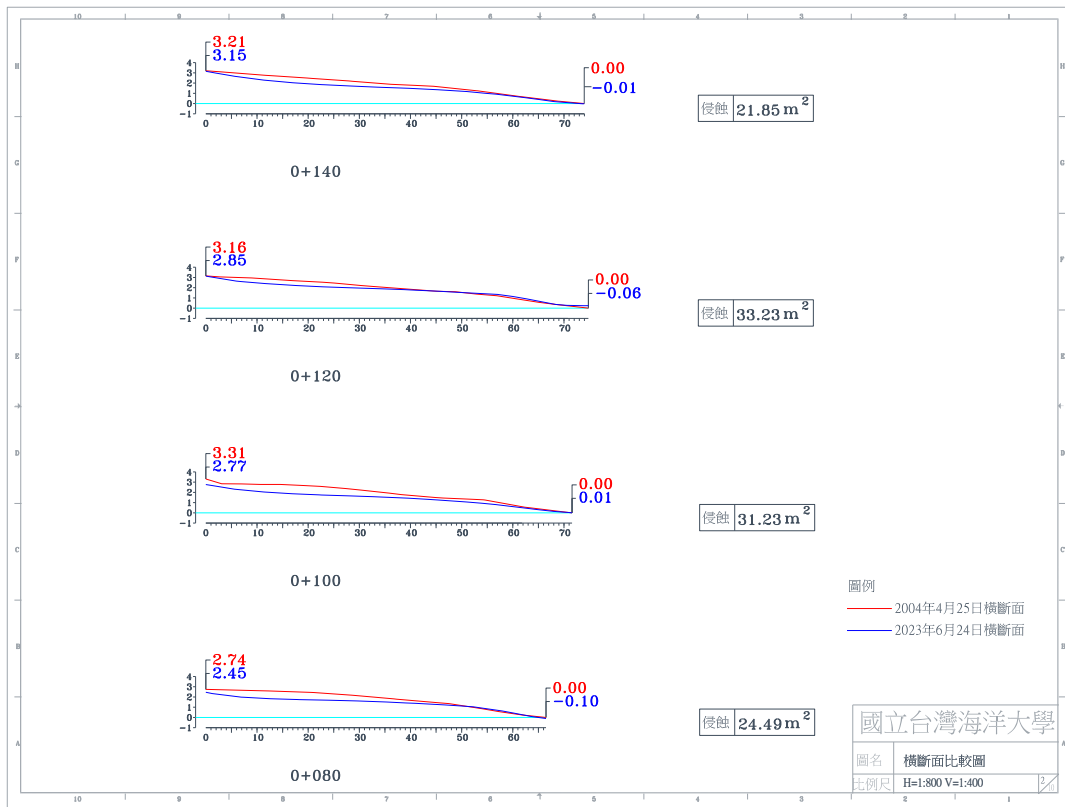
圖 4-4(i) 2023 年 6 月 24 日 A 監測區橫斷面比較圖
