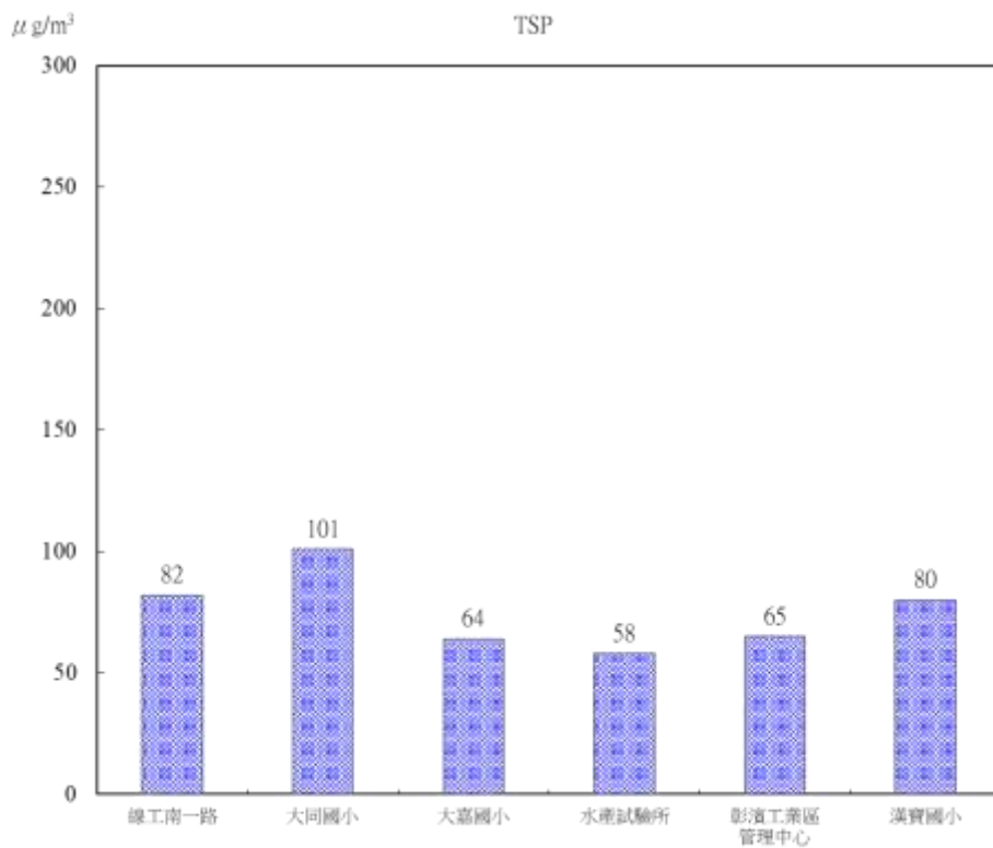
圖 2.1-8 本季各測站 TSP24 小時值監測結果比較分析圖
