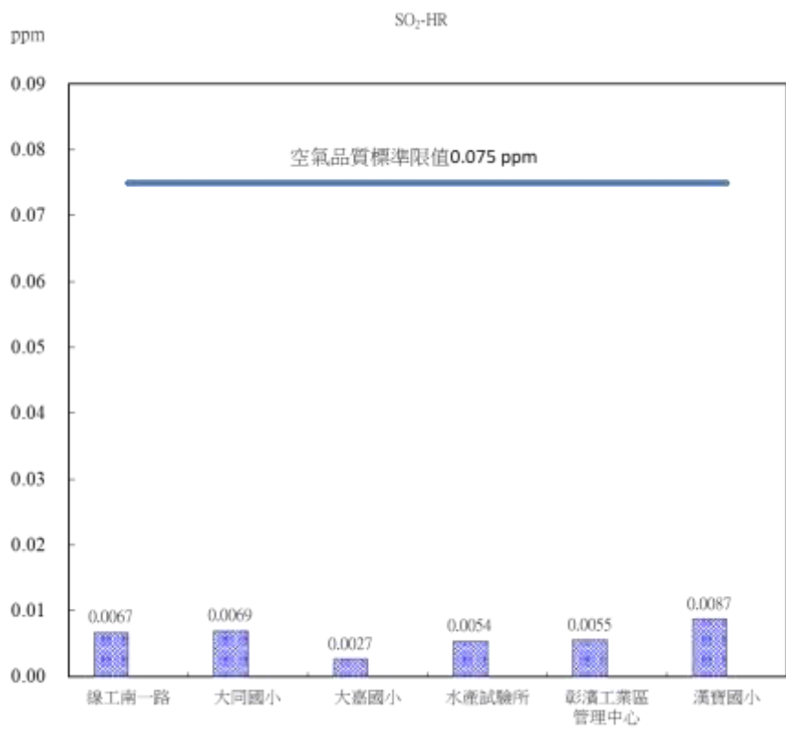
圖 2.1-4 本季各測站 SO 2 最高小時值監測結果比較分析圖
