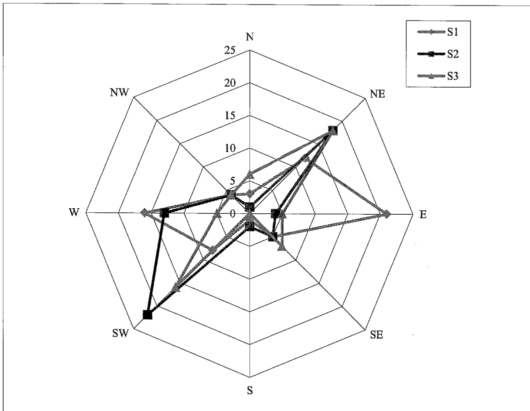
圖 3.1-40 各測站主要輸砂來向歷年累計次數雷達圖
