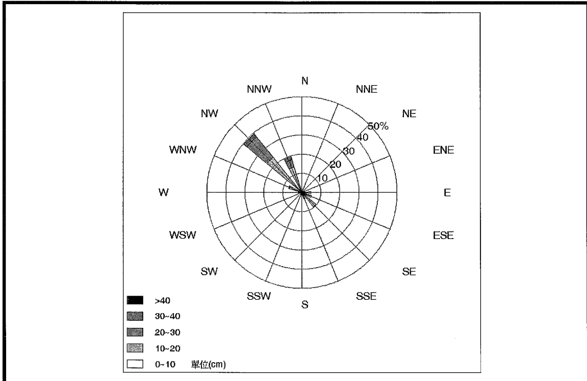
圖2.15-3 核四施工期間環境監測103年第3季海流儀實測流速流向玫瑰圖
