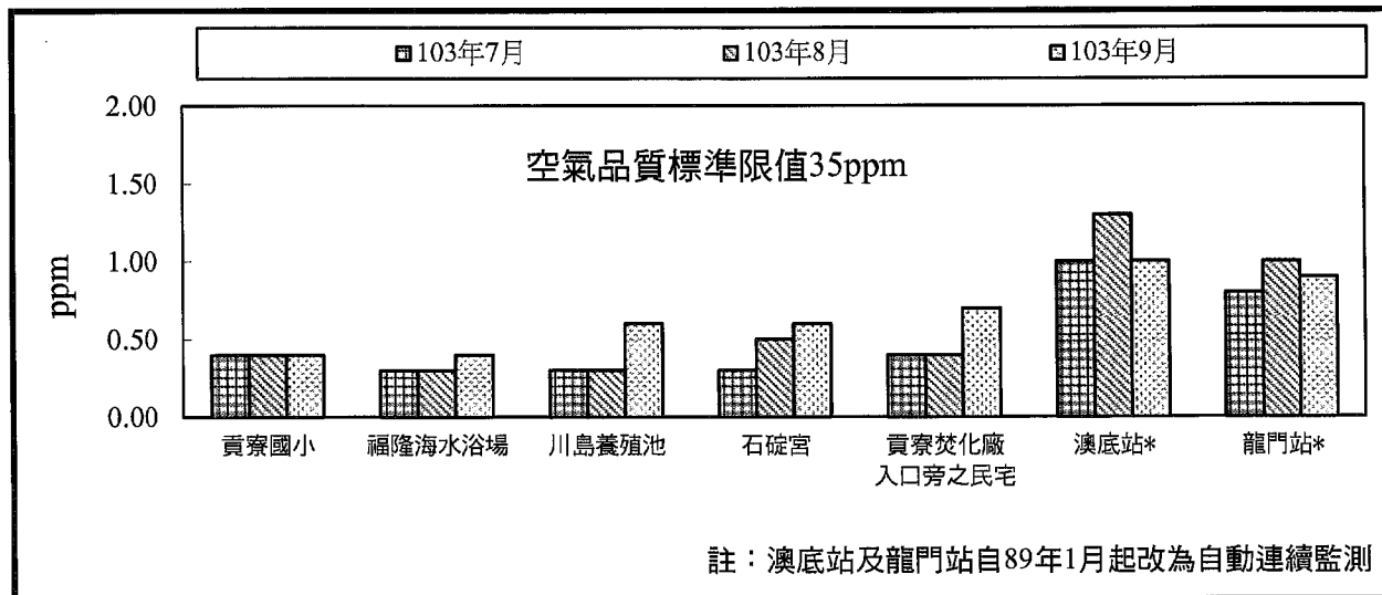
圖2.2-6 核四施工環境監測空氣品質一氧化碳103年7~9月小時平均值(最大值)比較分析圖
