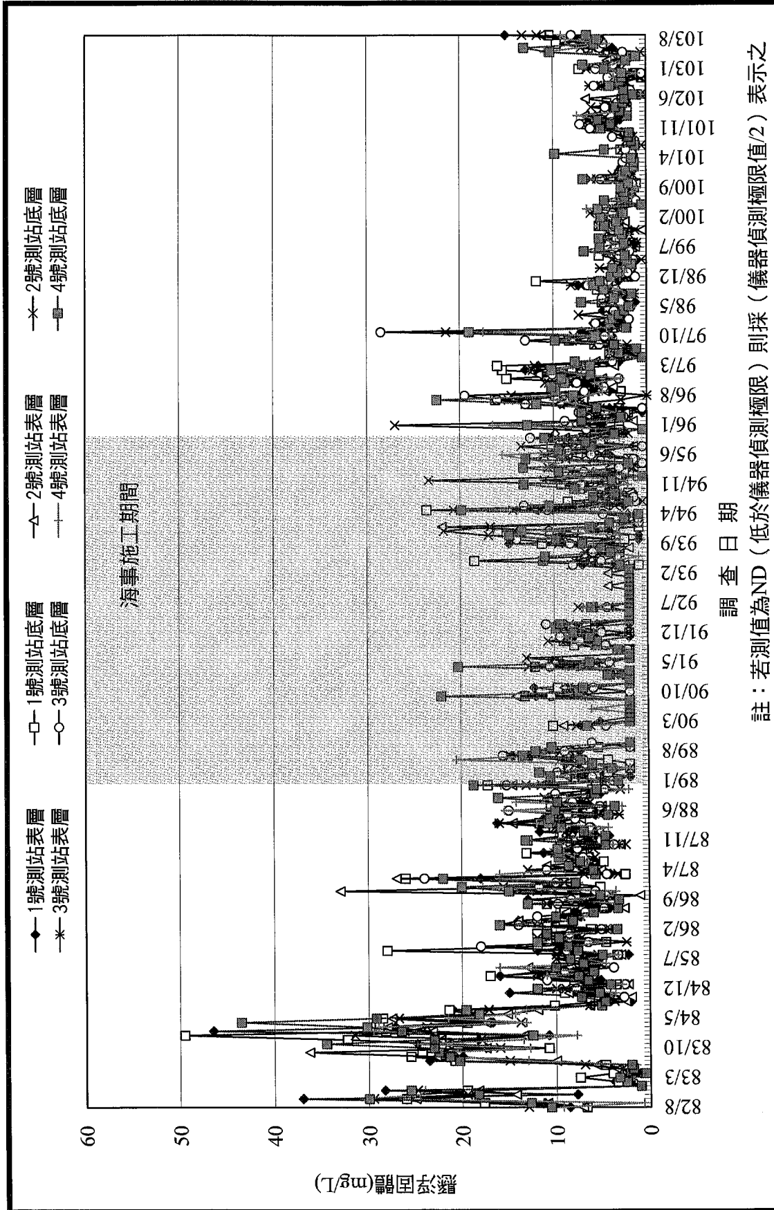
圖3.1-27 核四施工環境監測海域水質懸浮固體濃度變化圖
