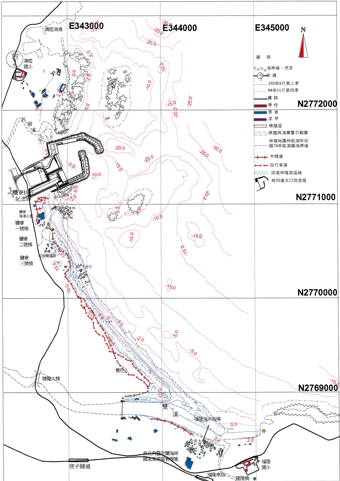
圖 3.1-50 核四施工期間環境監測海岸地形 103 年 8 月與 94 年 11 月監測結果比較（海事工程完工後）
