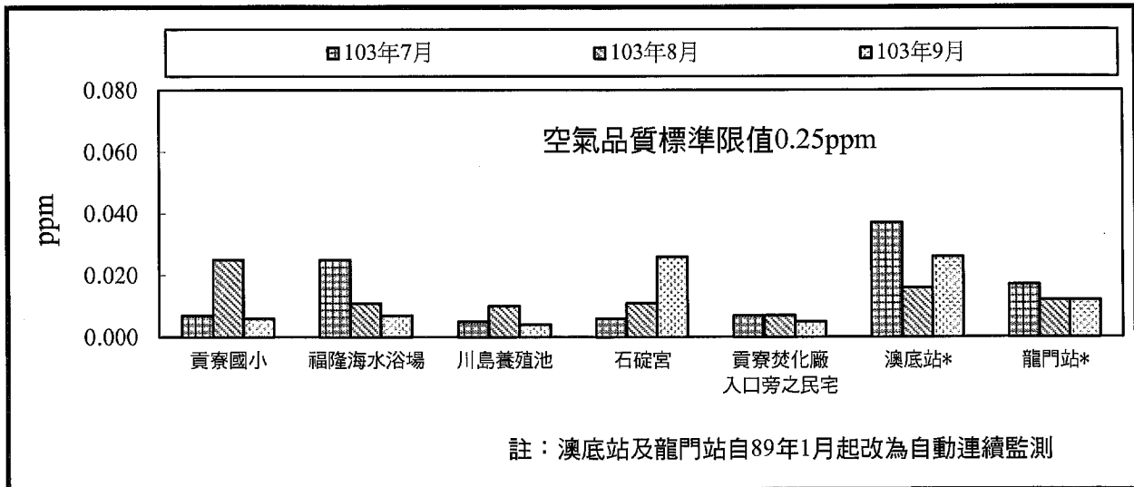
圖2.2-5 核四施工環境監測空氣品質二氧化氮103年7~9月小時平均值(最大值)比較分析圖
