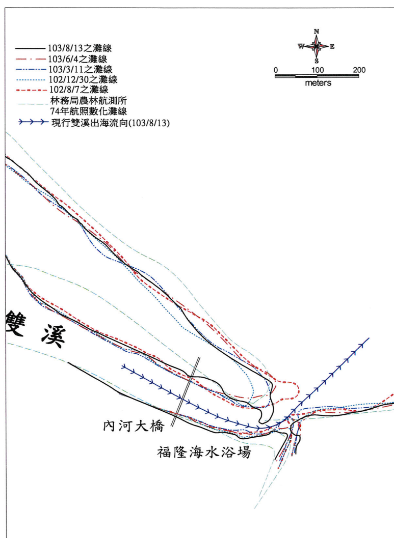
福隆海水浴場附近灘線變化及出海流向比較圖
