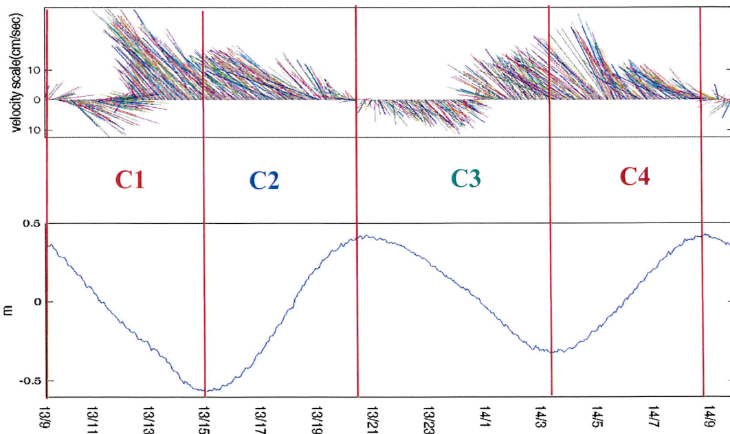
圖2.15-5 核四施工期間環境監測103年第3季近岸流場調查 累積向量路徑圖
