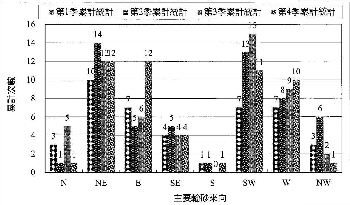
圖 3.1-43 歷年主要輸砂來向分季累計次數比較圖
