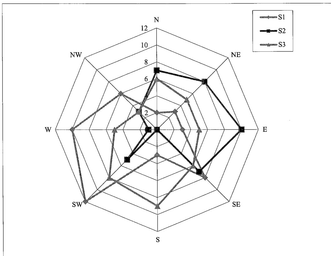
圖 3.1-42 各測站最大淨輸砂方向歷年累計次數雷達圖
