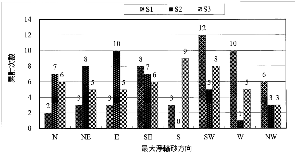
圖 3.1-41 各測站最大淨輸砂方向歷年累計次數比較圖
