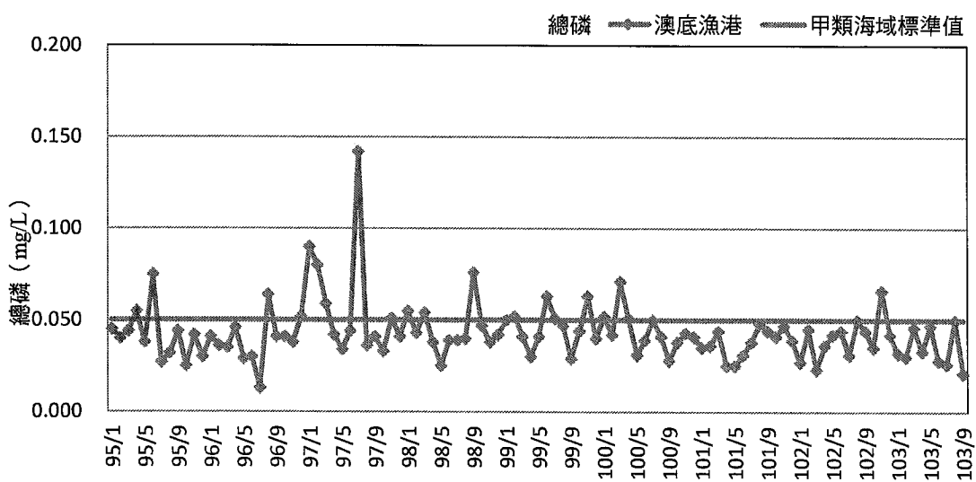
圖3.1-32 核四施工環境監測澳底漁港水質歷年調查變化圖
