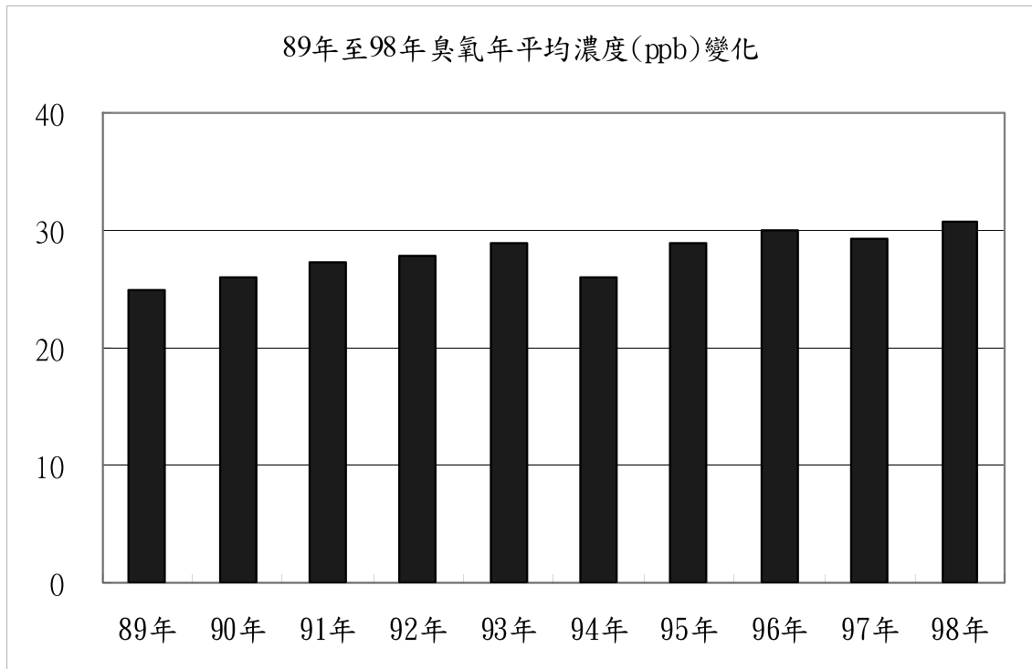
圖3-2-5 89年至98年臭氧年平均濃度變化圖
