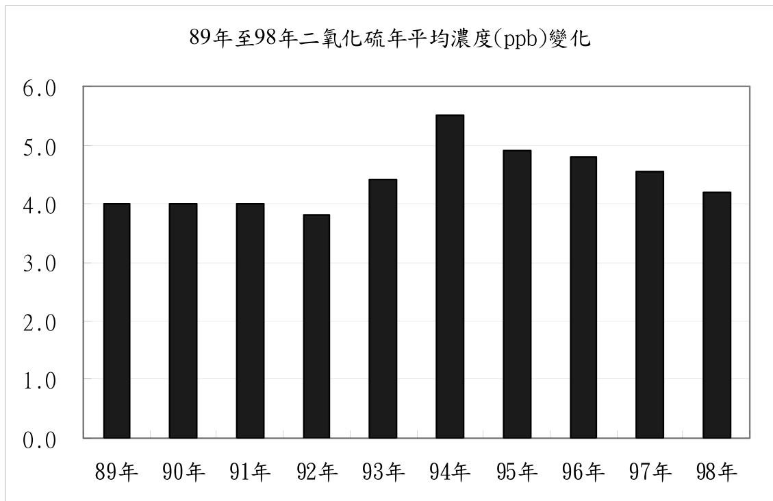
圖3-2-2 89年至98年二氧化硫年平均濃度變化圖
