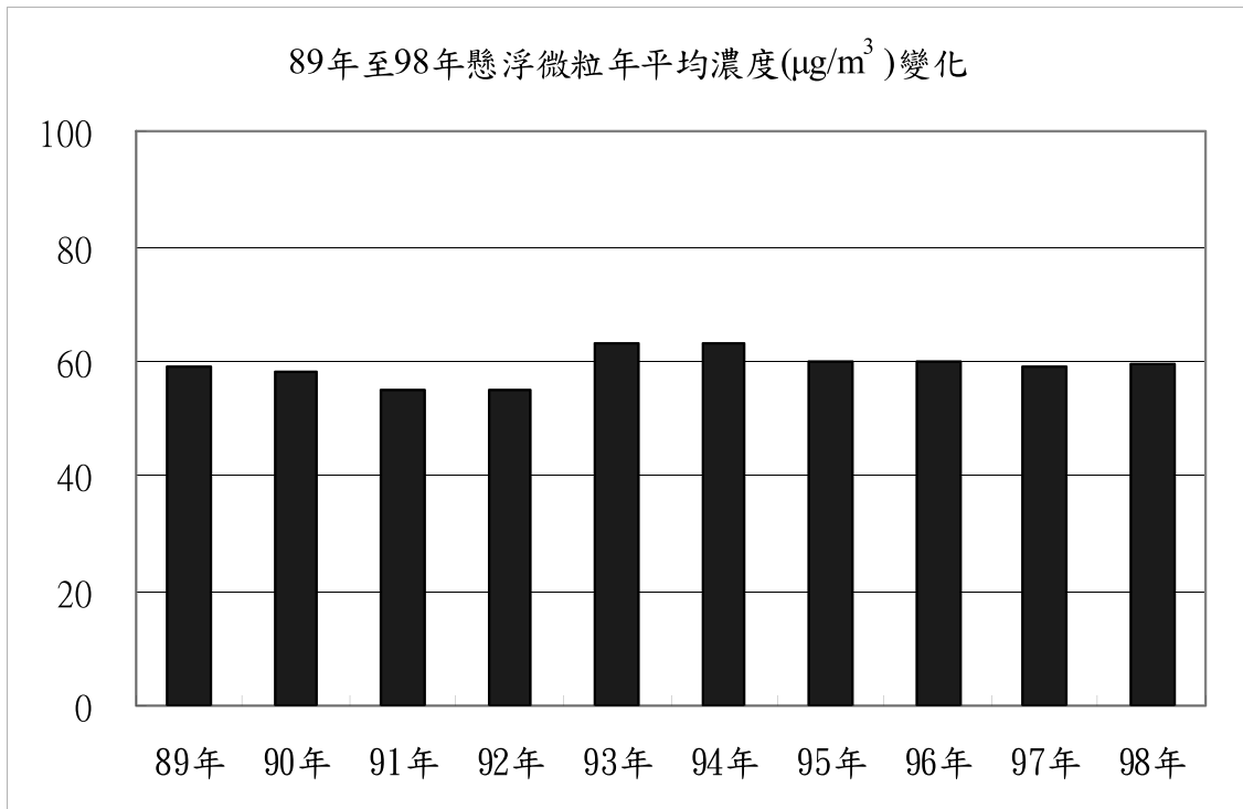
圖3-2-1 89年至98年懸浮微粒年平均濃度變化圖
