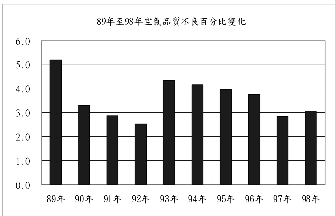
圖3-1-2 89年至98年空氣品質不良百分比變化圖
