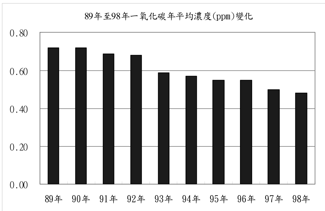
圖3-2-4 89年至98年一氧化碳年平均濃度變化圖
