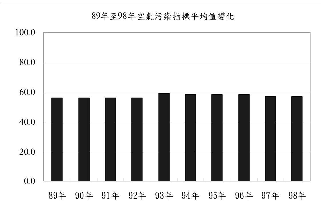
圖3-1-1 89年至98年空氣污染指標平均值變化圖
