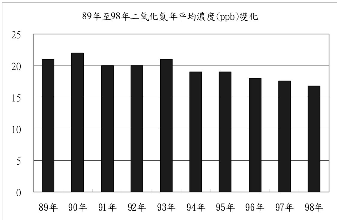
圖3-2-3 89年至98年二氧化氮年平均濃度變化圖
