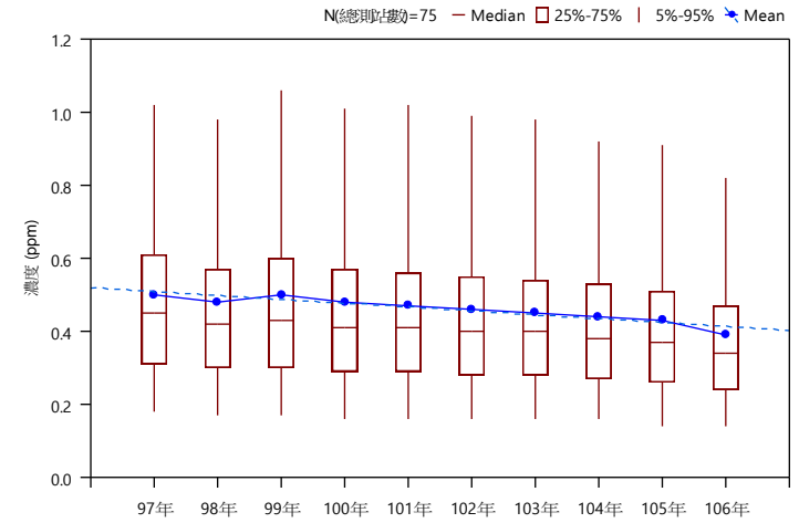
歷年一氧化碳(CO)濃度趨勢圖
