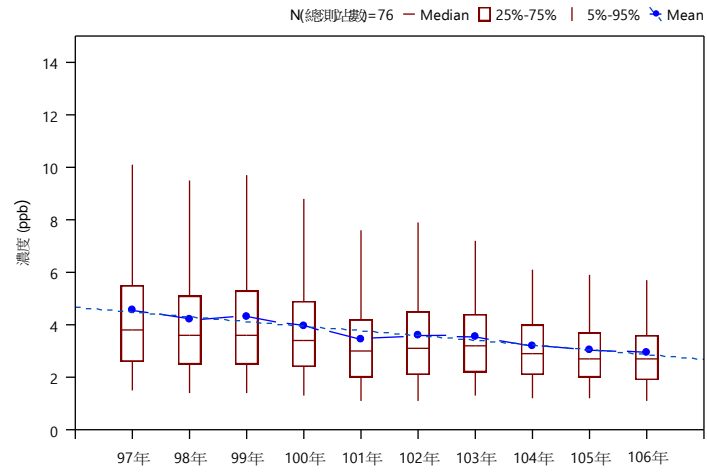
歷年二氧化硫(SO 2 )濃度趨勢圖
