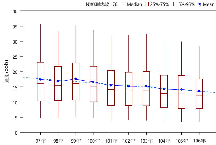
歷年二氧化氮(NO 2 )濃度趨勢圖
