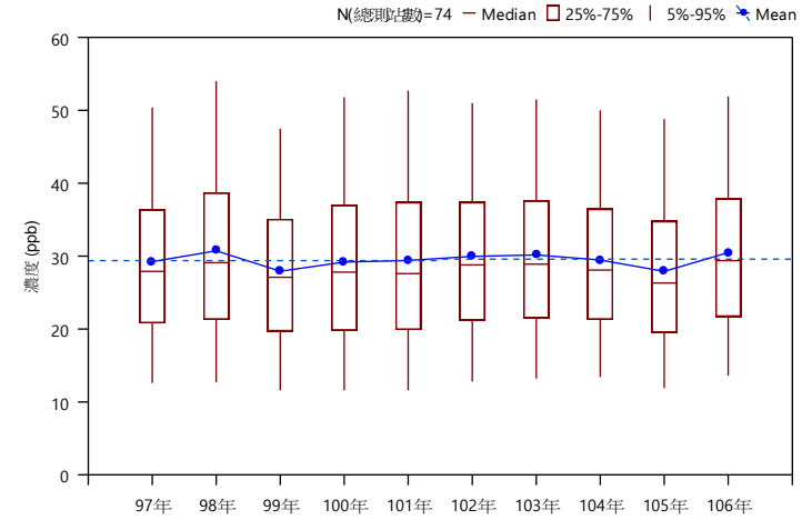
歷年臭氧(O 3,avg )濃度趨勢圖
