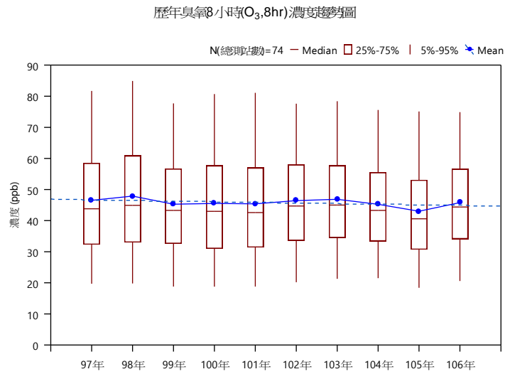
圖 3-13 (A)懸浮微粒 (B)細懸浮微粒(自動) (C)細懸浮微粒(手動站) (D)細懸浮微粒(手動站-扣除陽明、三義及恆春測站) (E)二氧化硫 (F)二氧化氮 (G)一氧化碳 (H)臭氧 (I)臭氧 8 小時 歷年濃度趨勢圖
