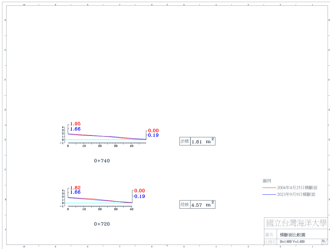
圖 4-4(a) 2023 年 9 月 9 日 A 監測區橫斷面比較圖
