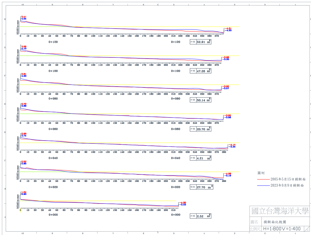
圖 4-5(f) 2023 年 9 月 9 日 B 監測區橫斷面比較圖
