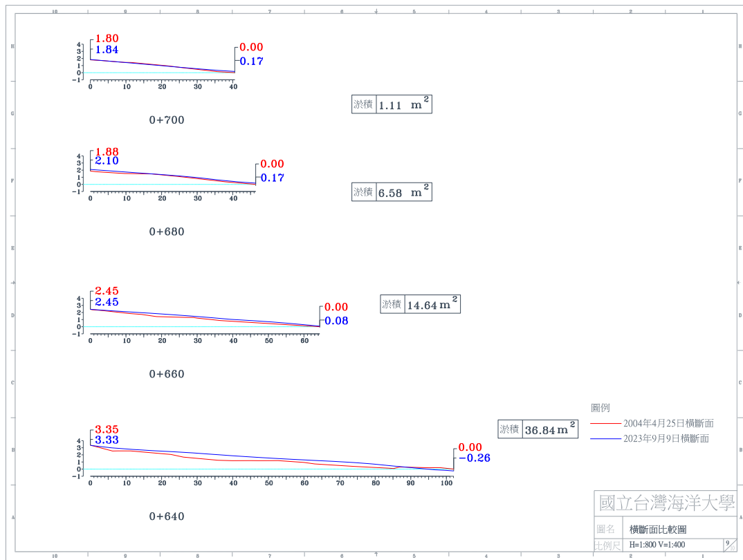
圖 4-4(b) 2023 年 9 月 9 日 A 監測區橫斷面比較圖
