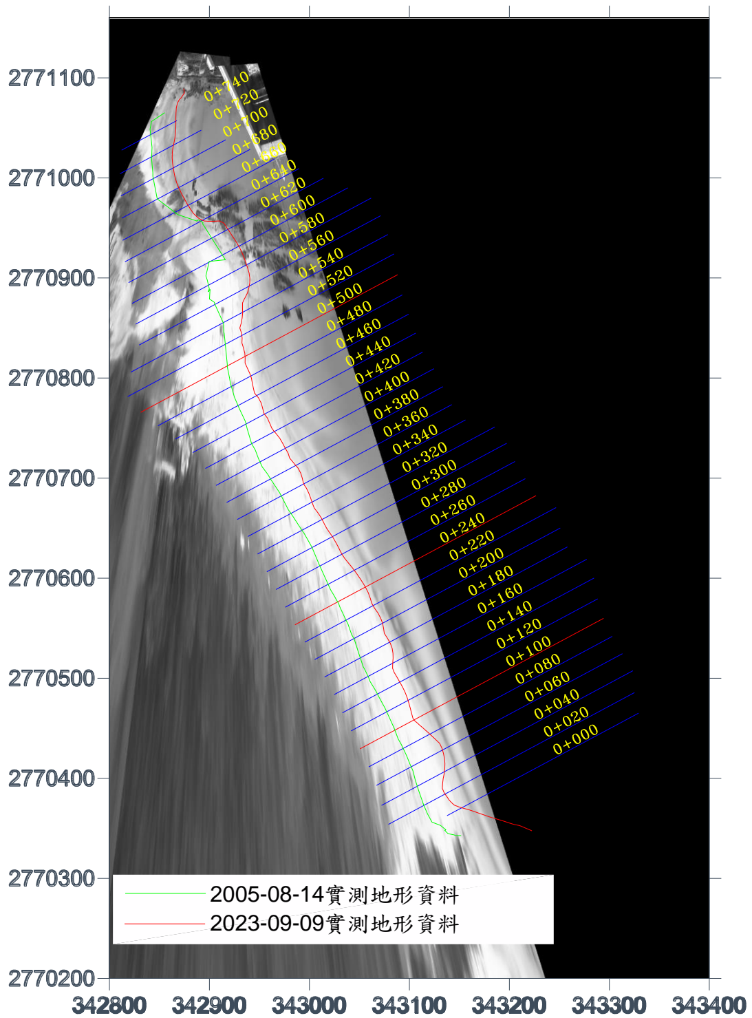
圖 4-19 長期實測 0 m 灘線比對平面示意圖(2023/09/09)
