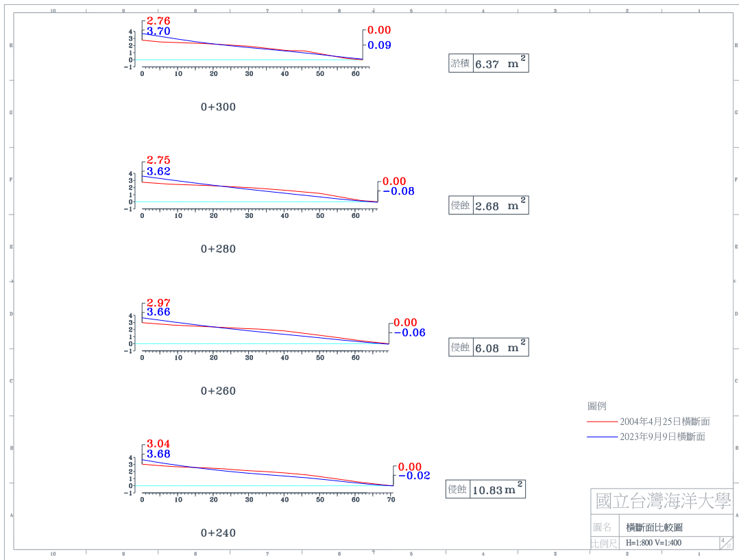
圖 4-4(g) 2023 年 9 月 9 日 A 監測區橫斷面比較圖
