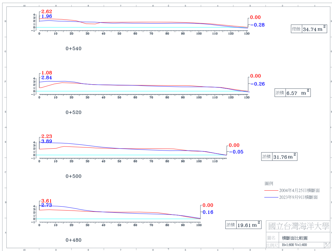
圖 4-4(d) 2023 年 9 月 9 日 A 監測區橫斷面比較圖
