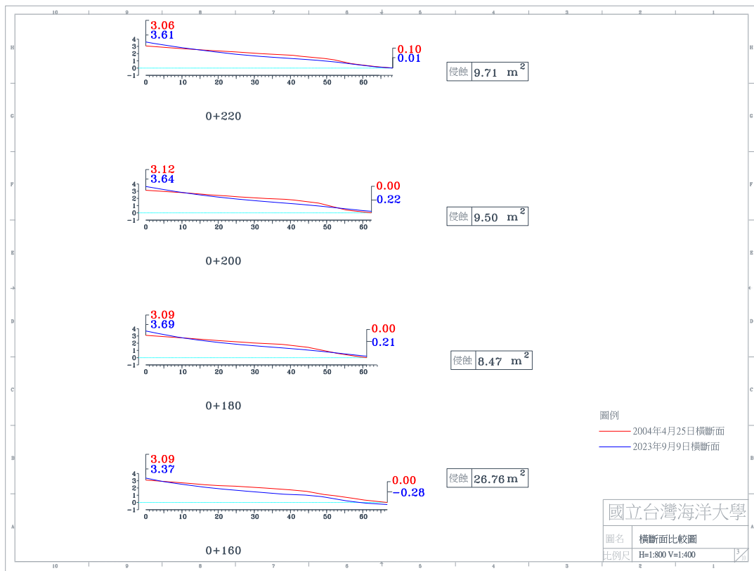
圖 4-4(h) 2023 年 9 月 9 日 A 監測區橫斷面比較圖
