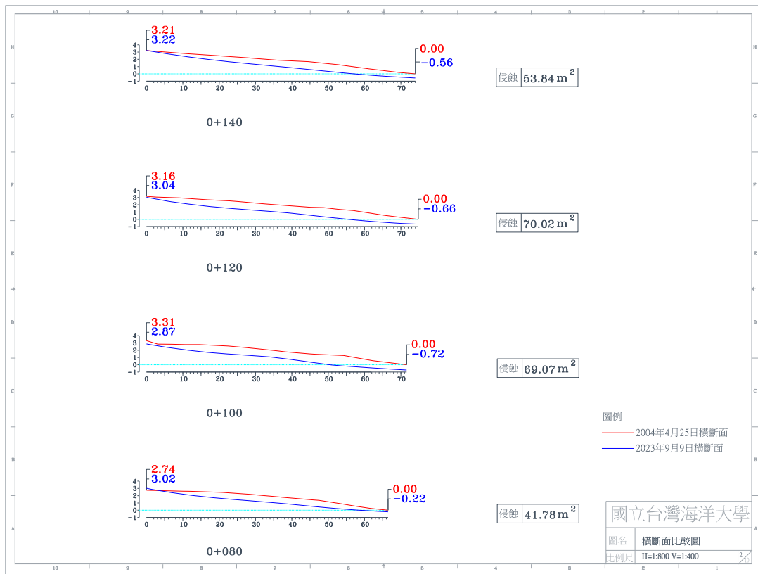
圖 4-4(i) 2023 年 9 月 9 日 A 監測區橫斷面比較圖
