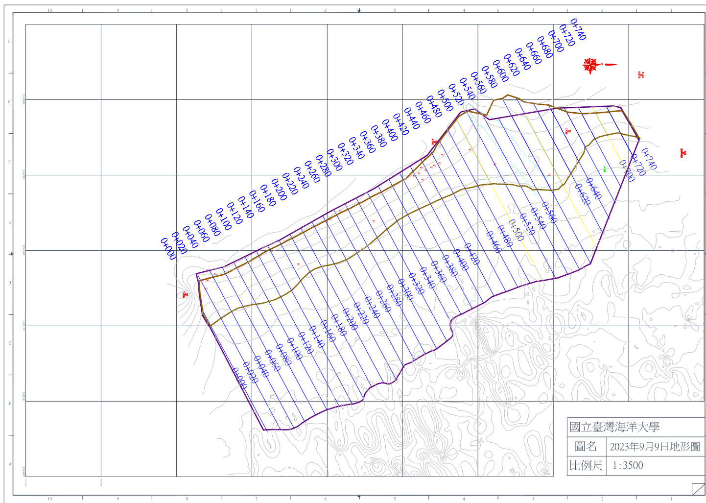
圖 4-1 2023 年 9 月 9 日監測地形
