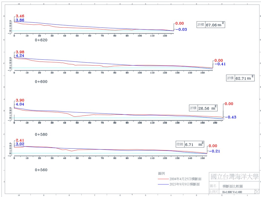
圖 4-4(c) 2023 年 9 月 9 日 A 監測區橫斷面比較圖
