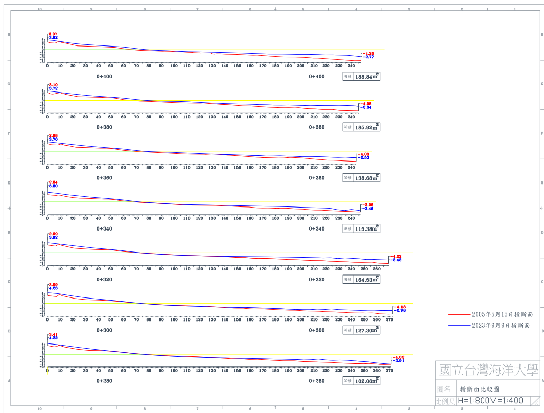
圖 4-5(d) 2023 年 9 月 9 日 B 監測區橫斷面比較圖
