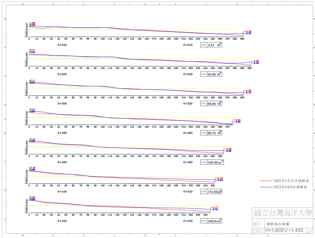
圖 4-5(c) 2023 年 9 月 9 日 B 監測區橫斷面比較圖
