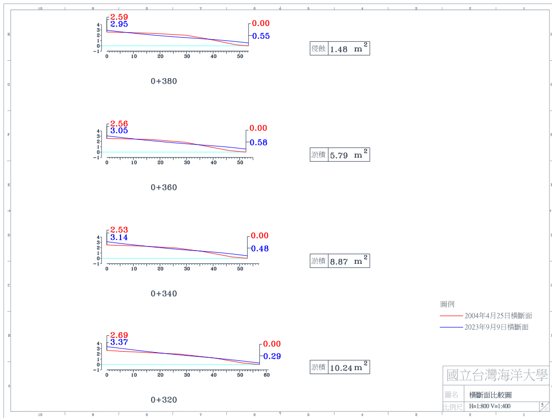
圖 4-4(f) 2023 年 9 月 9 日 A 監測區橫斷面比較圖
