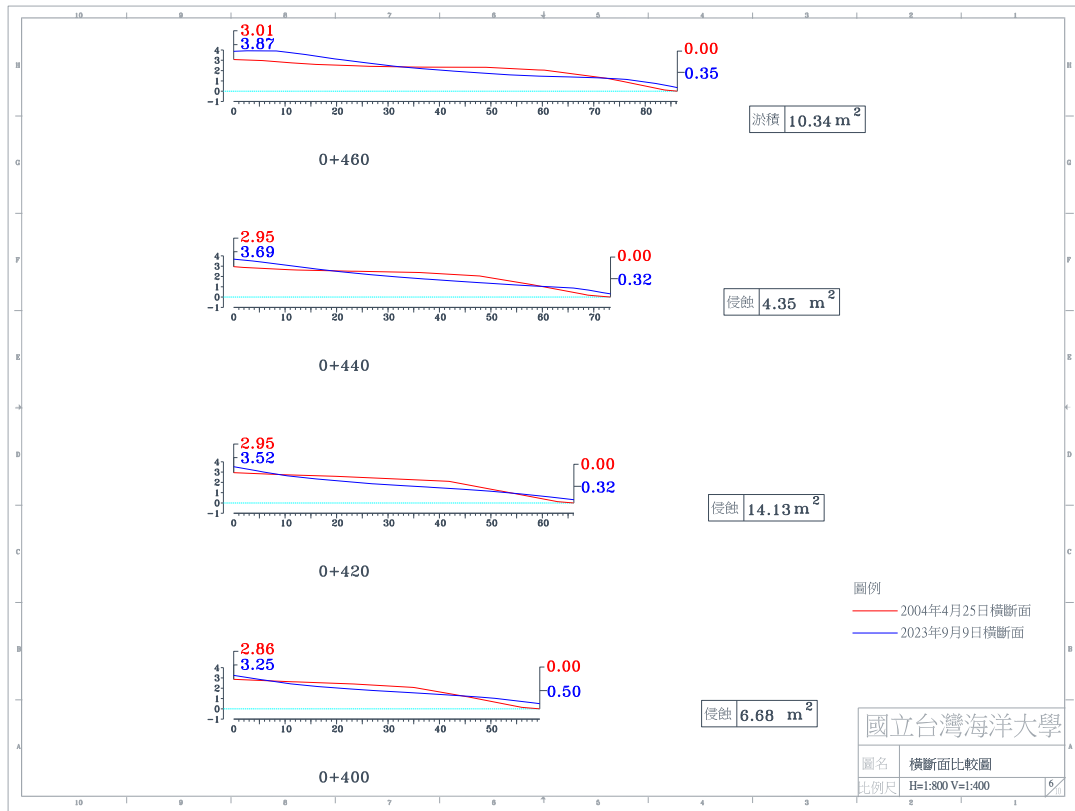
圖 4-4(e) 2023 年 9 月 9 日 A 監測區橫斷面比較圖
