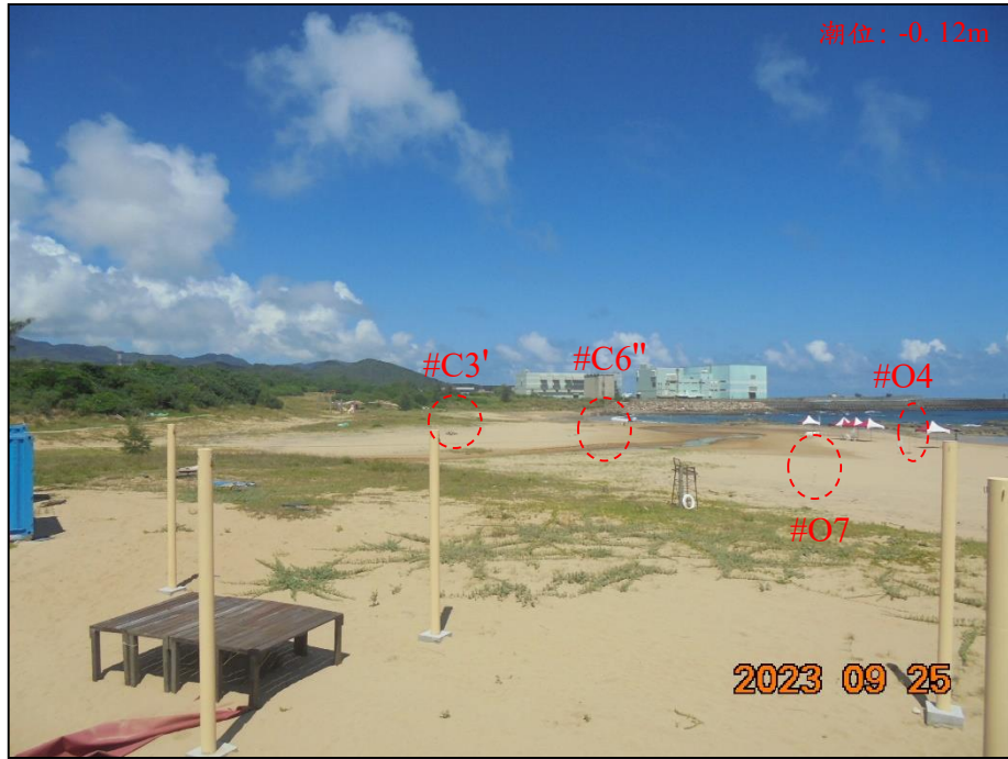
圖 3-10 小舞台前輔助觀測樁位置圖 (2023/09/25)
