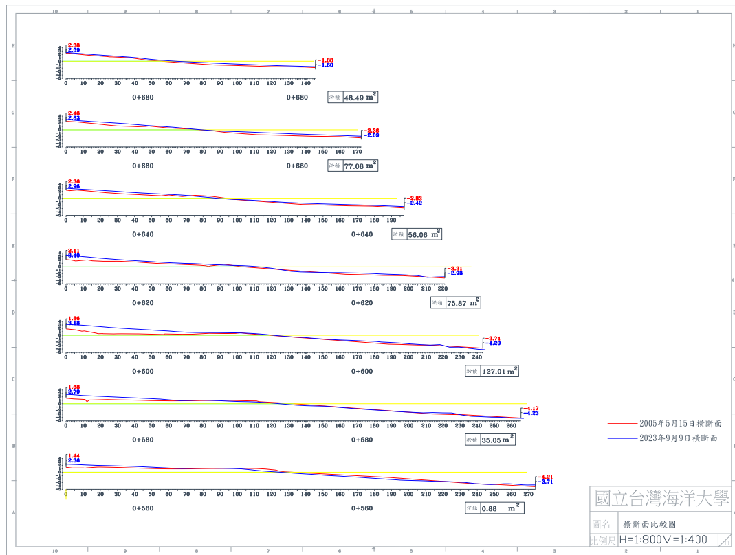
圖 4-5(b) 2023 年 9 月 9 日 B 監測區橫斷面比較圖
