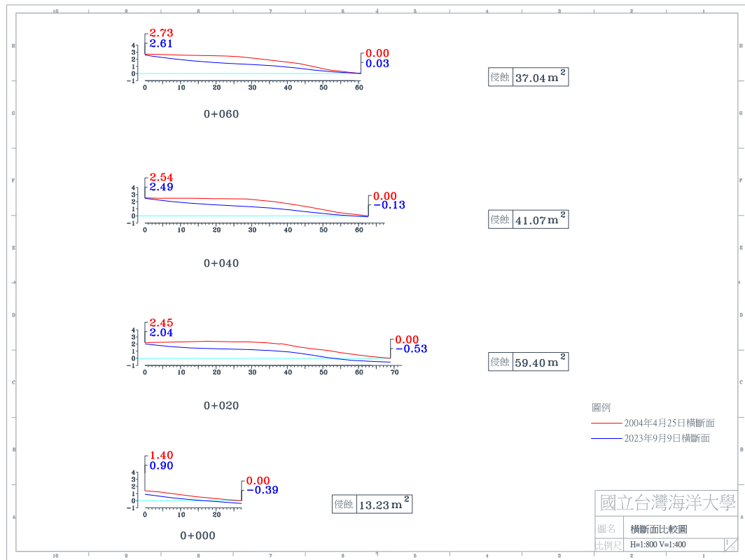
圖 4-4(j) 2023 年 9 月 9 日 A 監測區橫斷面比較圖
