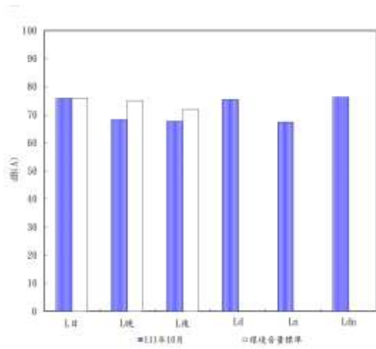
圖 2.2-75 5 號連絡道路口本季噪音調查結果分析圖
