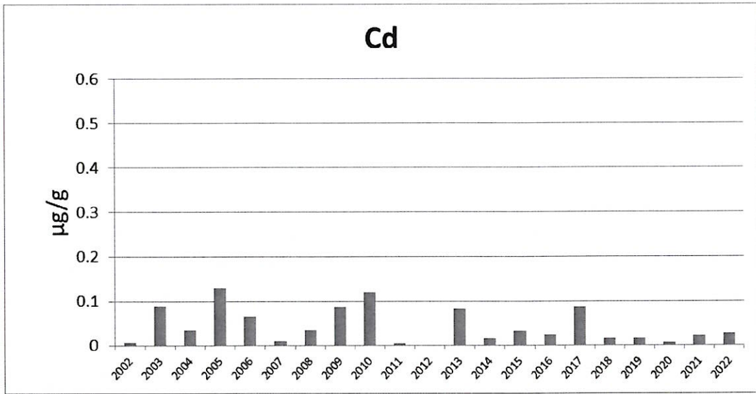
附錄 III.10-2 圖 7. 2002 至 2022 年 11 月短指和尚蟹體內鎘含量之年度比較圖
