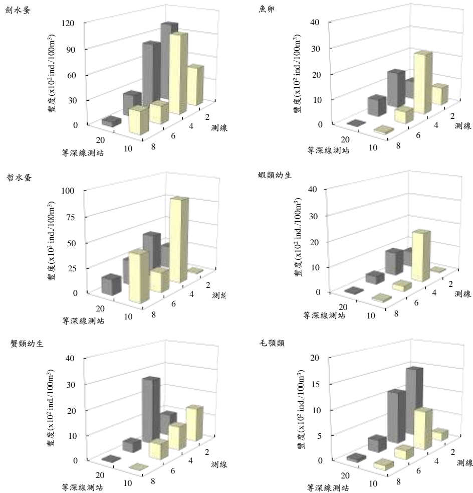
圖 2.10.2-2 民國 111 年 10 月彰化濱海工業區附近海域浮游動物主要優勢類群之豐度分布圖
