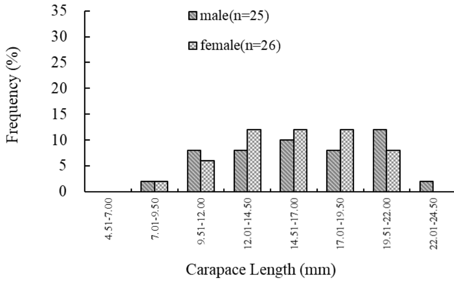
圖 III.6-16 本季雌雄螻蛄蝦體型頻度分布圖
