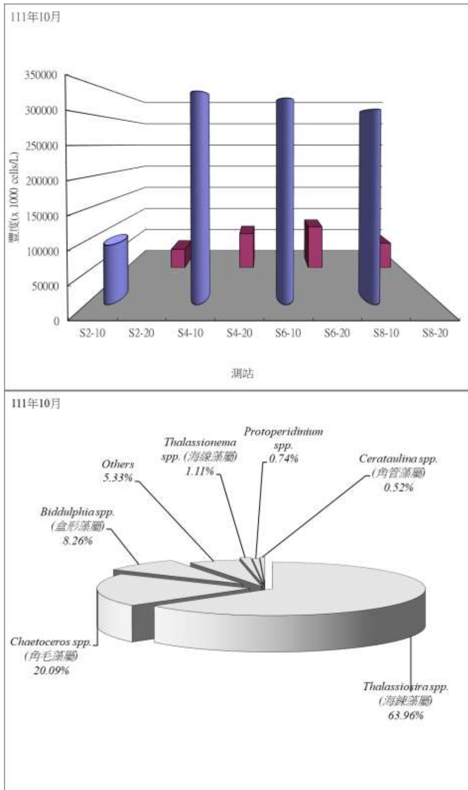
圖 2.10.1-1 民國 111 年 10 月於彰化濱海工業區附近海域各測站之浮游植物豐度分析圖
