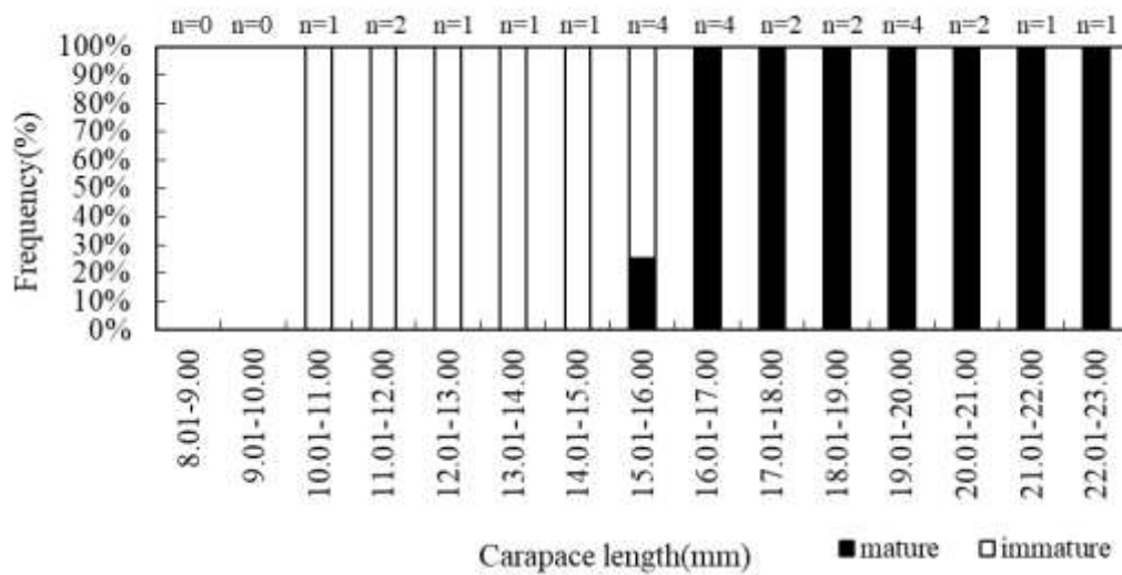
圖 III.6-19 本季成熟雌蝦與未成熟雌螻之比例
