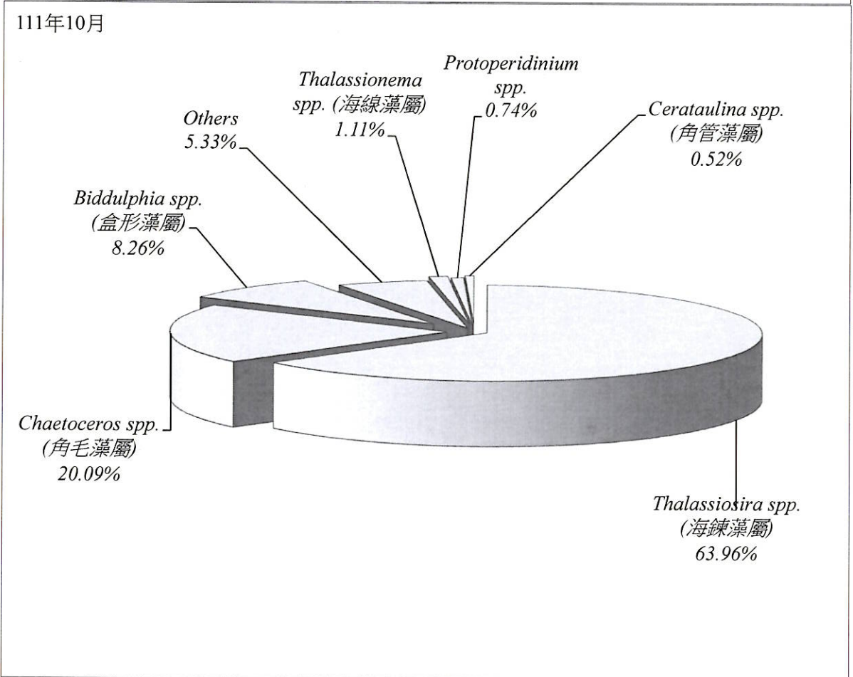
圖2.10.1-1 民國111年10月於彰化濱海工業區附近海域各測站之浮游植物豐度分析圖
