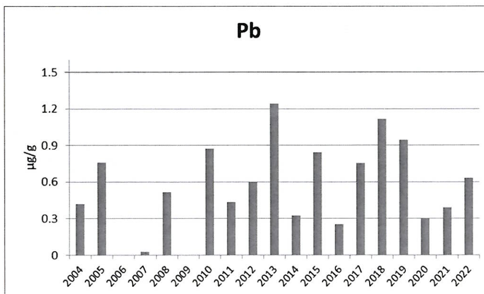
附錄 III.10-2 圖 10. 2004 至 2022 年 11 月漁舟蜆螺體內鉛含量之年度比較圖
