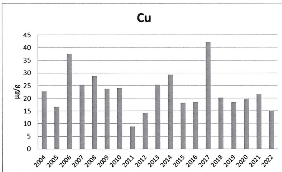
附錄 III.10-2 圖 9. 2004 至 2022 年 11 月漁舟蜆螺體內銅含量之年度比較圖
