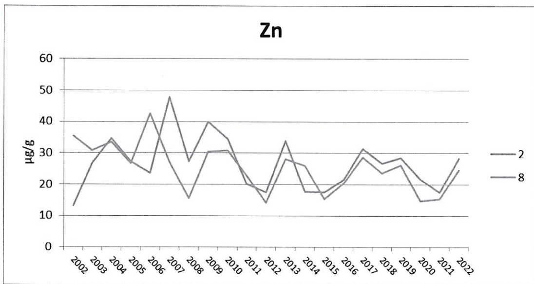
附錄 III.10-2 圖 16. 2002~2022 年 11 月測站 2 及 8 短指和尚蟹體內鋅含量之測站比較圖
