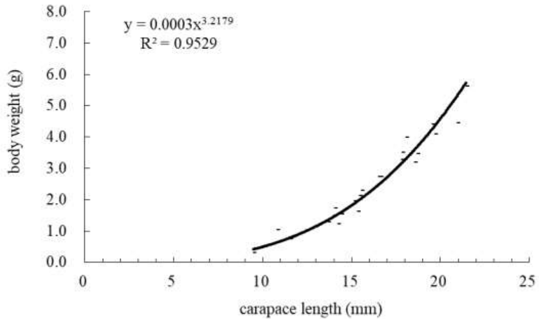
圖 III.6-13 本季螞蛄蝦雌蝦頭胸甲長(cl)與體重(bw 濕重)之關係
