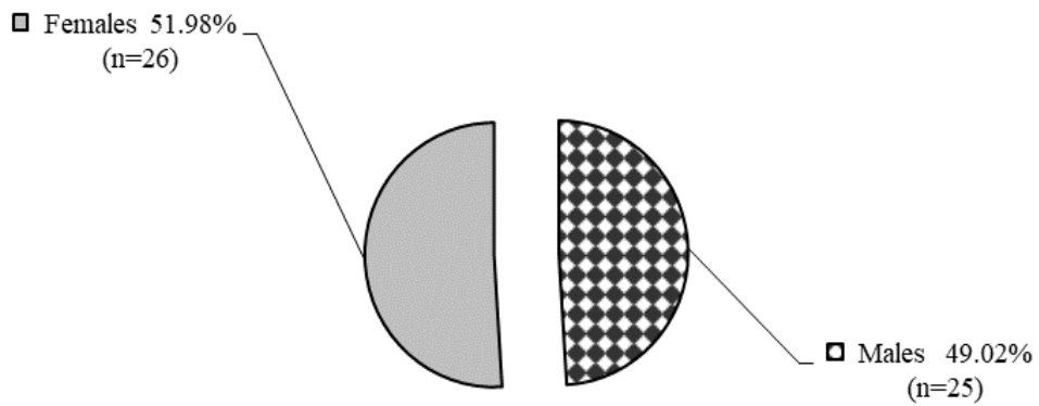
圖 III.6-17 本季伸港地區雌、雄螻蛄蝦之比例(n=51)
