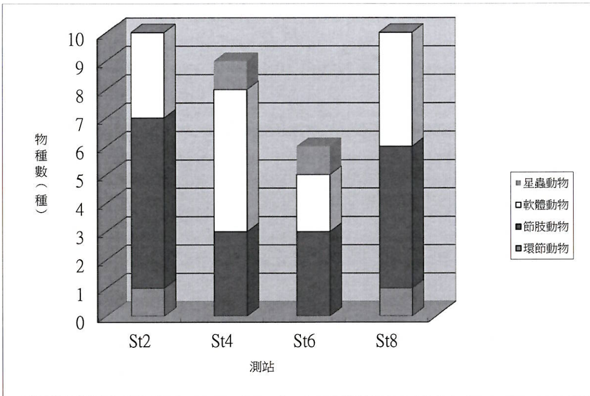
附錄III.10-1圖7 民國111年10月於彰濱工業區附近海域潮間帶各測站各大類生物之物種數比較圖
