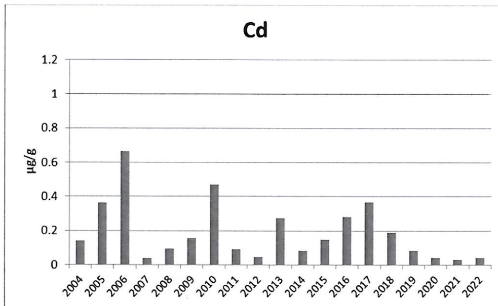
附錄 III.10-2 圖 11. 2004 至 2022 年 11 月漁舟蜆螺體內鎘含量之年度比較圖
