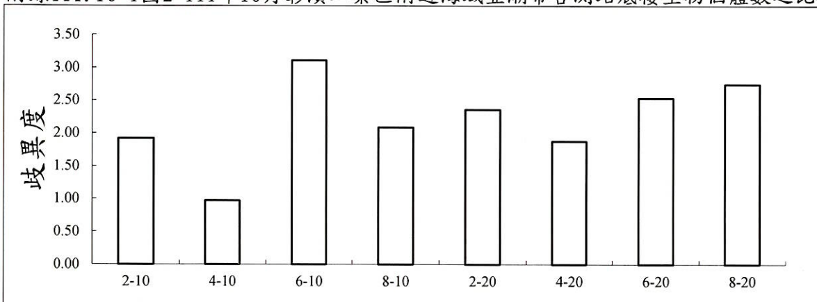
附錄III. 10-1圖3 111年10月彰濱工業區附近海域亞潮帶各測站底棲生物歧異度之比較
