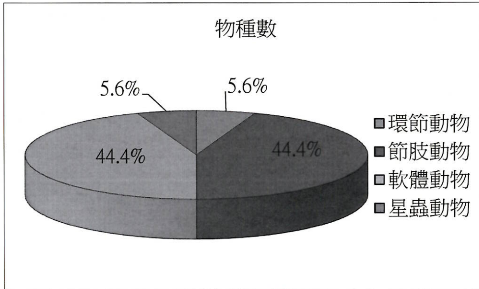
附錄III.10-1圖5 民國111年10月潮間帶各大類生物之物種數百分比
