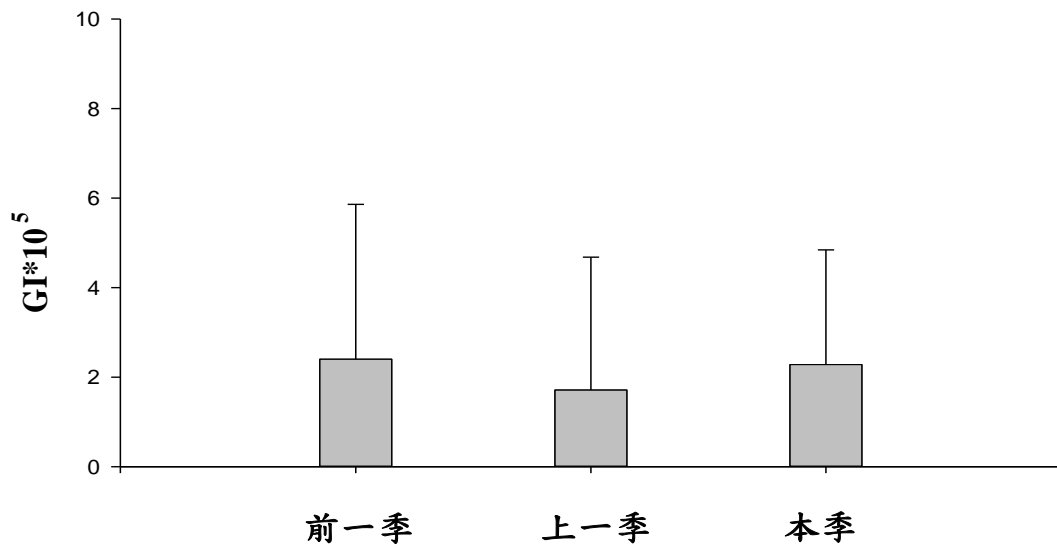
圖 III.6-18 本季與前兩季螻蛄蝦卵巢指數之比較
