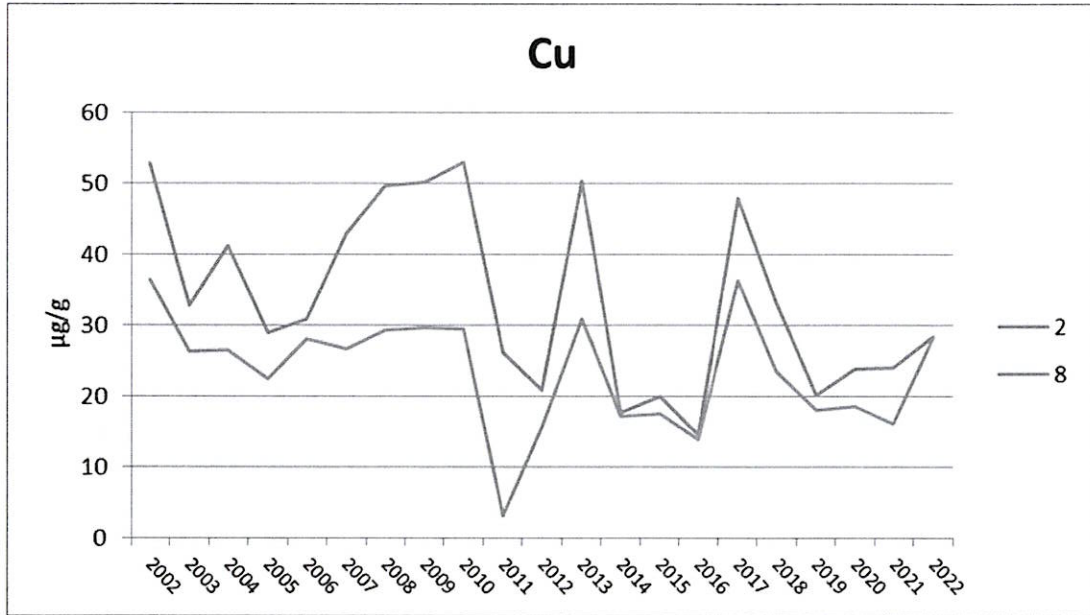
附錄 III.10-2 圖 13. 2002~2022 年 11 月測站 2 及 8 短指和尚蟹體內銅含量之測站比較圖
