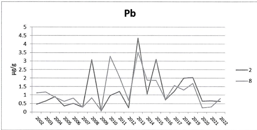
附錄 III.10-2 圖 14. 2002~2022 年 11 月測站 2 及 8 短指和尚蟹體內鉛含量之測站比較圖
