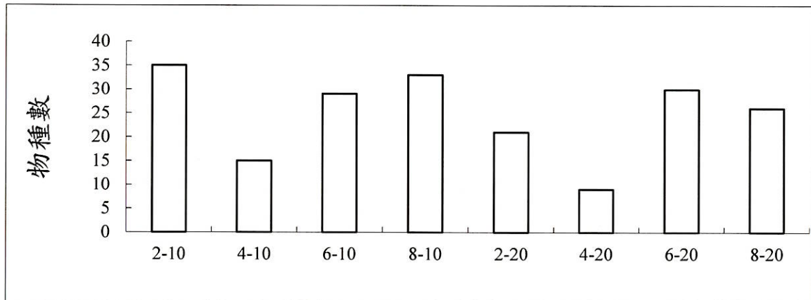
附錄III. 10-1圖1 111年10月彰濱工業區附近海域亞潮帶各測站底棲生物物種數之比較
