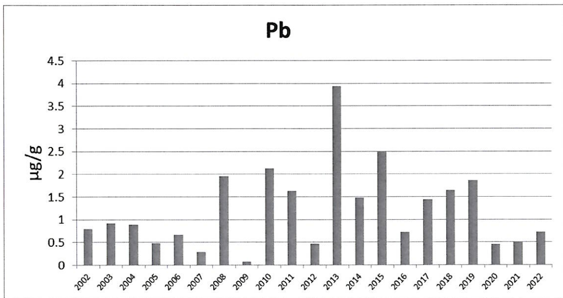
附錄 III.10-2 圖 6. 2002 至 2022 年 11 月短指和尚蟹體內鉛含量之年度比較圖
