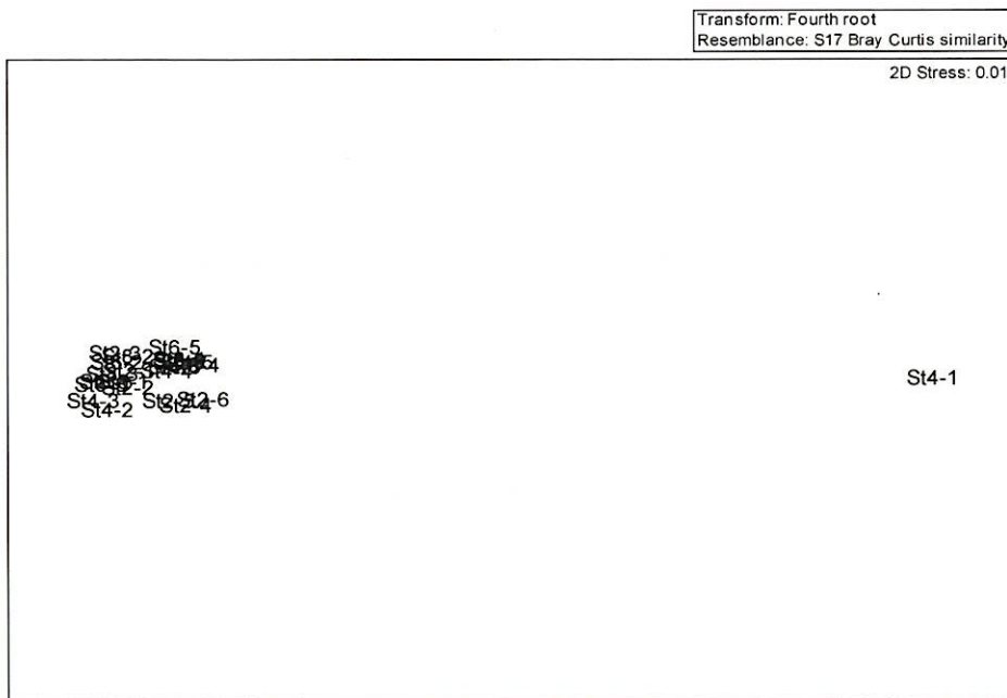
附錄III.10-2圖4 民國111年10月於彰濱工業區附近海域潮間帶各測站之群聚MDS圖。
