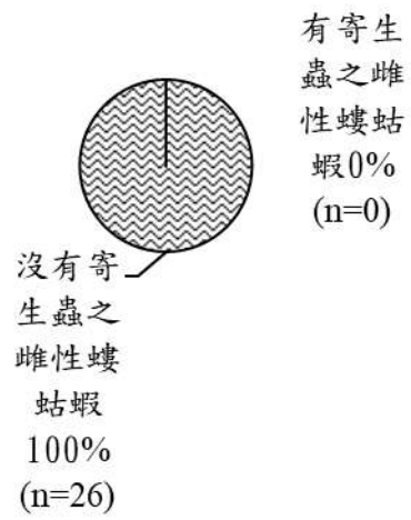
圖III.6-25 本季雌性螻蛄蝦被等足目寄生的百分率(n=26)。
