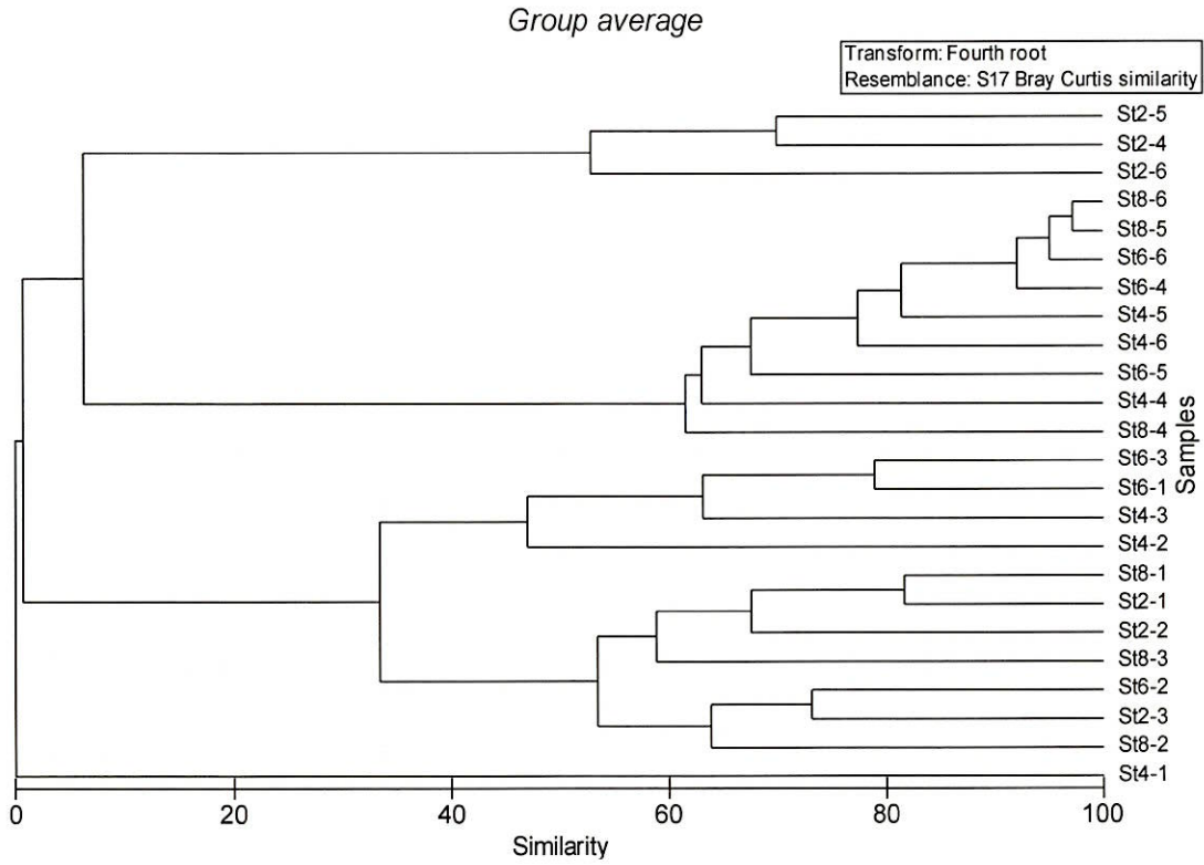
附錄III.10-2圖3 民國111年10月於彰濱工業區附近海域潮間帶各測站之群聚分析樹狀圖。
