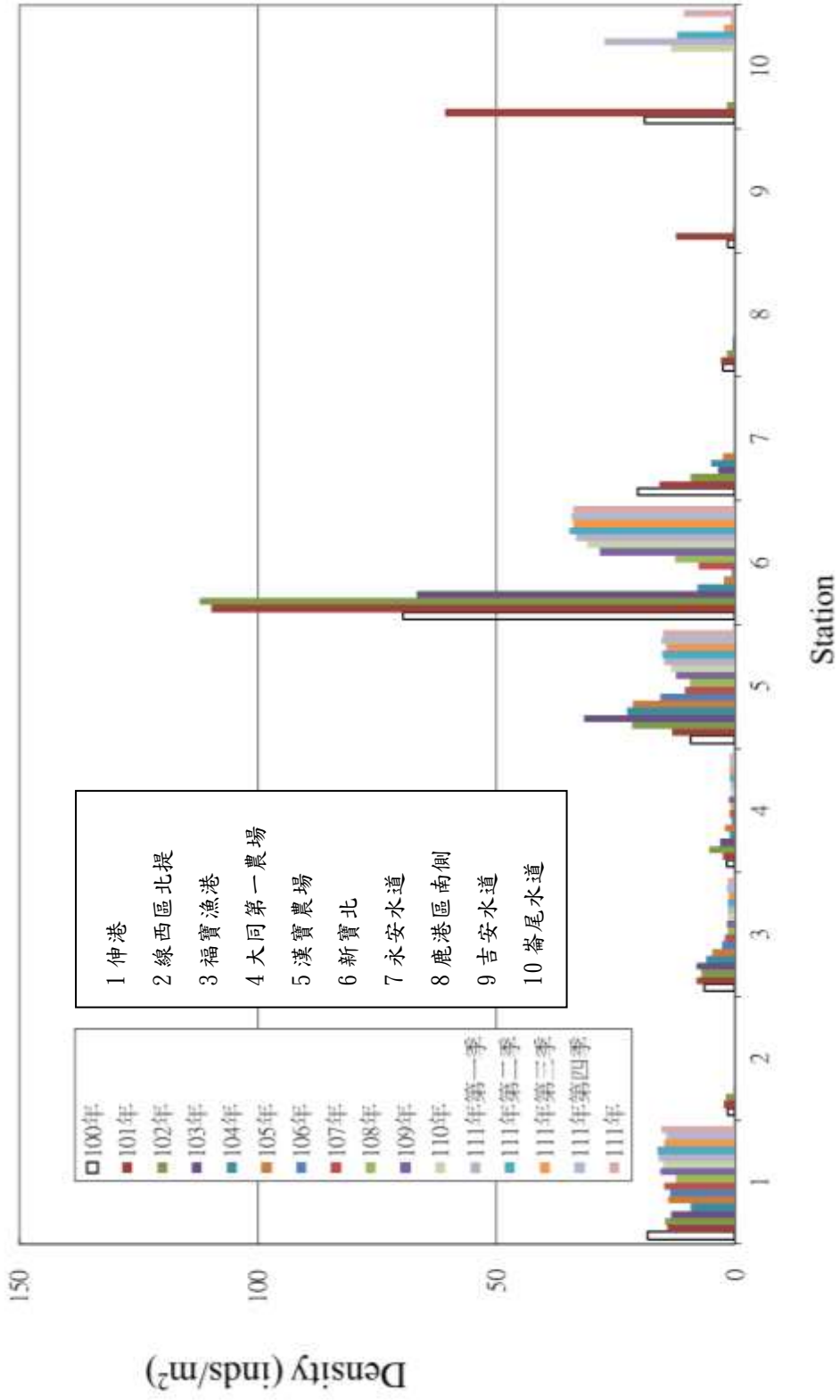
圖 3.1.6-1 各測站蜉蝣平均密度(個體數/m 2 )分布圖
