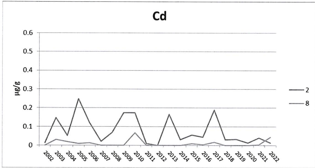
附錄 III.10-2 圖 15. 2002~2022 年 11 月測站 2 及 8 短指和尚蟹體內鎘含量之測站比較圖
