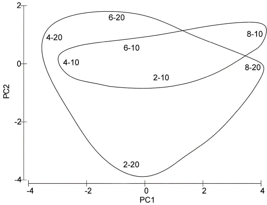
圖 2.10.2-3 民國 111 年 10 月彰濱工業區附近海域各測站浮游動物群聚分析圖 (圖中第一個數字代表測站，第二個數字代表深度)
