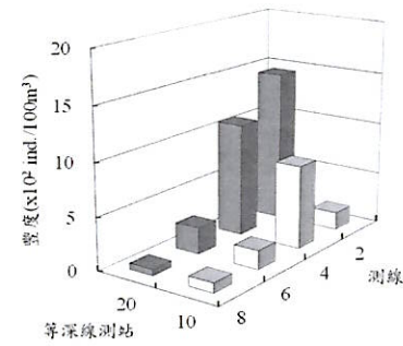
圖 2.10.2-2 民國 111 年 10 月彰化濱海工業區附近海域浮游動物主要優勢類群之豐度分布圖
