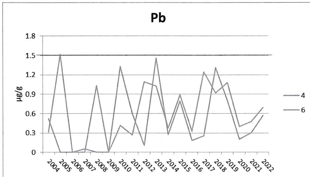
附錄 III.10-2 圖 18. 2004~2022 年 11 月測站 4 及 6 漁舟蜆螺體內鉛含量之測站比較圖
