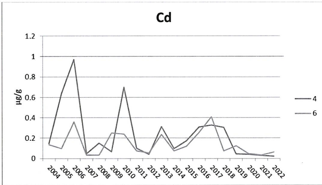
附錄 III.10-2 圖 19. 2004~2022 年 11 月測站 4 及 6 漁舟蜆螺體內鎘含量之測站比較圖
