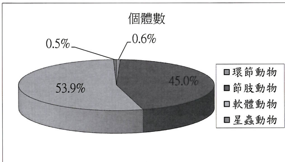
附錄III.10-1圖6 民國111年10月潮間帶各大類生物之個體數百分比
