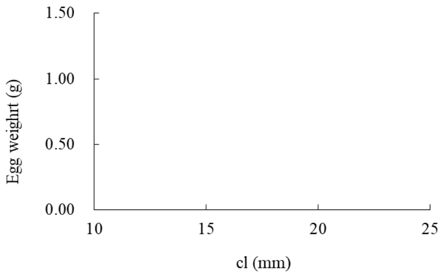
圖 III.6-23 本季螻蛄蝦抱卵母蝦(限未發眼卵)頭胸甲長(cl)與抱卵重(濕重)之關係(本季未發現抱卵螻蛄蝦)
