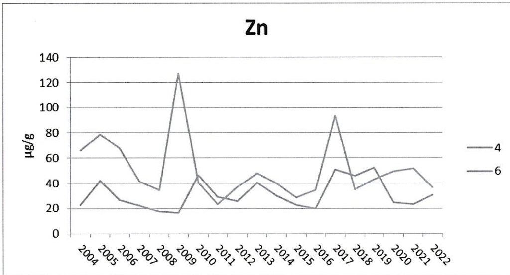
附錄 III.10-2 圖 20. 2004~2022 年 11 月測站 4 及 6 漁舟蜆螺體內鋅含量之測站比較圖
