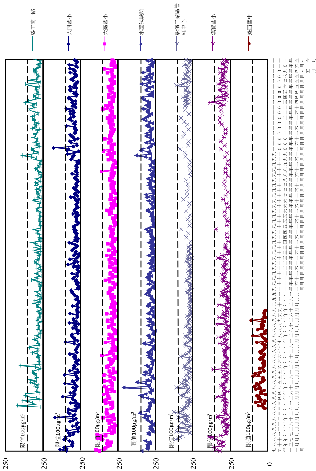
圖 3.1.1-7 彰濱地區歷年粒徑小於 10 \mu\text{m} 之懸浮微粒(PM 10 )日平均值監測結果分析圖
