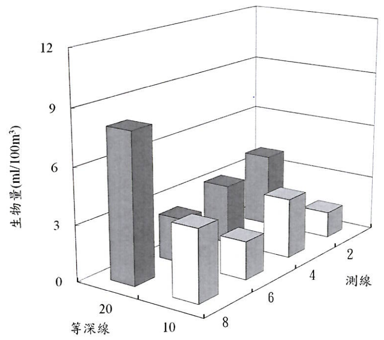
圖 2.10.2-1 民國 111 年 10 月彰化濱海工業區附近海域浮游動物之豐度及生物量分布圖
