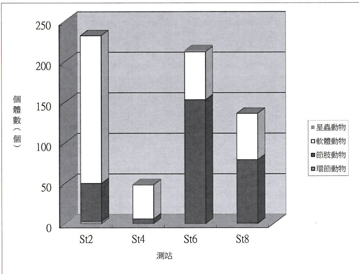
附錄III.10-1圖8 民國111年10月於彰濱工業區附近海域潮間帶各測站各大類生物之個體數比較圖
