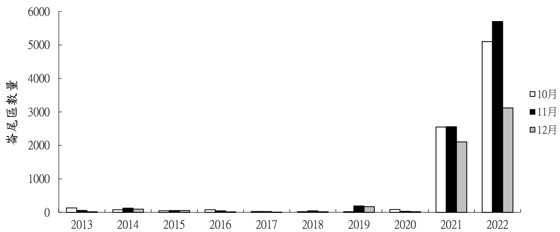
圖 3.1.5-4 崙尾西側海堤歷年同期鳥類調查結果比較
