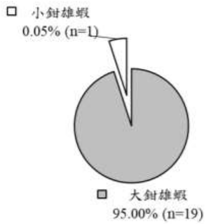
圖 III.6-14 本季螻蛄大小鉗雄蝦各佔之比例(n=20)
