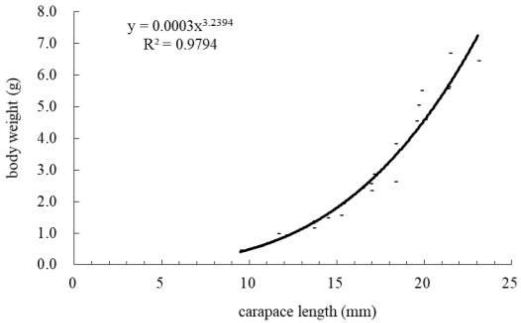
圖 III.6-12 本季螞蛄蝦雄蝦頭胸甲長(cl)與體重(bw 濕重)之關係
