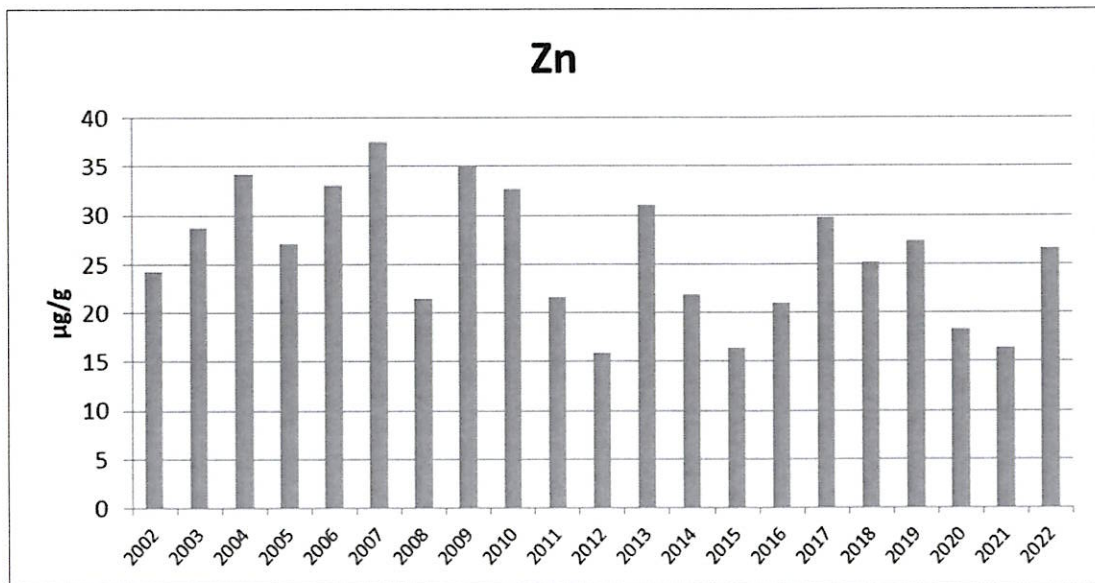
附錄 III.10-2 圖 8. 2002 至 2022 年 11 月短指和尚蟹體內鋅含量之年度比較圖
