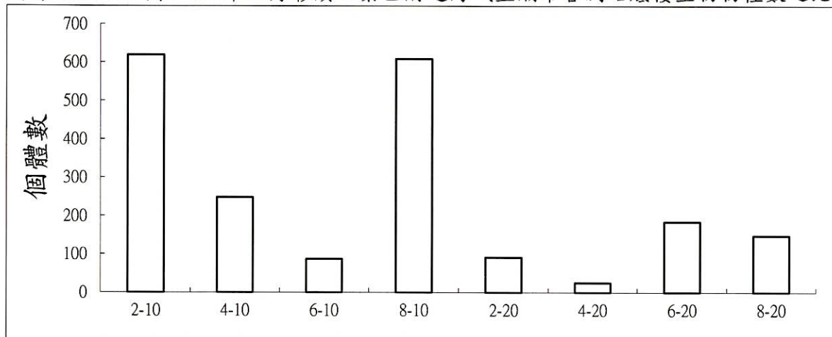
附錄III. 10-1圖2 111年10月彰濱工業區附近海域亞潮帶各測站底棲生物個體數之比較
