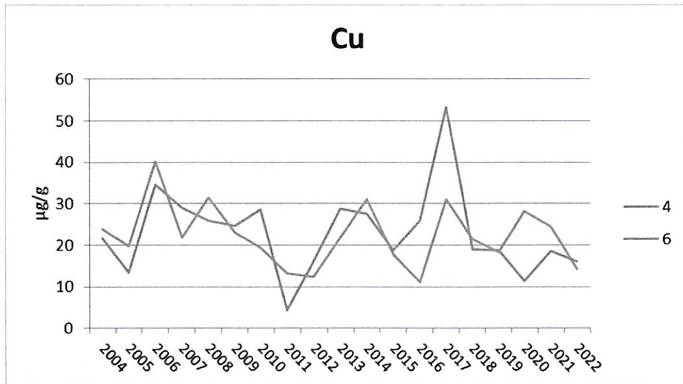
附錄 III.10-2 圖 17. 2004~2022 年 11 月測站 4 及 6 漁舟蜆螺體內銅含量之測站比較圖
