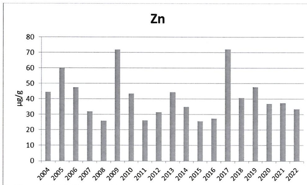
附錄 III.10-2 圖 12. 2004 至 2022 年 11 月漁舟蜆螺體內鋅含量之年度比較圖
