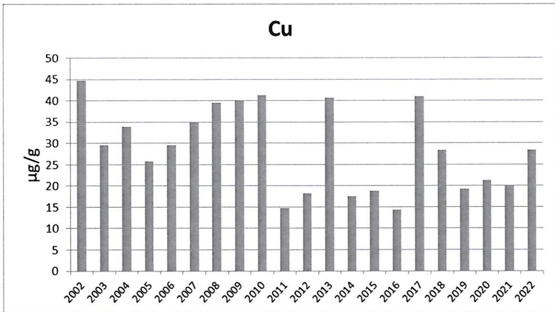
附錄 III.10-2 圖 5. 2002 至 2022 年 11 月短指和尚蟹體內銅含量之年度比較圖
