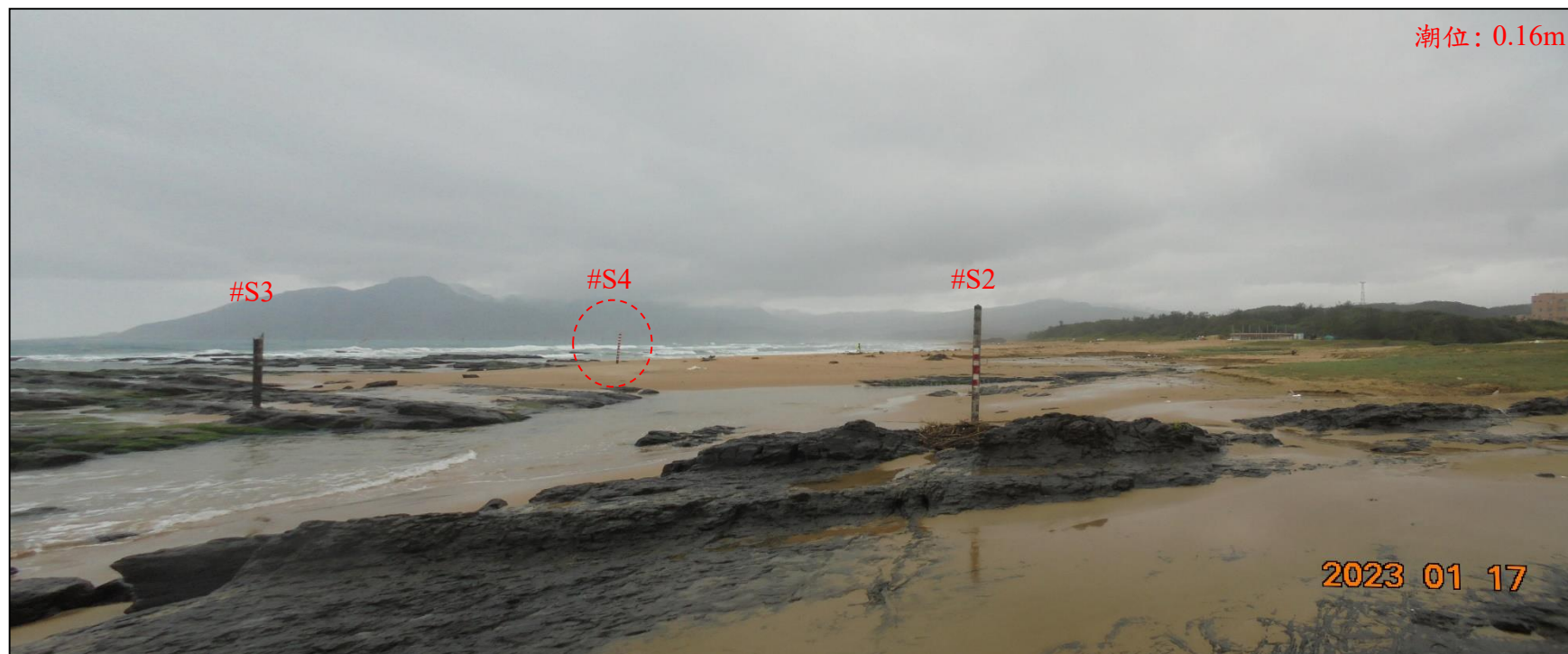
附圖 2-2 監測區北側礁石區內觀測樁位置圖(2023/01/17)
