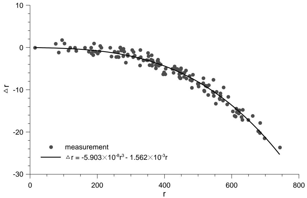
圖 3-18 攝影鏡頭編號 Cam2 之徑向扭曲迴歸結果圖
