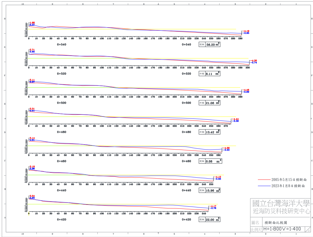
圖 4-5(c) 2023 年 1 月 8 日 B 監測區橫斷面比較圖
