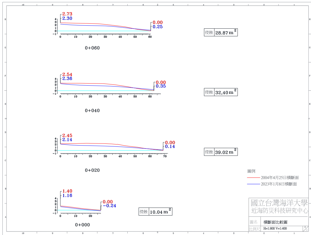
圖 4-4(j) 2023 年 1 月 8 日 A 監測區橫斷面比較圖
