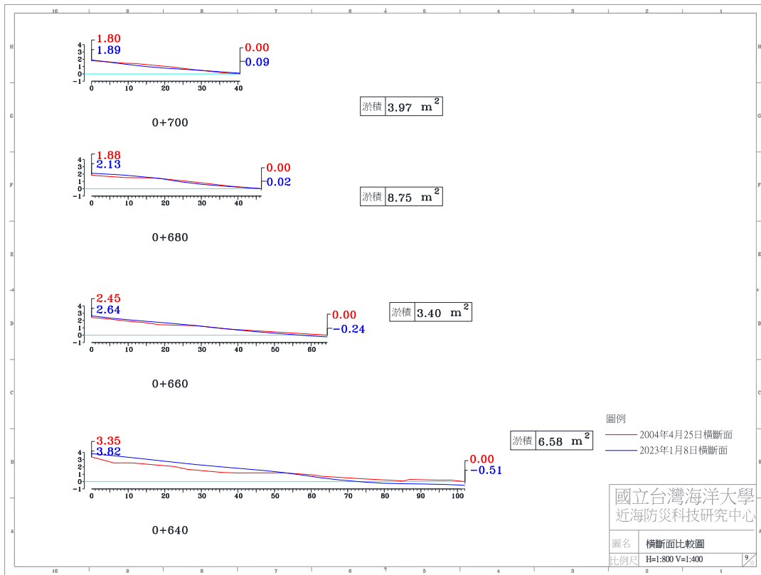
圖 4-4(b) 2023 年 1 月 8 日 A 監測區橫斷面比較圖
