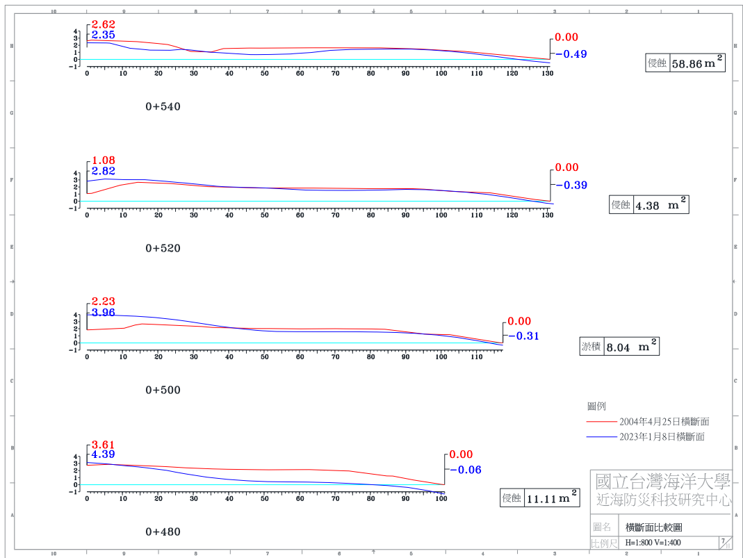
圖 4-4(d) 2023 年 1 月 8 日 A 監測區橫斷面比較圖
