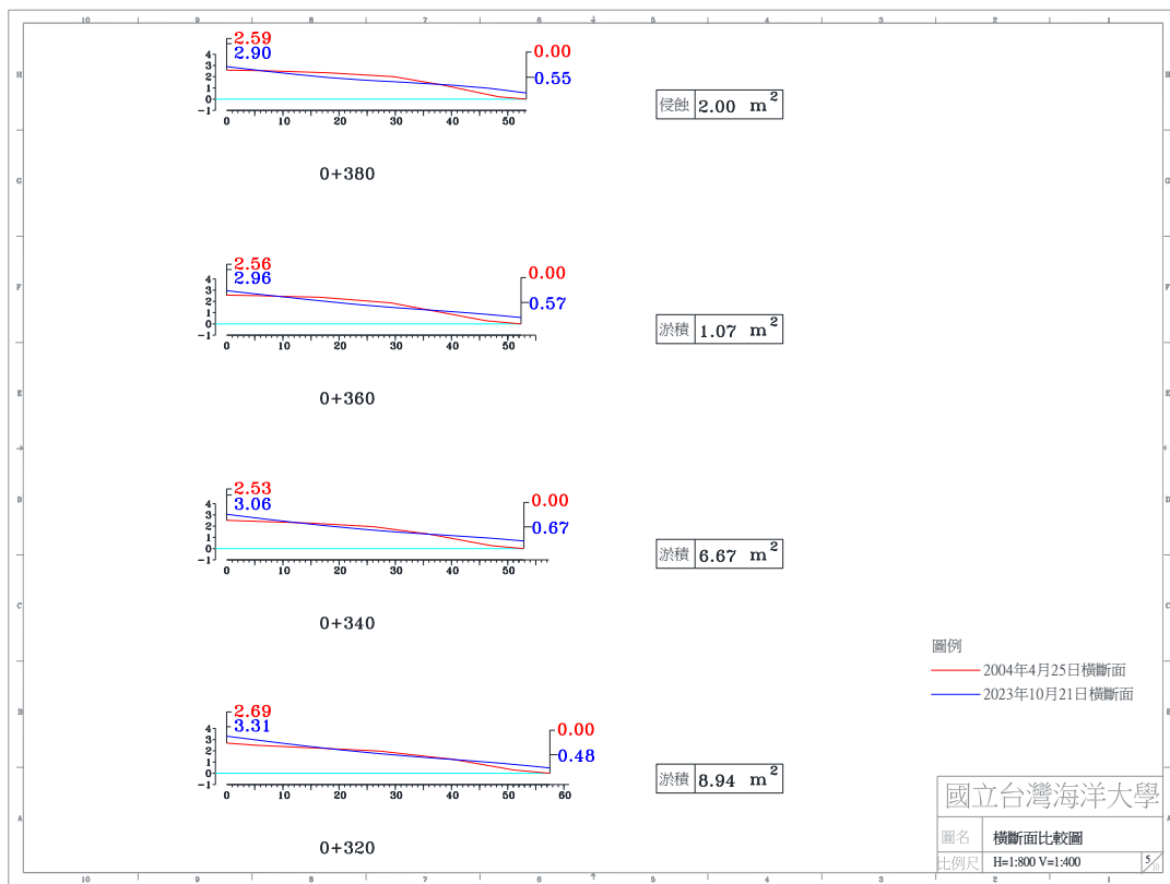
圖 4-4(f) 2023 年 10 月 21 日 A 監測區橫斷面比較圖
