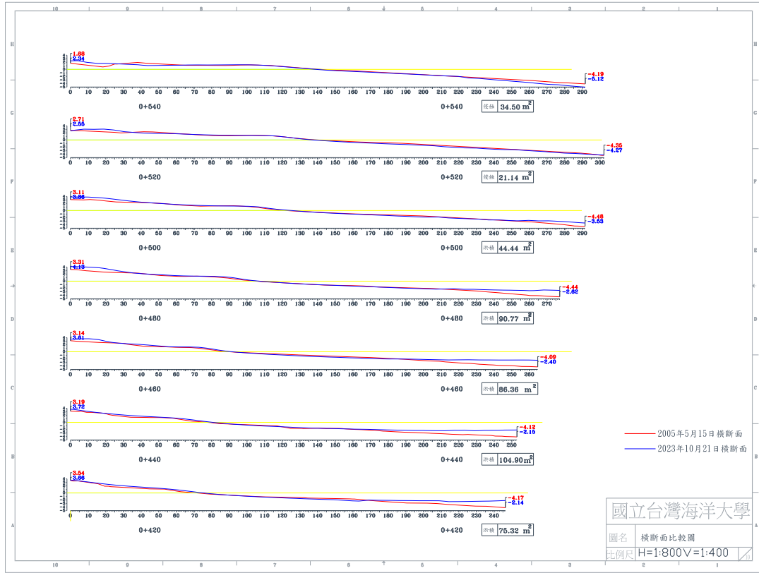
圖 4-5(c) 2023 年 10 月 21 日 B 監測區橫斷面比較圖
