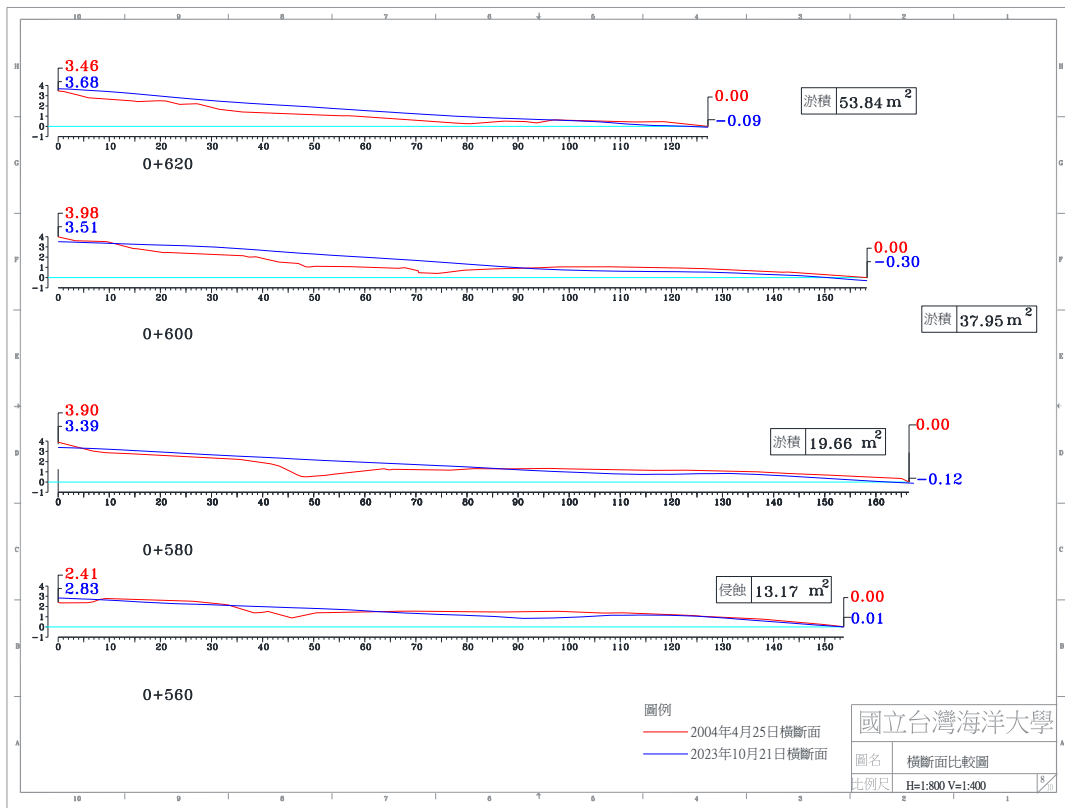
圖 4-4(c) 2023 年 10 月 21 日 A 監測區橫斷面比較圖
