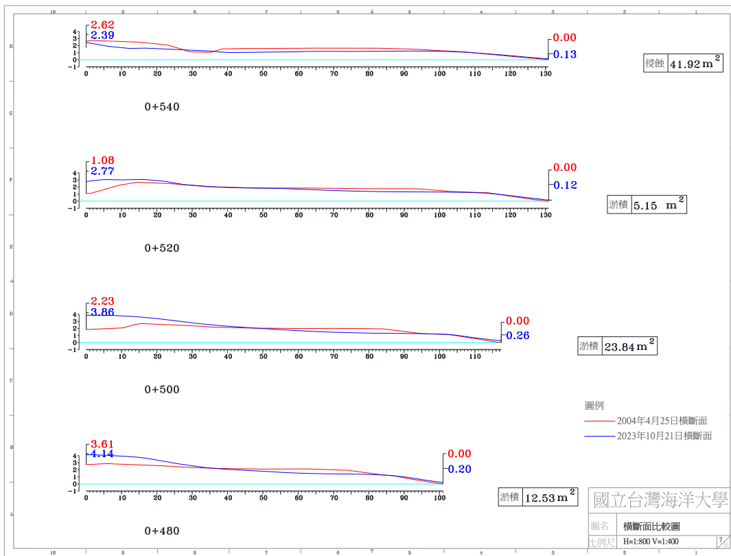
圖 4-4(d) 2023 年 10 月 21 日 A 監測區橫斷面比較圖
