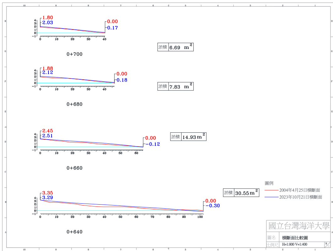
圖 4-4(b) 2023 年 10 月 21 日 A 監測區橫斷面比較圖
