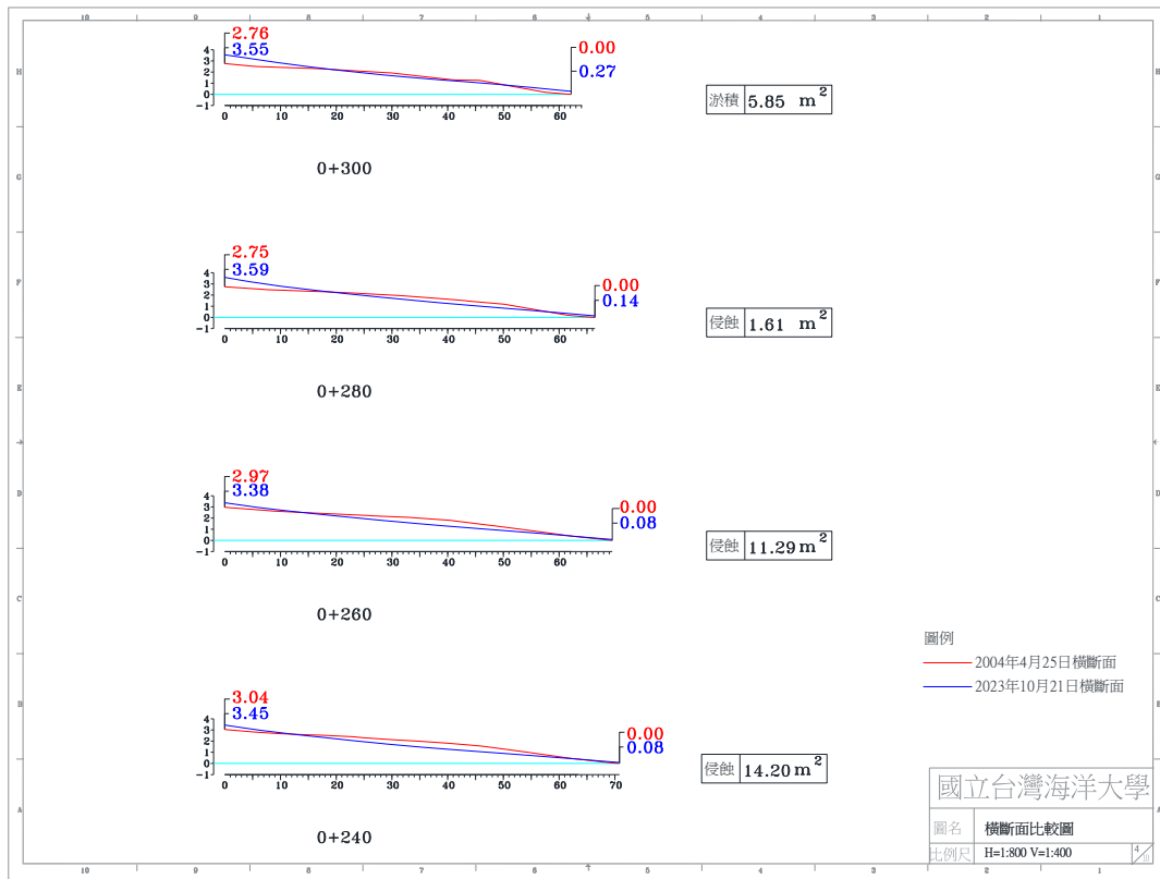
圖 4-4(g) 2023 年 10 月 21 日 A 監測區橫斷面比較圖
