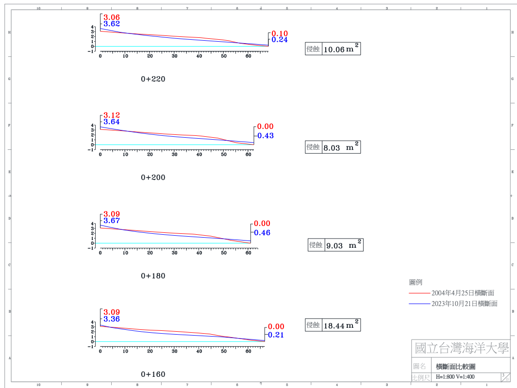
圖 4-4(h) 2023 年 10 月 21 日 A 監測區橫斷面比較圖
