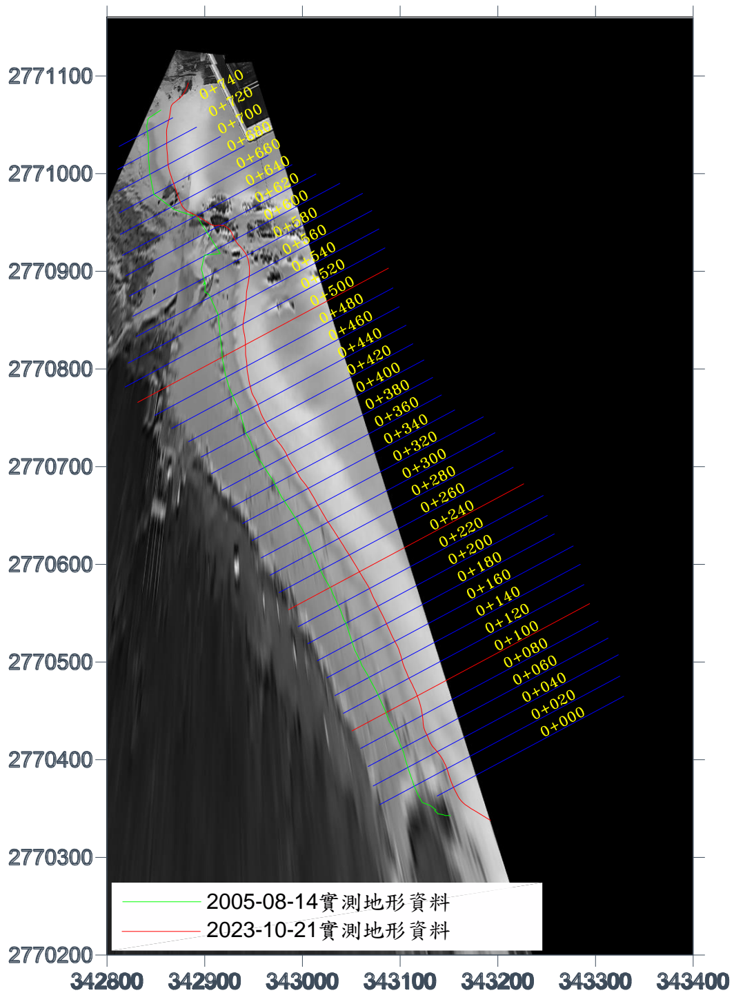
圖 4-22 長期實測 0 m 灘線比對平面示意圖(2023/10/21)
