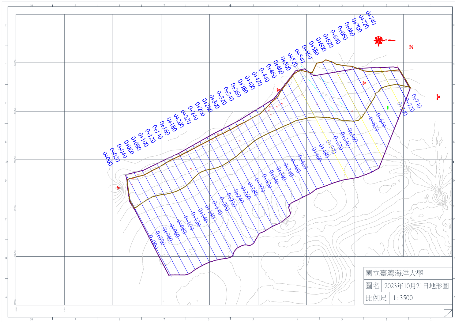
圖 4-1 2023 年 10 月 21 日監測地形
