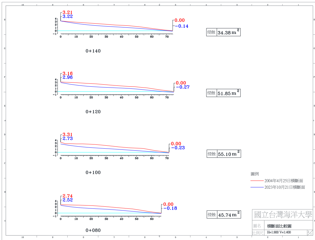
圖 4-4(i) 2023 年 10 月 21 日 A 監測區橫斷面比較圖
