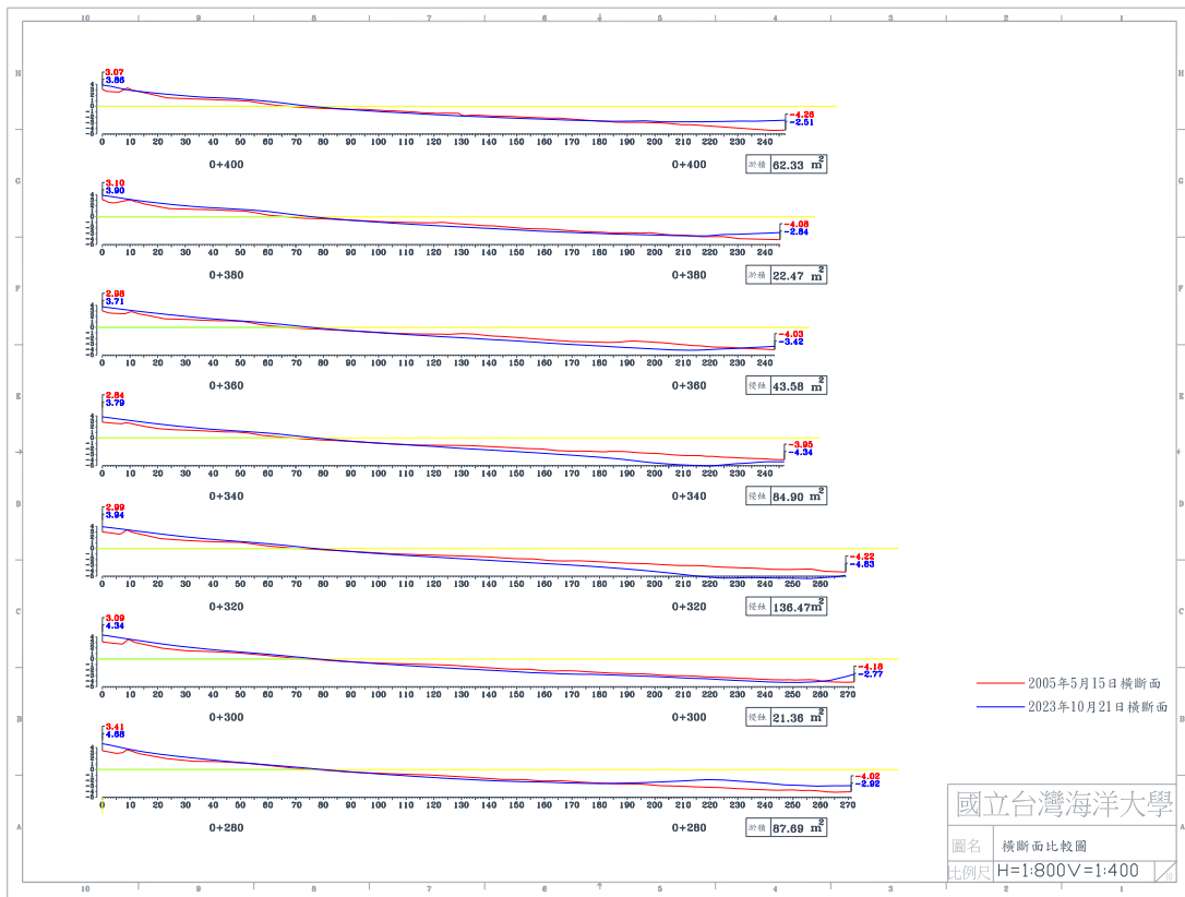
圖 4-5(d) 2023 年 10 月 21 日 B 監測區橫斷面比較圖
