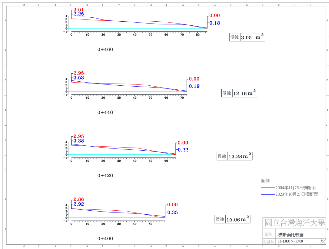
圖 4-4(e) 2023 年 10 月 21 日 A 監測區橫斷面比較圖
