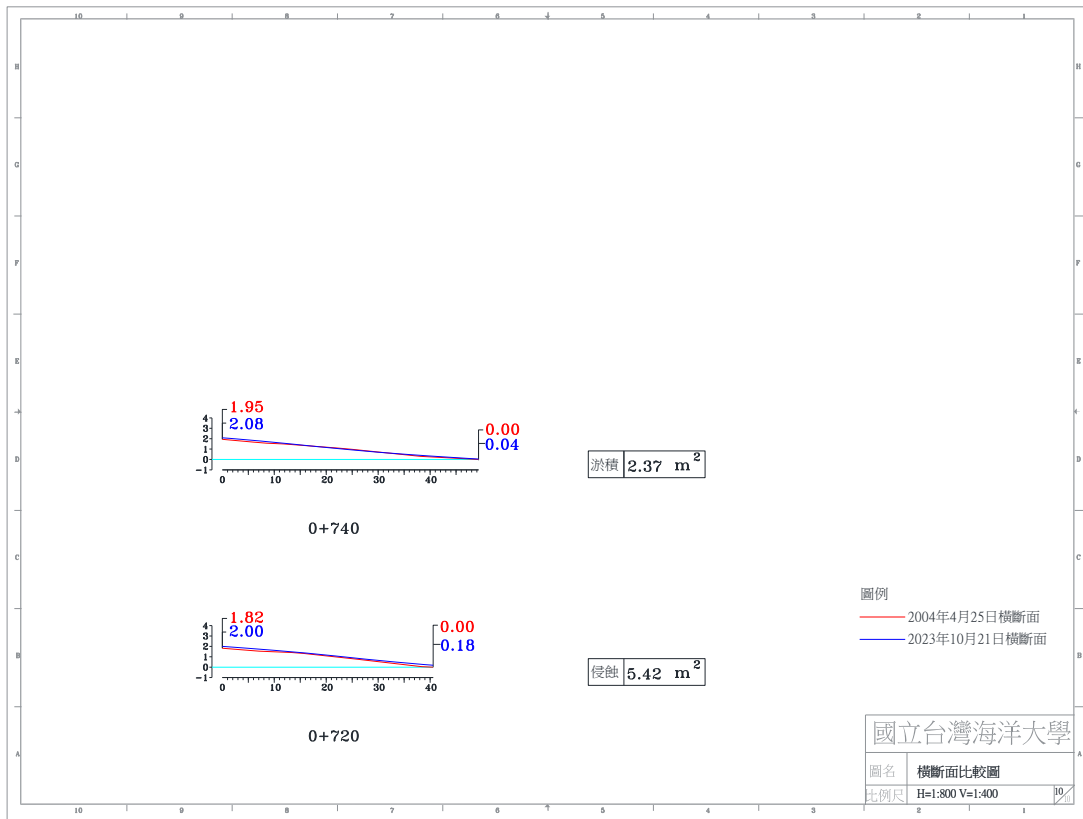
圖 4-4(a) 2023 年 10 月 21 日 A 監測區橫斷面比較圖
