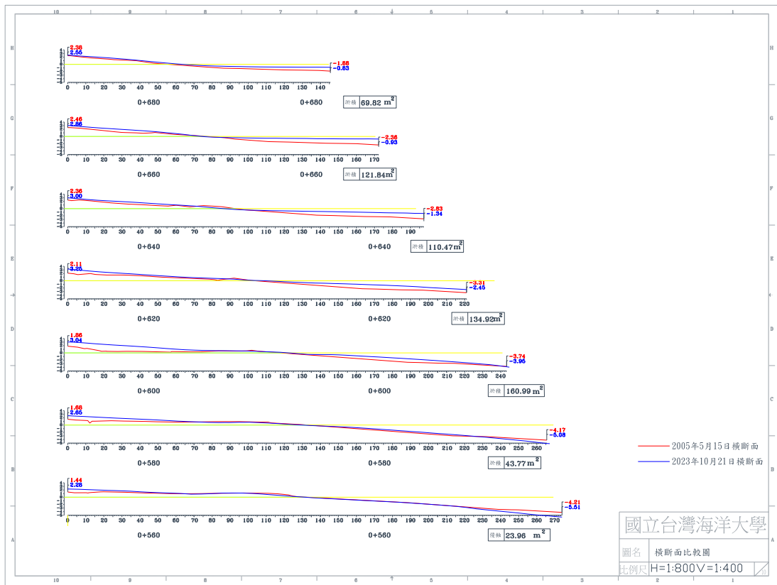
圖 4-5(b) 2023 年 10 月 21 日 B 監測區橫斷面比較圖
