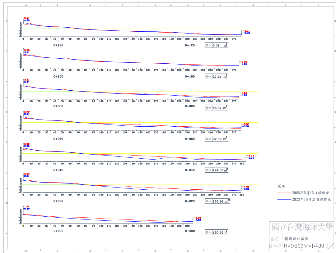
圖 4-5(f) 2023 年 10 月 21 日 B 監測區橫斷面比較圖
