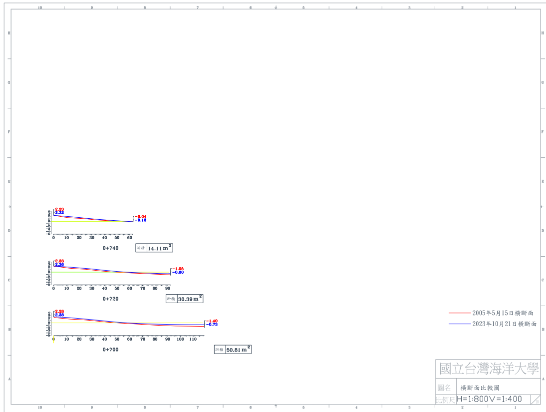
圖 4-5(a) 2023 年 10 月 21 日 B 監測區橫斷面比較圖
