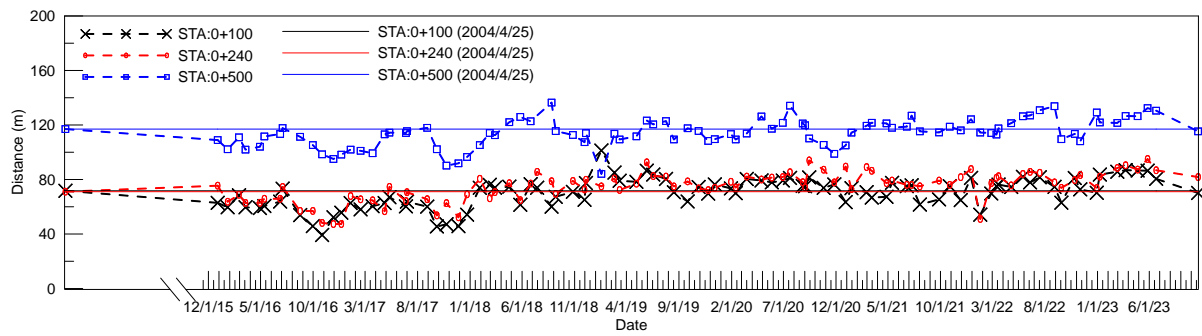
圖 4-21 岸線斷面沙灘寬度變化圖(2023/10/21)
