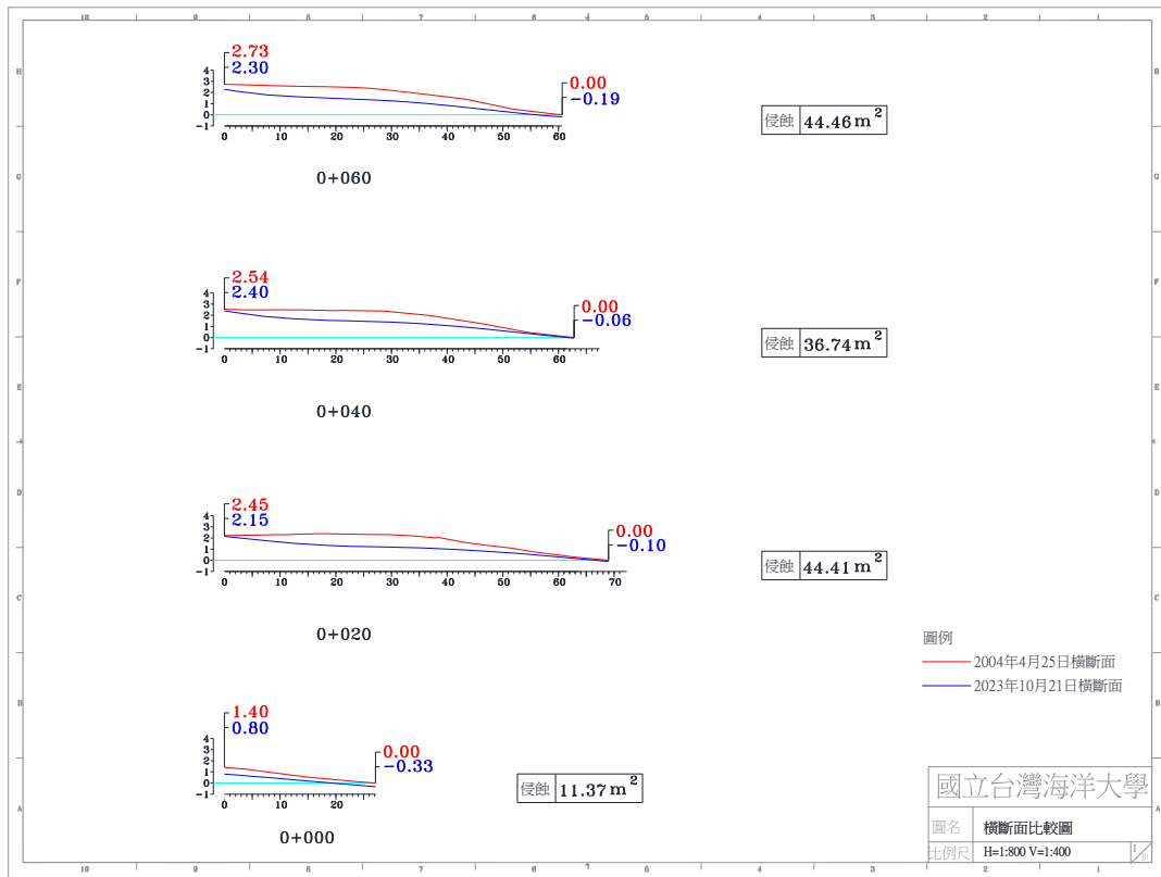
圖 4-4(j) 2023 年 10 月 21 日 A 監測區橫斷面比較圖
