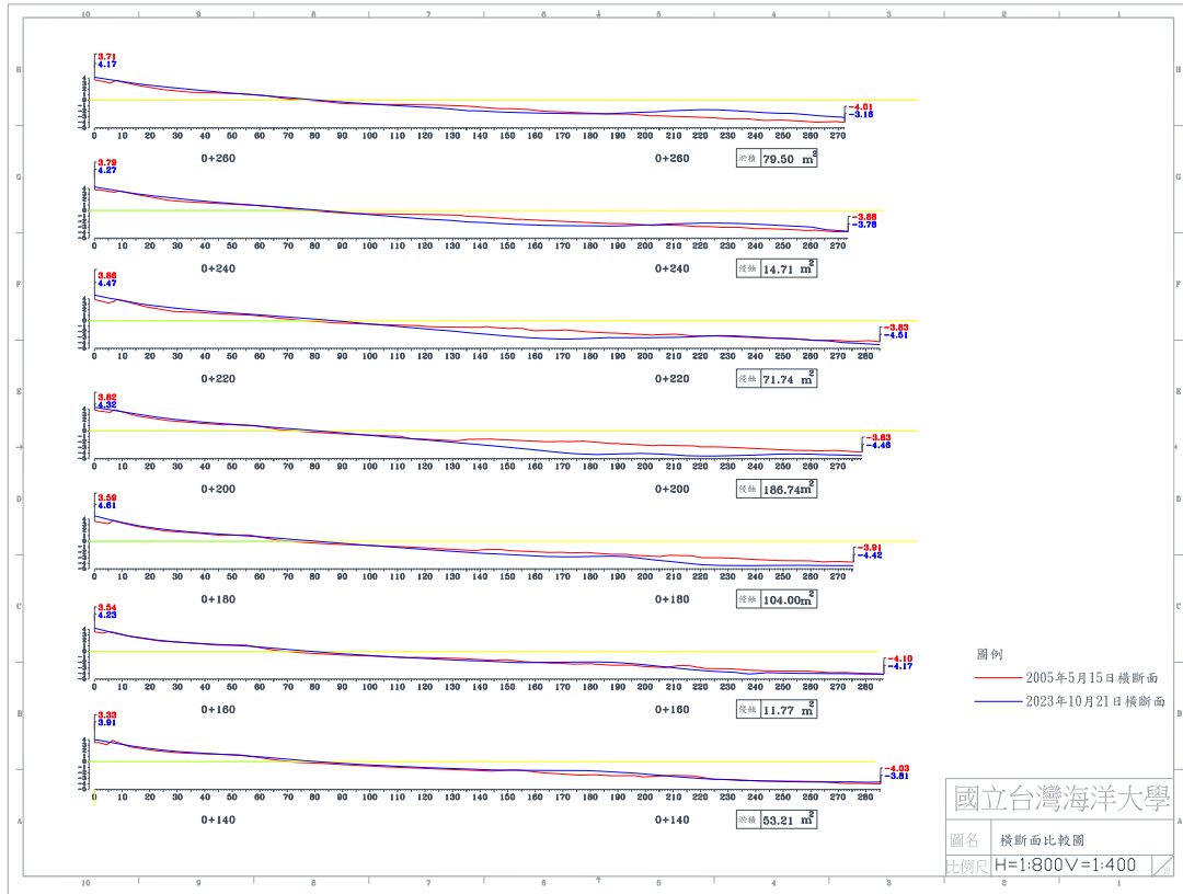
圖 4-5(e) 2023 年 10 月 21 日 B 監測區橫斷面比較圖
