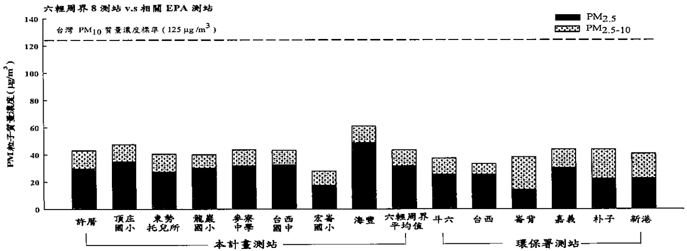
圖 2.1.1-5 本季六輕周界測站與 EPA 相關測站粒狀物濃度比較
