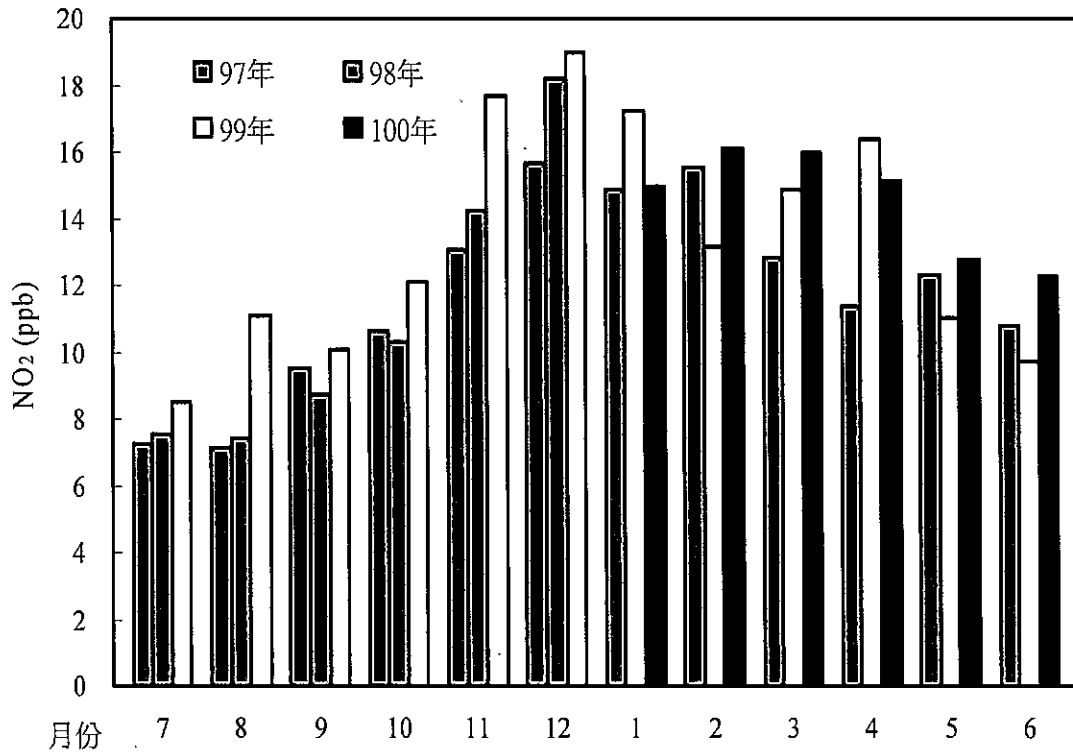
圖 2.1.5-60 土庫站 100 年第二季與 99 年及 98 年二氧化氮月平均比較圖
