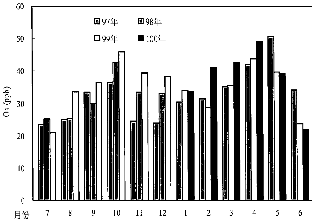
圖 2.1.5-53 台西站 100 年第二季與 99 年及 98 年臭氧月平均比較圖
