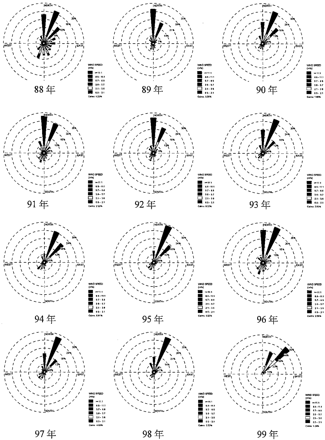
圖 2.6.1-5 88-99 年歷年台西站之風花圖
