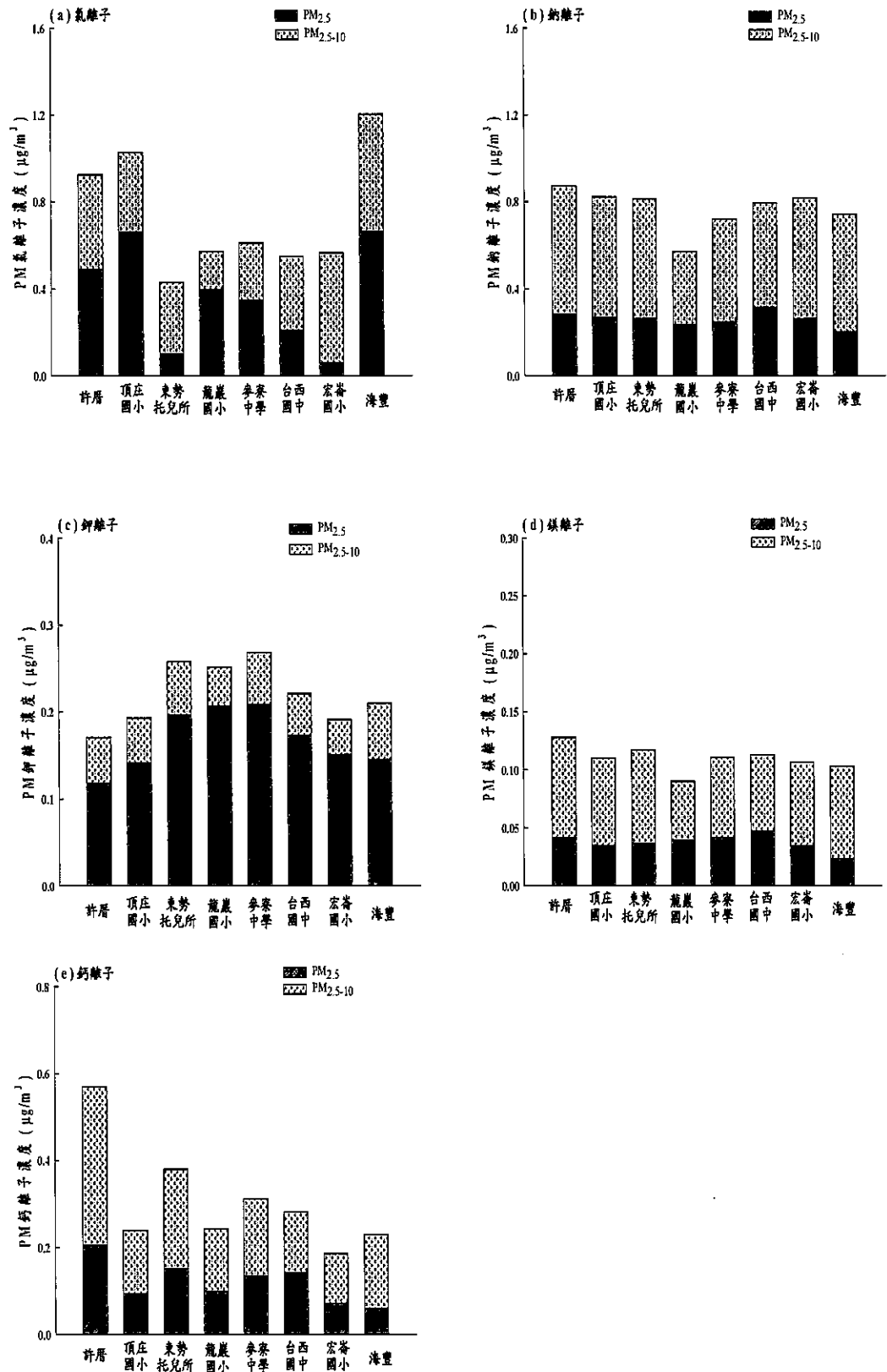
圖 2.1.1-4 本各採樣點 \text{PM}_{2.5} 及 \text{PM}_{2.5-10} 無機離子濃度
