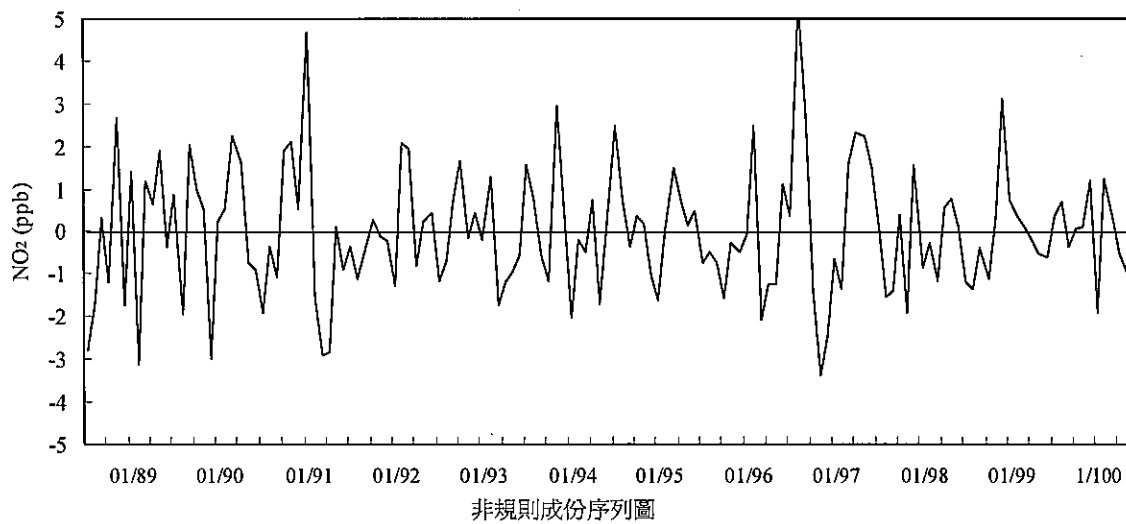
圖 2.1.5-14 台西站 88-100 年第二季間二氧化氮濃度趨勢圖
