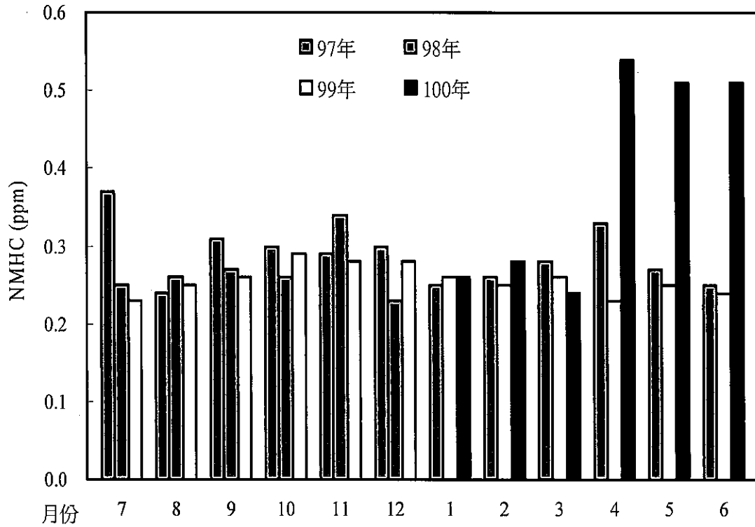
圖 2.1.5-62 台西站 100 年第二季與 99 年及 98 年 NMHC 月平均比較圖
