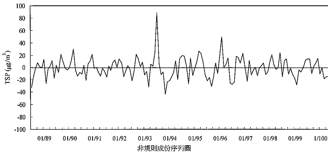
圖 2.1.5-19 麥寮站 88-100 年第二季間總懸浮微粒 TSP 濃度趨勢圖
