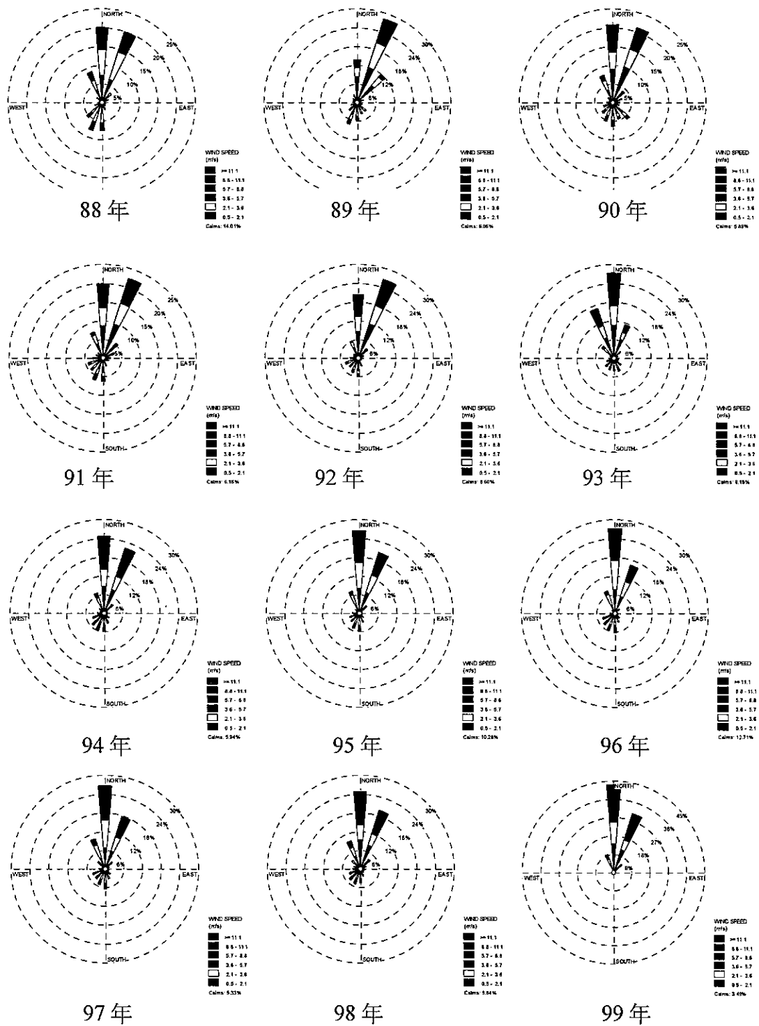
圖 2.6.1-6 88-99 年歷年土庫站之風花圖
