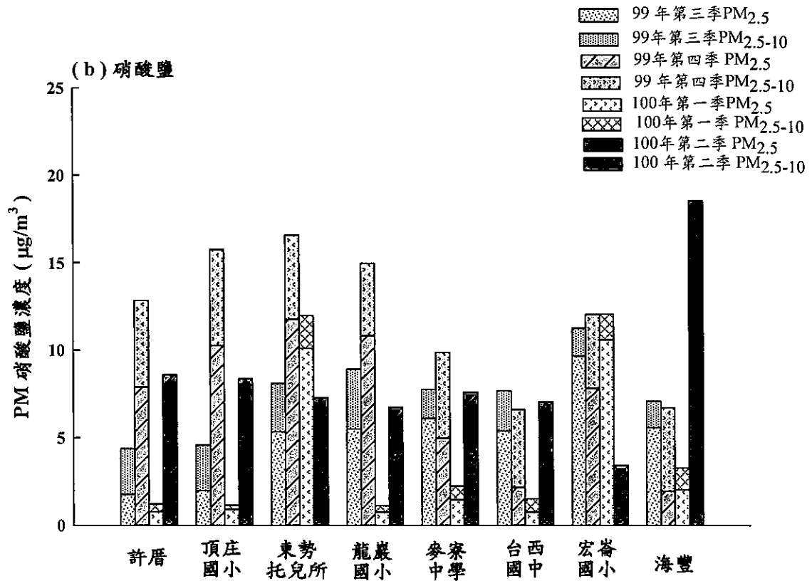
圖 2.1.1-8 本計畫四季各採樣點 PM 2.5 及 PM 2.5-10 硫酸鹽與硝酸鹽濃度
