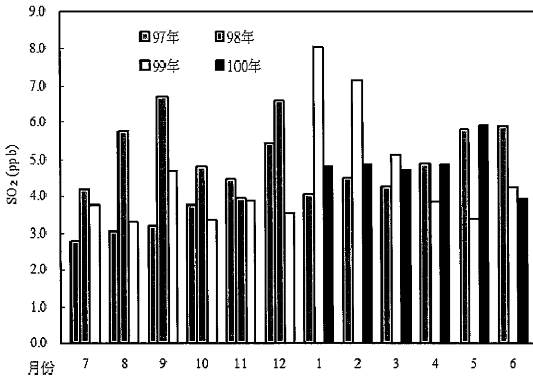
圖 2.1.5-47 台西站 100 年第二季與 99 年及 98 年二氧化硫月平均比較圖
