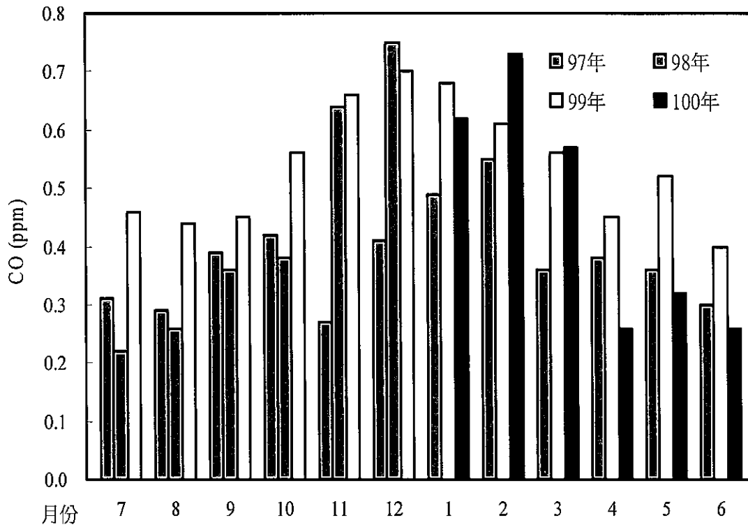
圖 2.1.5-51 土庫站 100 年第二季與 99 年及 98 年一氧化碳月平均比較圖
