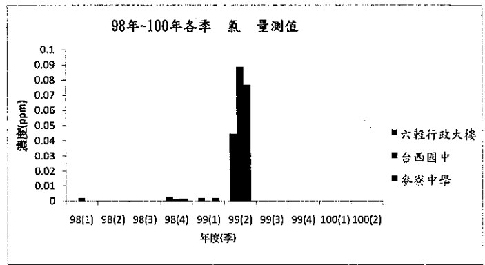
圖 2.1.4-8 98 年至 100 年 1-2 季 氯 物種彙整
