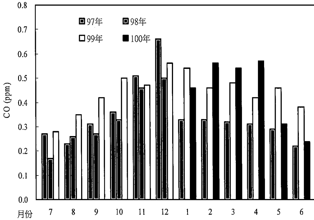
圖 2.1.5-50 台西站 100 年第二季與 99 年及 98 年一氧化碳月平均比較圖
