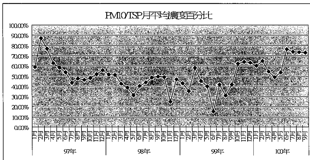
圖 3.2-1 歷年 PM 10 與 TSP 月平均濃度百分比趨勢圖
