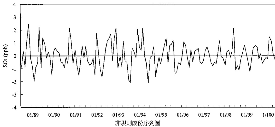
圖 2.1.5-1 麥寮站 88 - 100 年第二季間二氧化硫濃度趨勢圖
