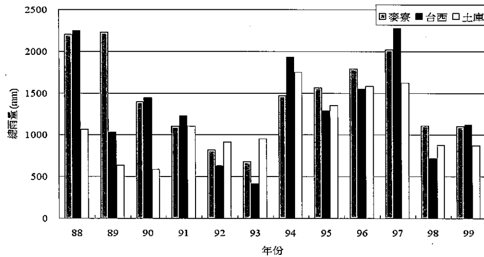
圖 2.1.6-3 台塑三測站歷年總雨量資料比較圖
