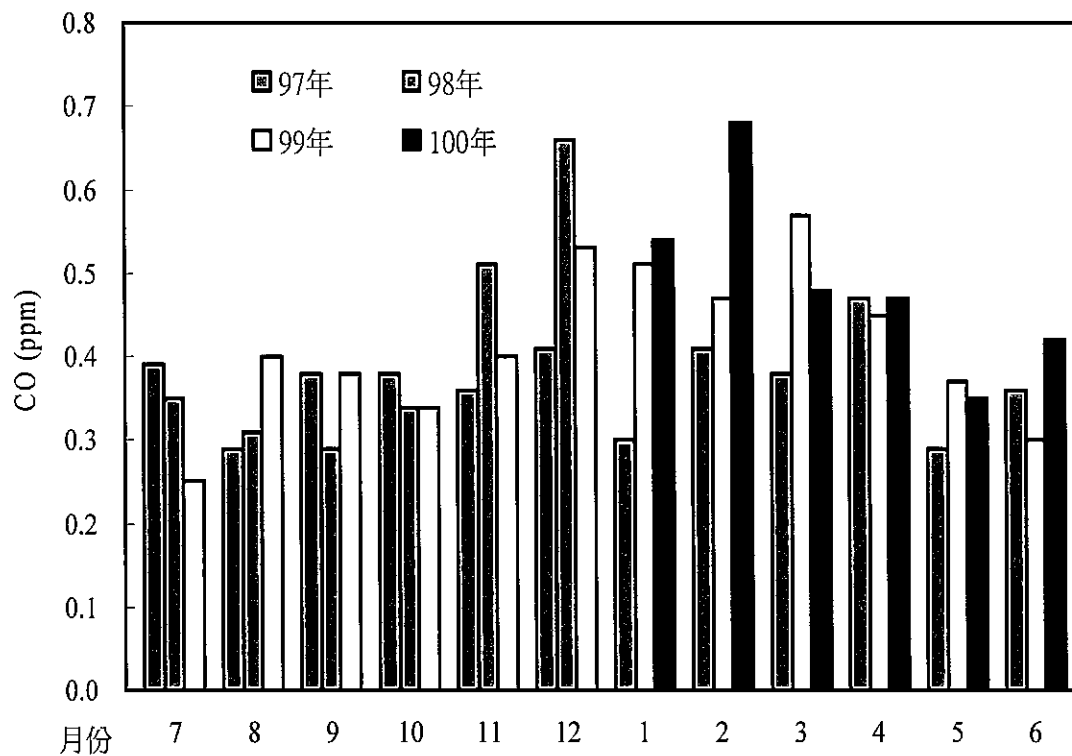
圖 2.1.5-49 麥寮站 100 年第二季與 99 年及 98 年一氧化碳月平均比較圖
