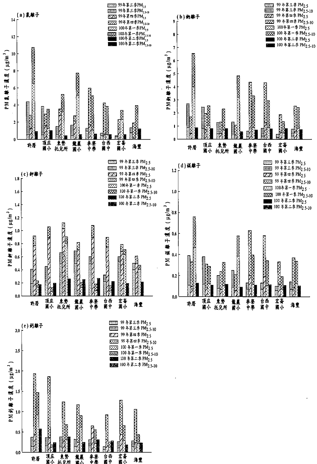
圖 2.1.1-9 本計畫四季各採樣點 \text{PM}_{2.5} 及 \text{PM}_{2.5-10} 無機離子濃度
