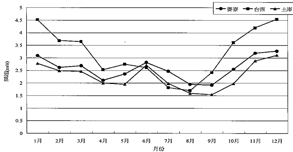
圖 2.1.6-9 92 年台塑三測站月平均風速資料比較圖
