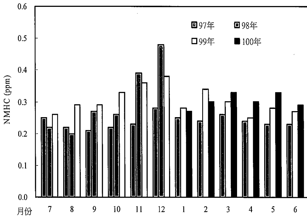
圖 2.1.5-63 土庫站 100 年第二季與 99 年及 98 年 NMHC 月平均比較圖
