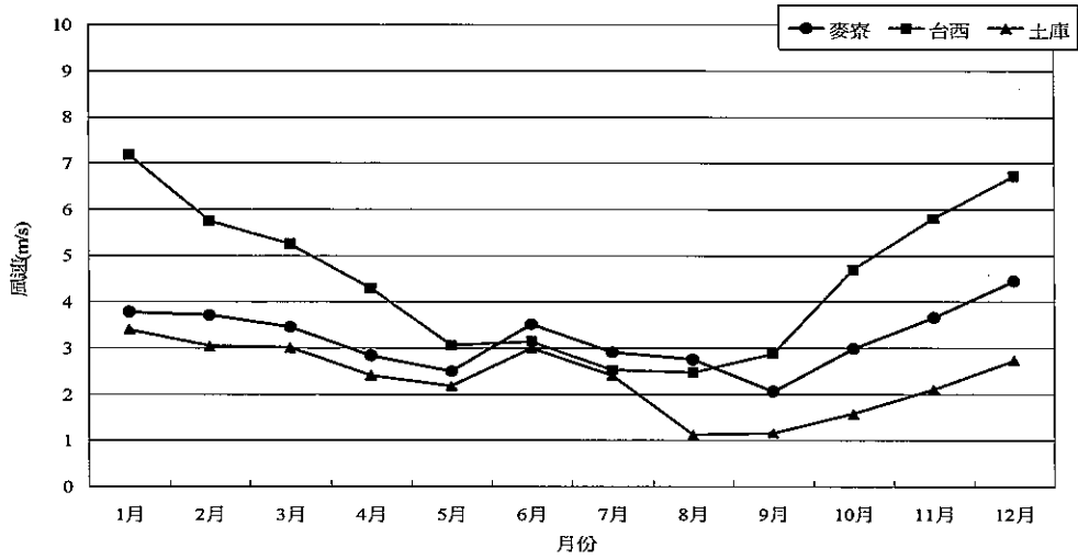
圖 2.1.6-7 88 年台塑三測站月平均風速資料比較圖
