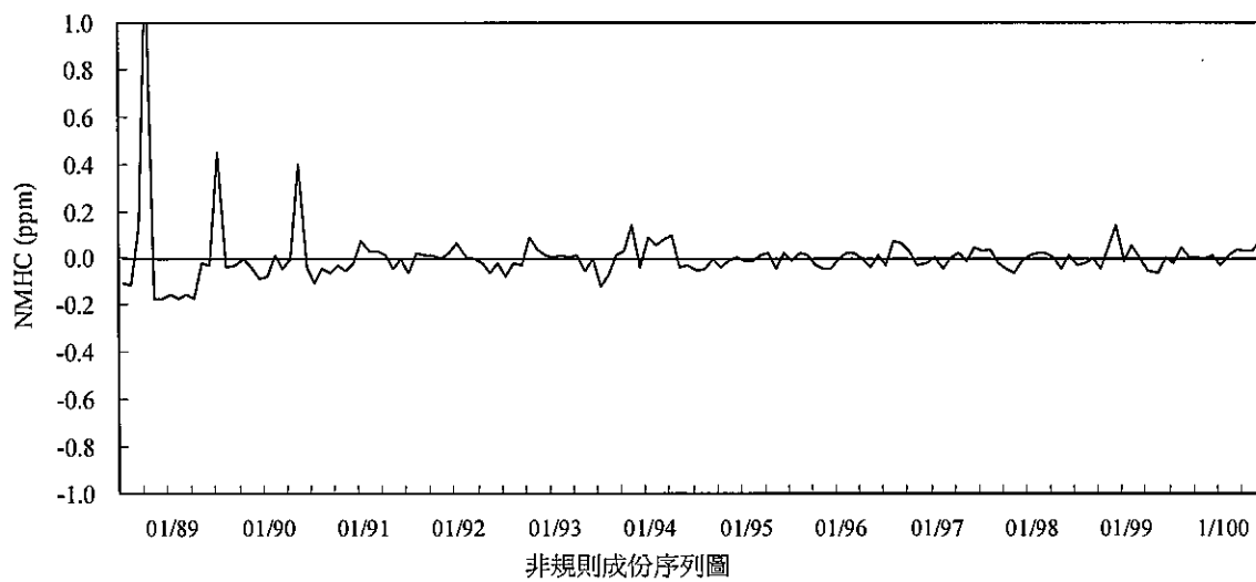
圖 2.1.5-18 土庫站 88-100 年第二季間非甲烷碳氫化合物 NMHC 濃度趨勢圖
