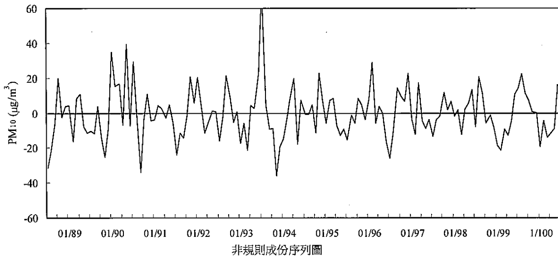
圖 2.1.5-10 麥寮站 88-100 年第二季間懸浮微粒 PM 10 濃度趨勢圖
