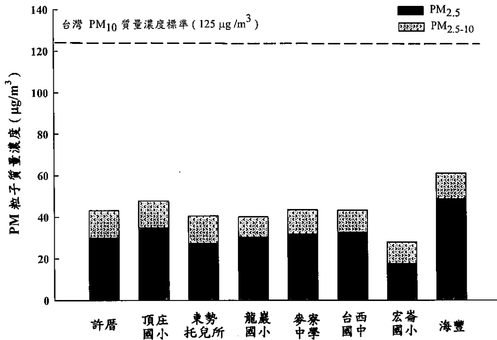
圖 2.1.1-1 本季各採樣點 PM 2.5 及 PM 2.5-10 質量濃度
