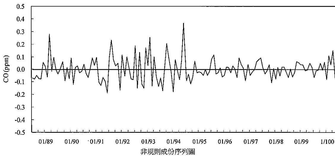
圖 2.1.5-5 台西站 88-100 年第二季間一氧化碳濃度趨勢圖
