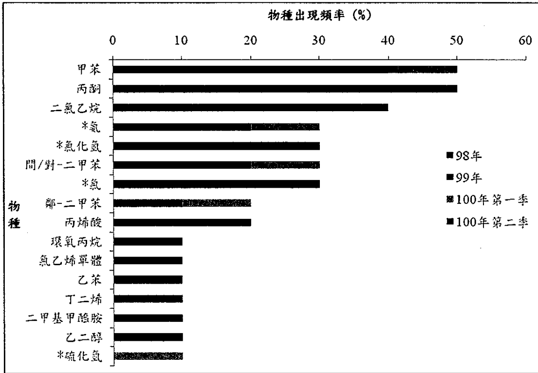
圖 2.1.4-2 行政大樓歷年 (98、99~100年1季~2季) 共十季物種測得頻率排序
