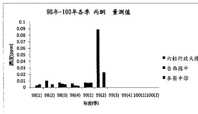
圖 2.1.4-7 98 年至 100 年 1-2 季 丙酮 物種彙整
