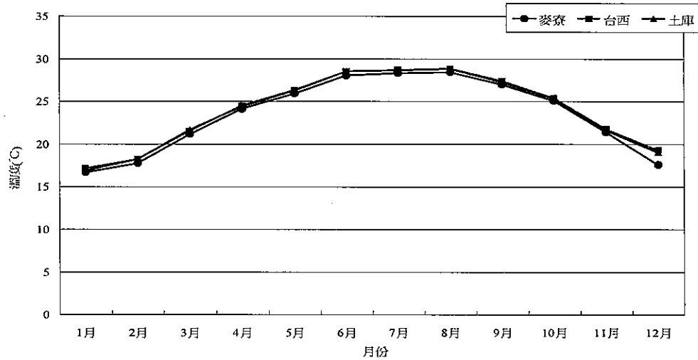
圖 2.1.6-11 91年台塑三測站月平均溫度資料比較圖
