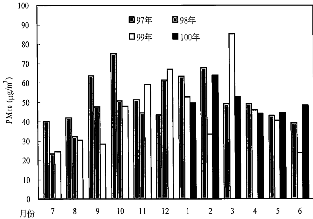
圖 2.1.5-56 台西站 100 年第二季與 99 年及 98 年懸浮微粒 PM 10 月平均比較圖
