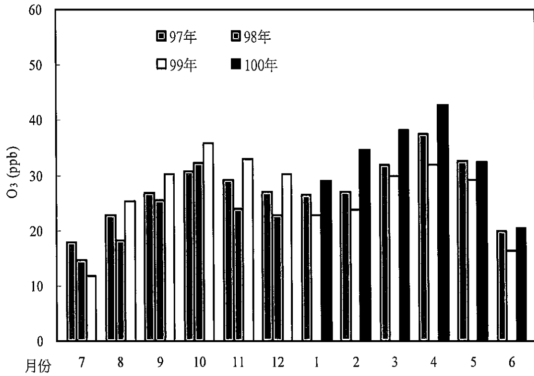
圖 2.1.5-54 土庫站 100 年第二季與 99 年及 98 年臭氧月平均比較圖
