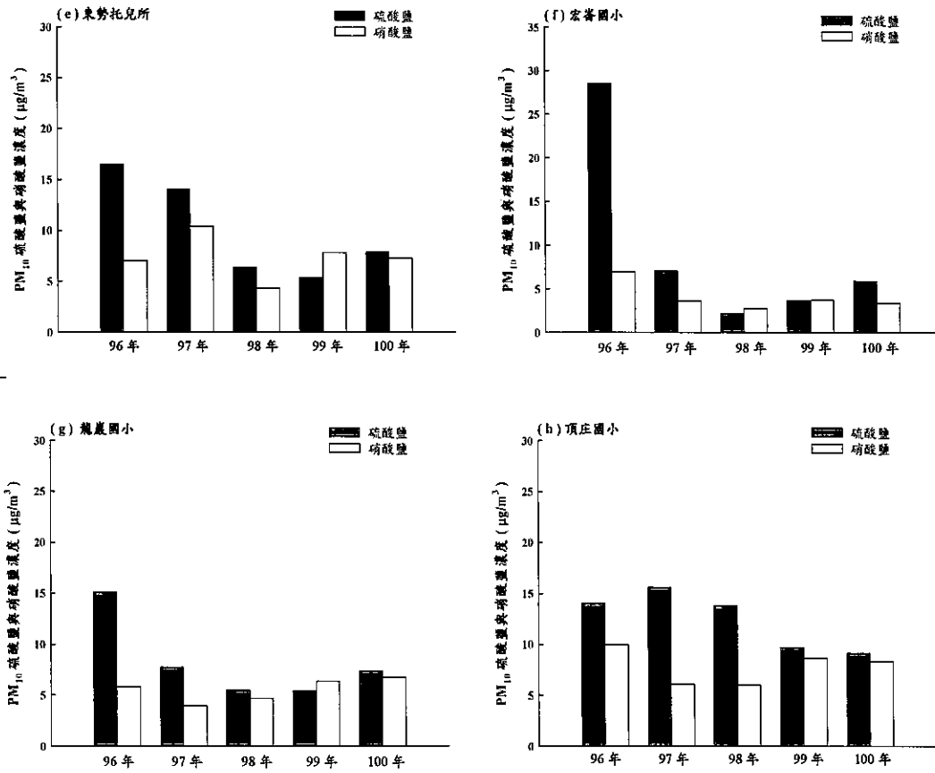
圖 2.1.2-2 96 - 100 年第二季各採樣點 PM 10 硫酸鹽與硝酸鹽濃度
