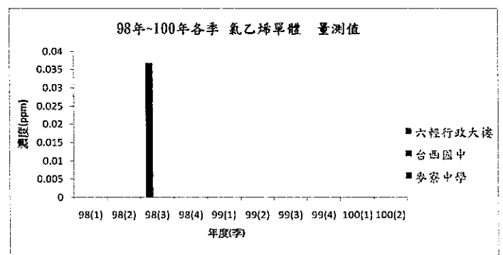
圖 2.1.4-10 98 年至 100 年 1-2 季 氯乙烯單體 物
