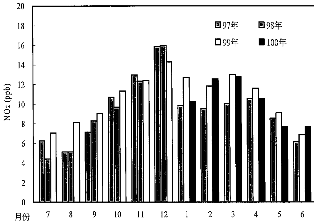
圖 2.1.5-59 台西站 100 年第二季與 99 年及 98 年二氧化氮月平均比較圖
