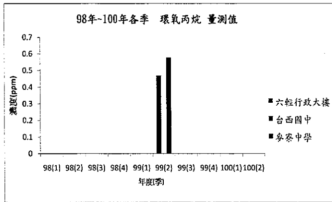
圖 2.1.4-5 98 年至 100 年 1-2 季 環氧丙烷 物種
