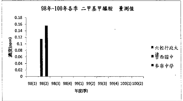
圖 2.1.4-14 98 年至 100 年 1-2 季 二甲基甲醯胺 物
