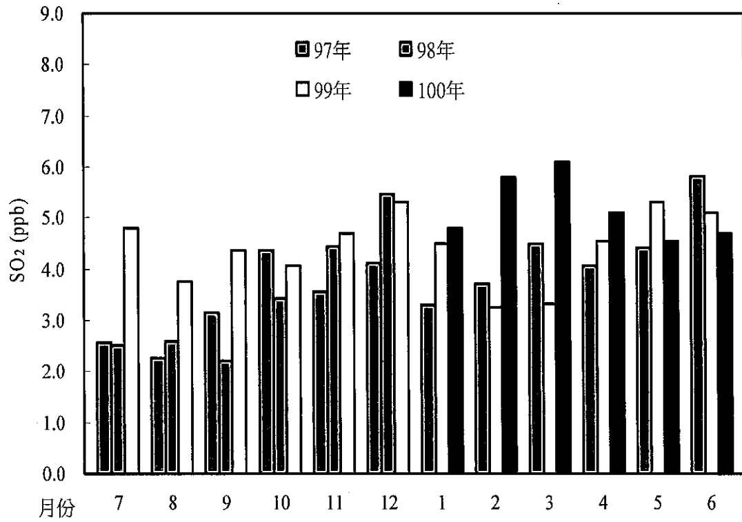
圖 2.1.5-46 麥寮站 100 年第二季與 99 年及 98 年二氧化硫月平均比較圖
