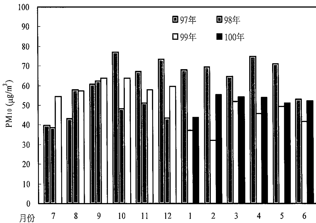
圖 2.1.5-55 麥寮站 100 年第二季與 99 年及 98 年懸浮微粒 PM 10 月平均比較圖
