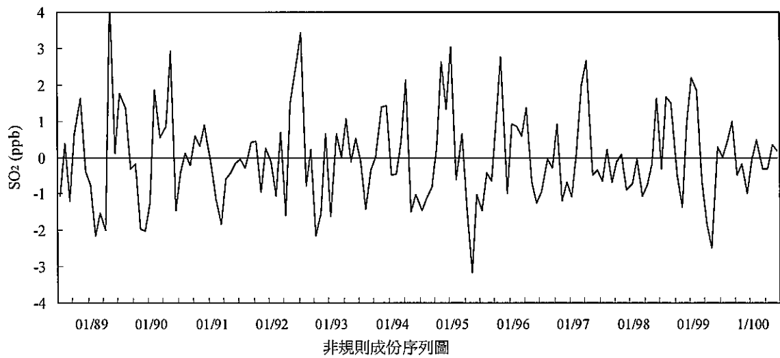
圖 2.1.5-2 台西站 88 - 100 年第二季間二氧化硫濃度趨勢圖
