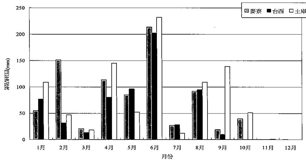
圖 2.1.6-15 92年台塑三測站月總雨量資料比較圖
