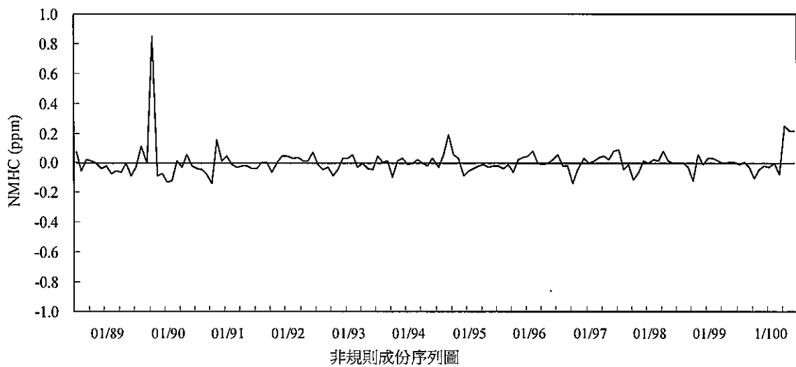
圖 2.1.5-17 台西站 88-100 年第二季間非甲烷碳氫化合物 NMHC 濃度趨勢圖
