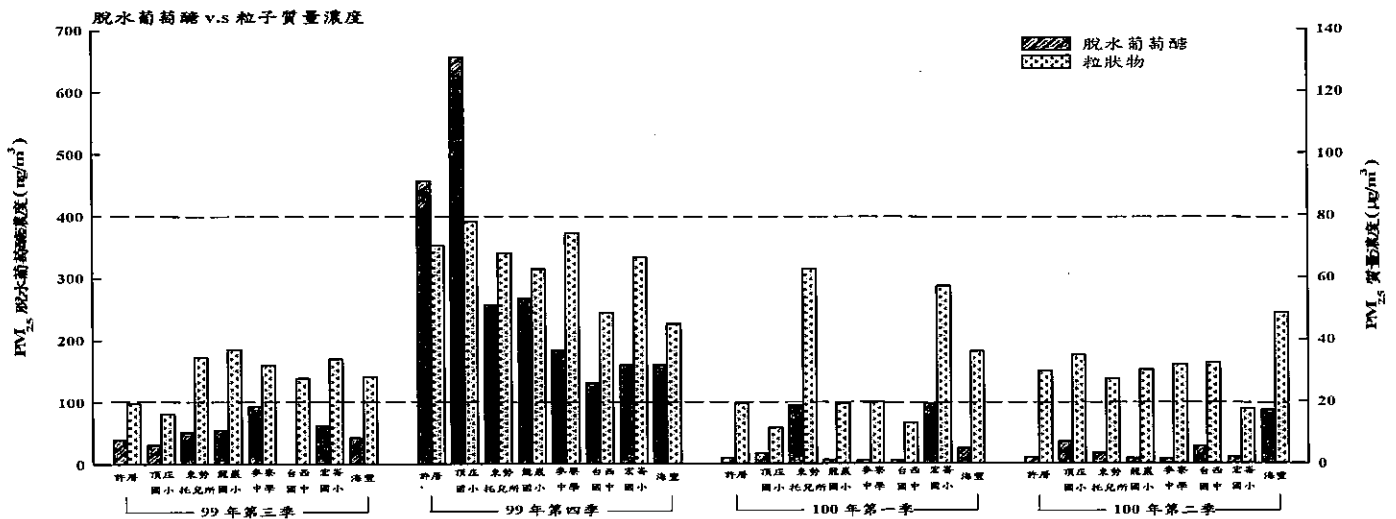
圖 2.1.1-7 本計畫四季各採樣點 PM 2.5 脫水葡萄糖與粒子質量濃度
