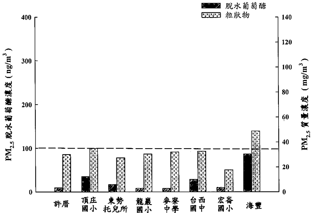
圖 2.1.1-3 本季各採樣點 PM 2.5 脫水葡萄糖與粒子質量濃度
