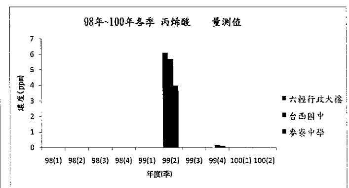
圖 2.1.4-12 98 年至 100 年 1-2 季 丙烯酸 物種
