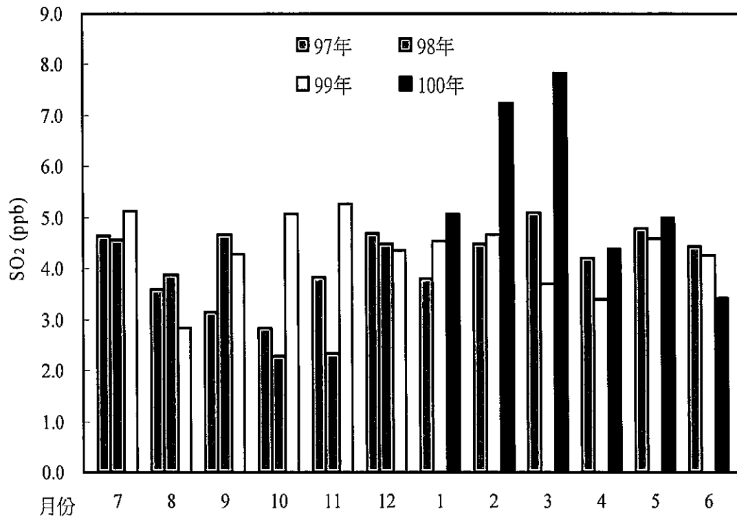
圖 2.1.5-48 土庫站 100 年第二季與 99 年及 98 年二氧化硫月平均比較圖
