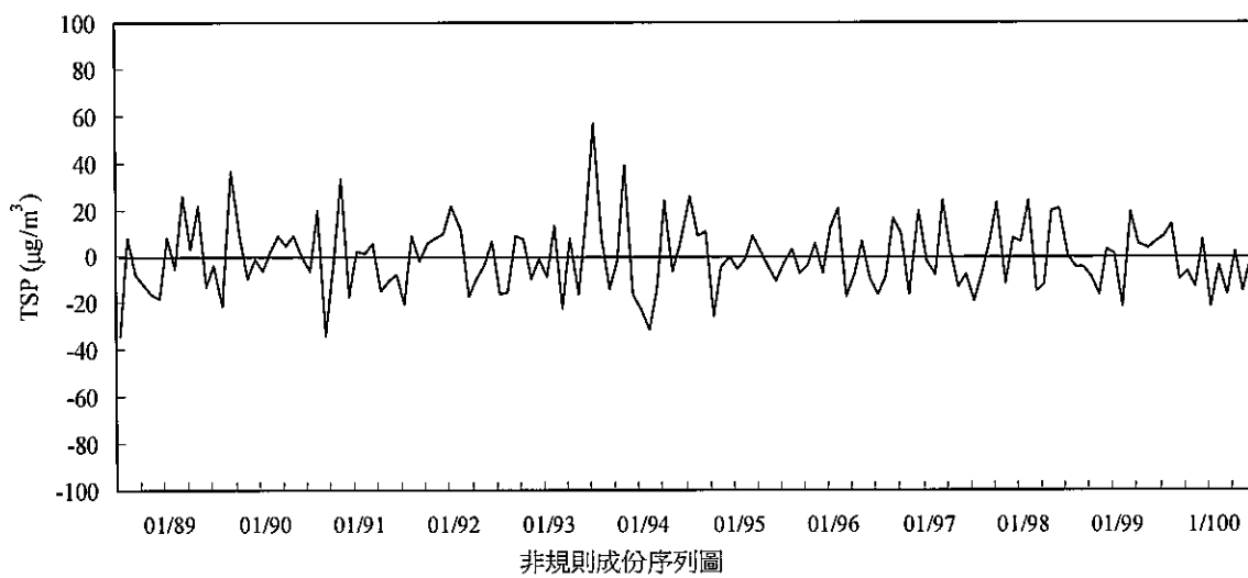
圖 2.1.5-21 土庫站 88-100 年第二季間總懸浮微粒 TSP 濃度趨勢
