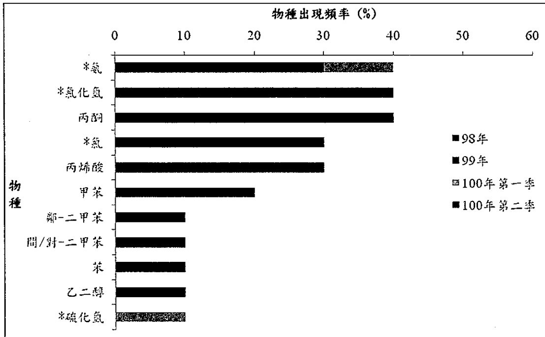
圖 2.1.4-3 台西國中歷年 (98、99~100年1季~2季) 共十季物種測得頻率排序
