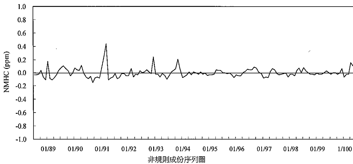
圖 2.1.5-16 麥寮站 88-100 年第二季間非甲烷碳氫化合物 NMHC 濃度趨勢圖
