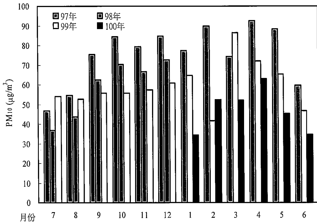
圖 2.1.5-57 土庫站 100 年第二季與 99 年及 98 年懸浮微粒 PM 10 月平均比較圖
