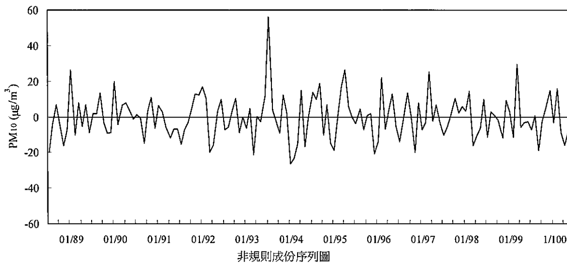
圖 2.1.5-11 台西站 88-100 年第二季間懸浮微粒 PM 10 濃度趨勢圖
