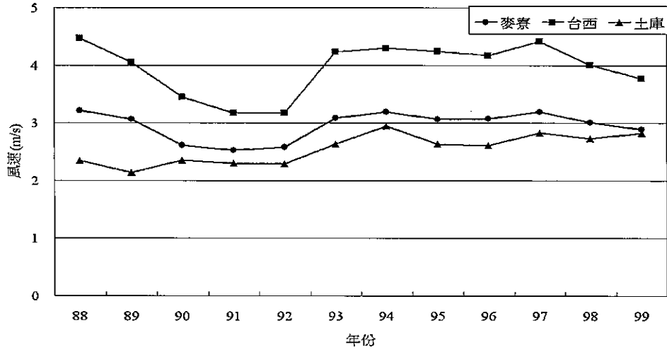
圖 2.1.6-1 台塑三測站歷年平均風速資料比較圖
