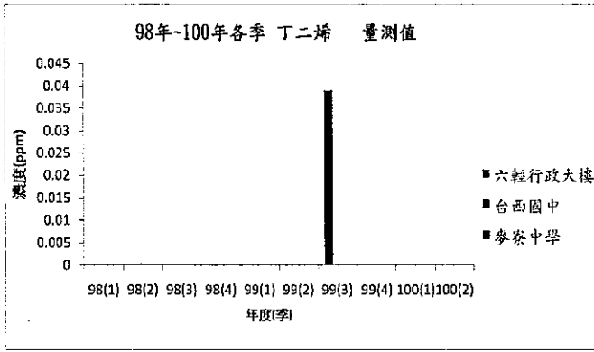
圖 2.1.4-13 98 年至 100 年 1-2 季 丁二烯 物種
