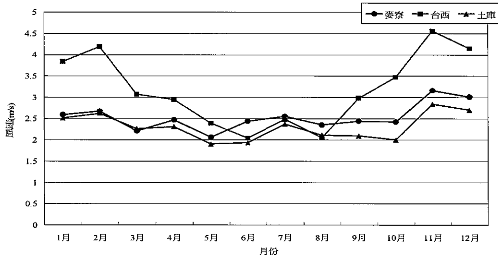
圖 2.1.6-8 91 年台塑三測站月平均風速資料比較圖
