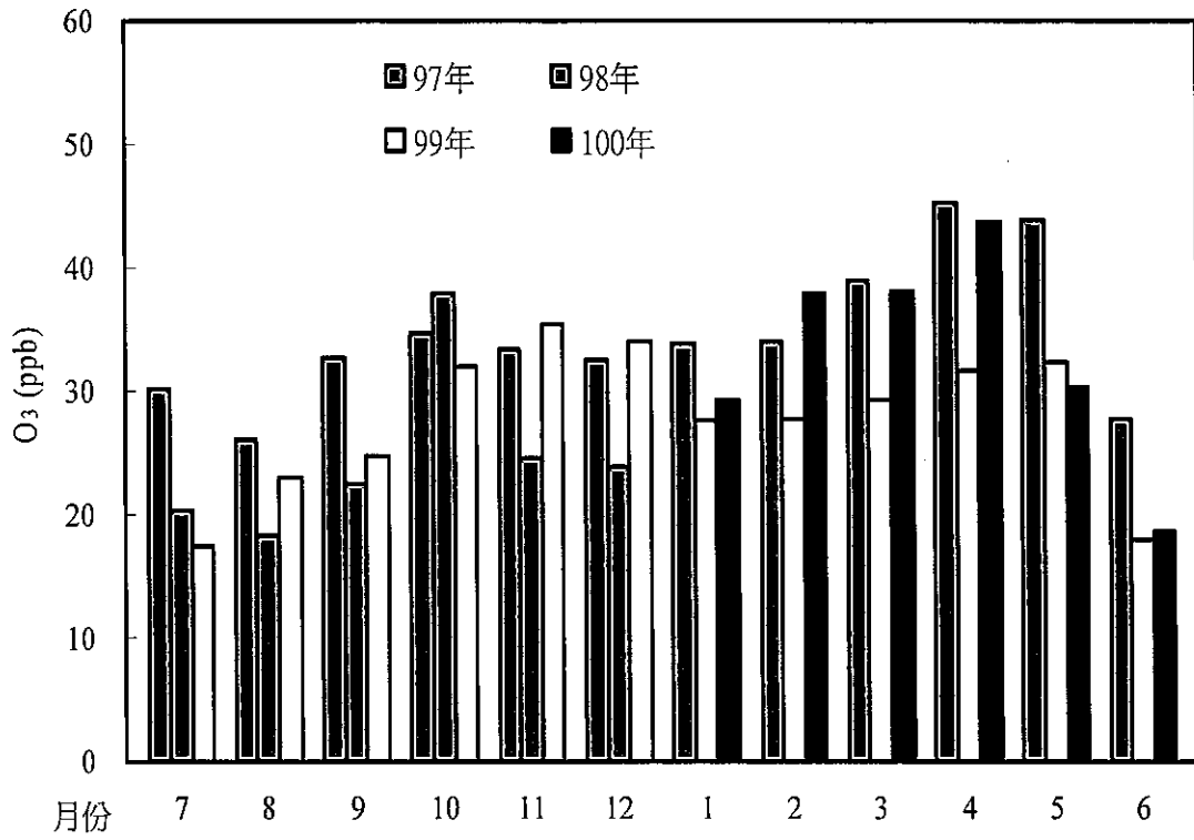
圖 2.1.5-52 麥寮站 100 年第二季與 99 年及 98 年臭氧月平均比較圖
