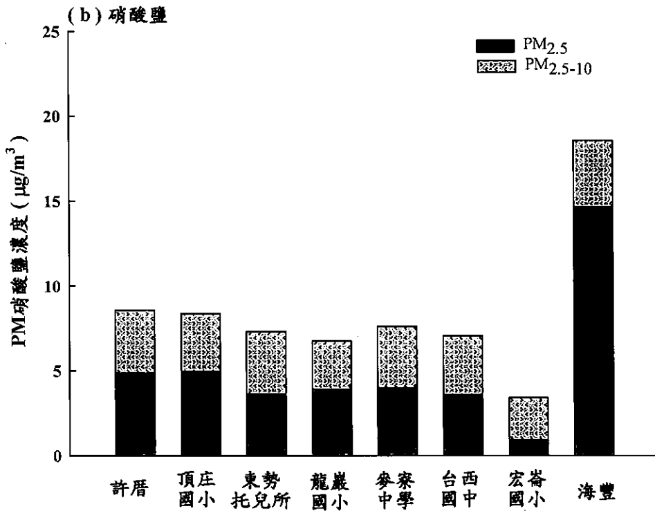
圖 2.1.1-2 本季各採樣點 PM 2.5 及 PM 2.5-10 硫酸鹽與硝酸鹽濃度
