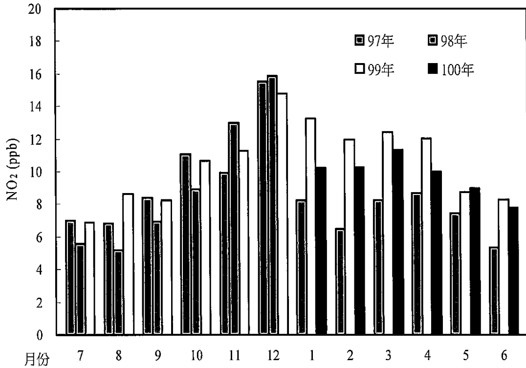
圖 2.1.5-58 麥寮站 100 年第二季與 99 年及 98 年二氧化氮月平均比較圖
