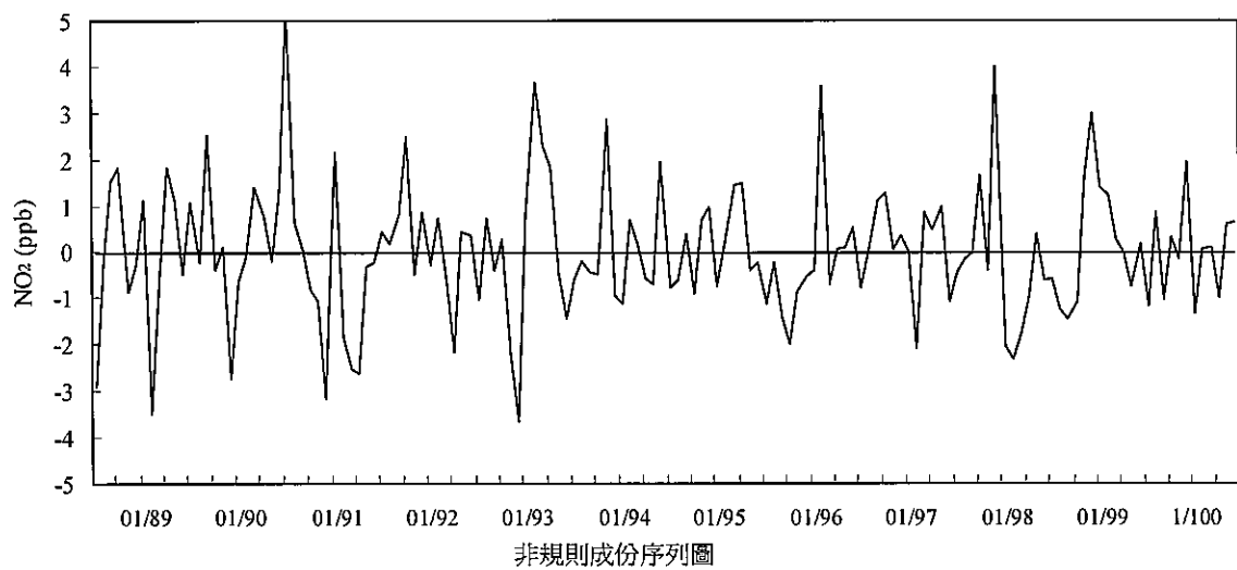
圖 2.1.5-13 麥寮站 88-100 年第二季間二氧化氮濃度趨勢圖
