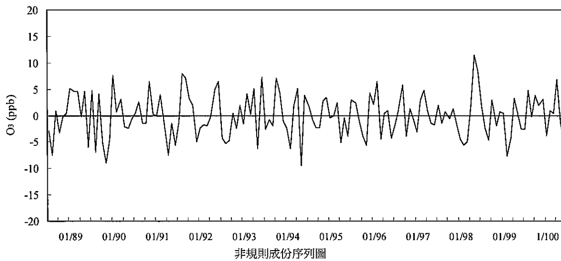
圖 2.1.5-8 台西站 88-100 年第二季間臭氧濃度趨勢圖
