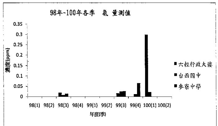
圖 2.1.4-6 98 年至 100 年 1-2 季 氨 物種彙整
