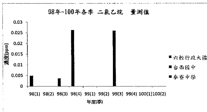
圖 2.1.4-9 98 年至 100 年 1-2 季 二氯乙烷 物種
