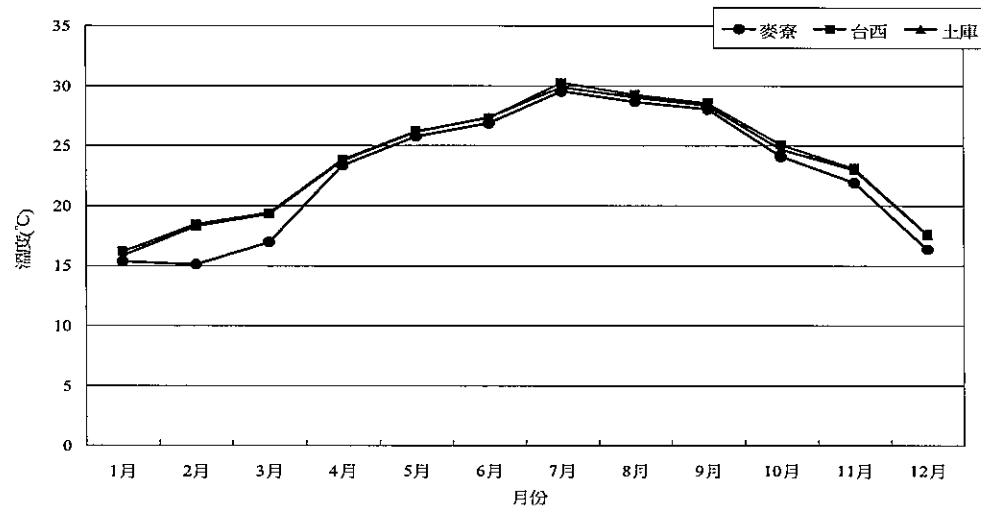
圖 2.1.6-12 92年台塑三測站月平均溫度資料比較圖
