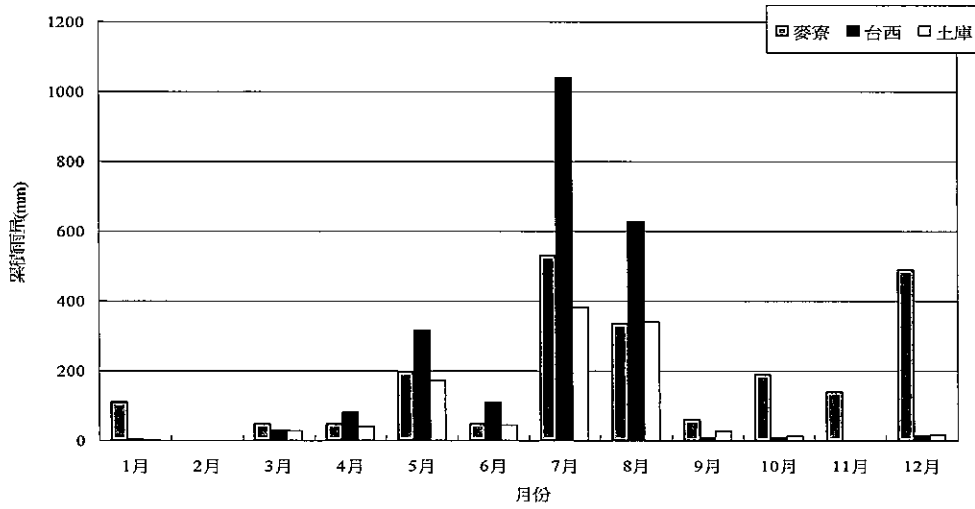
圖 2.1.6-13 88年台塑三測站月總雨量資料比較圖
