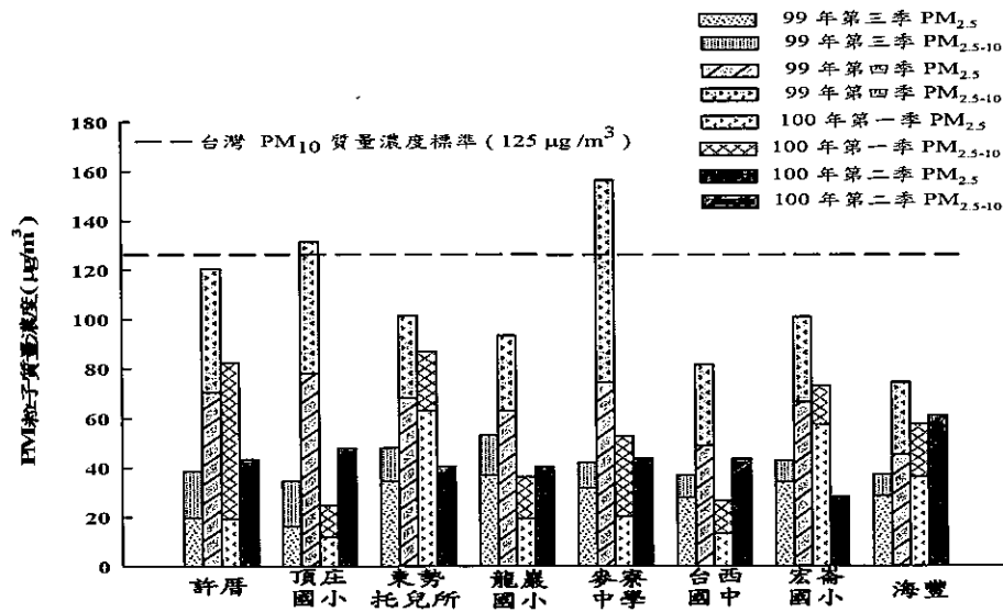
圖 2.1.1-6 本計畫四季各採樣點 PM 2.5 及 PM 2.5-10 質量濃度
