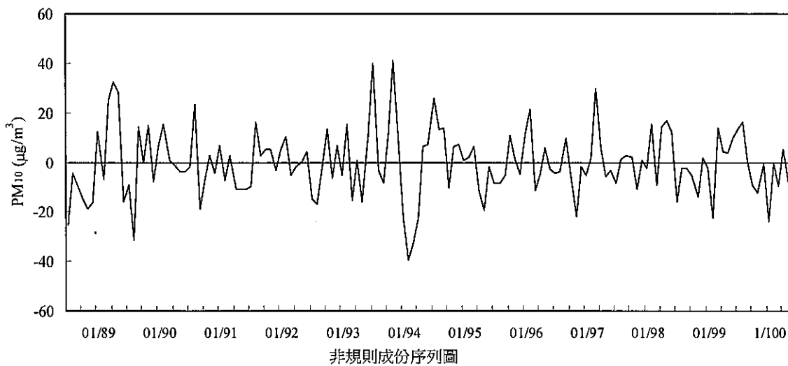
圖 2.1.5-12 土庫站 88-100 年第二季間懸浮微粒 PM 10 濃度趨勢圖
