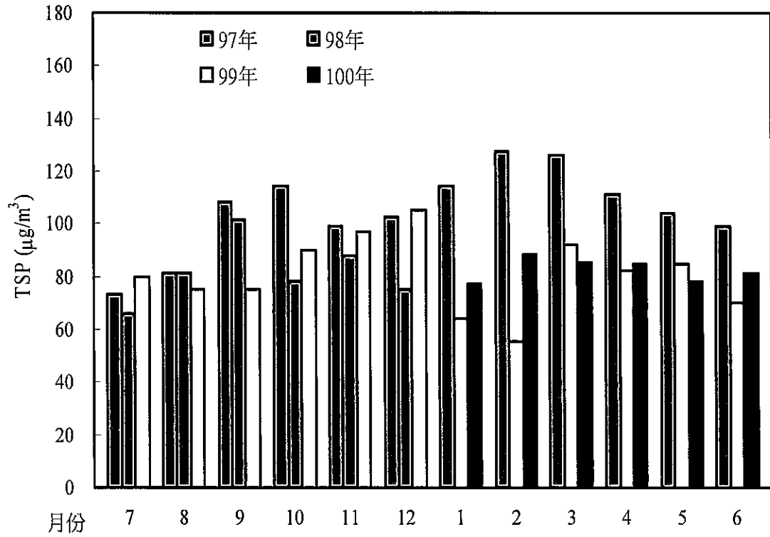
圖 2.1.5-64 麥寮站 100 年第二季與 99 年及 98 年總懸浮微粒 TSP 月平均比較圖
