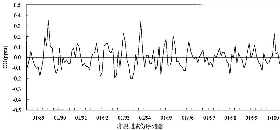
圖 2.1.5-4 麥寮站 88-100 年第二季間一氧化碳濃度趨勢圖
