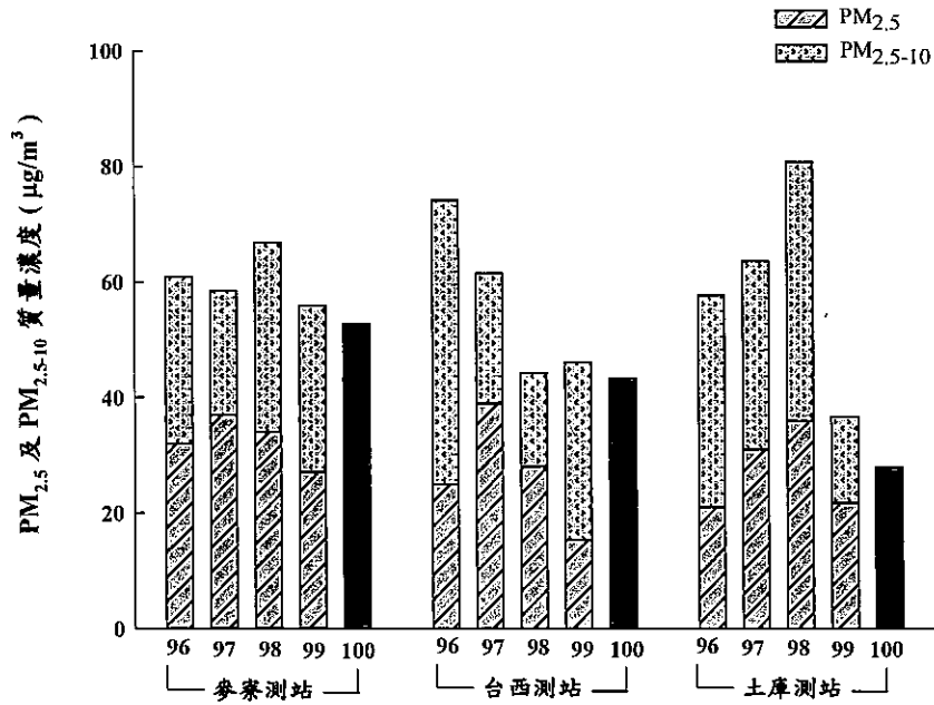
圖 2.1.2-1 歷年 96 - 100 第二季各採樣點 PM 2.5 及 PM 10 質量濃度
