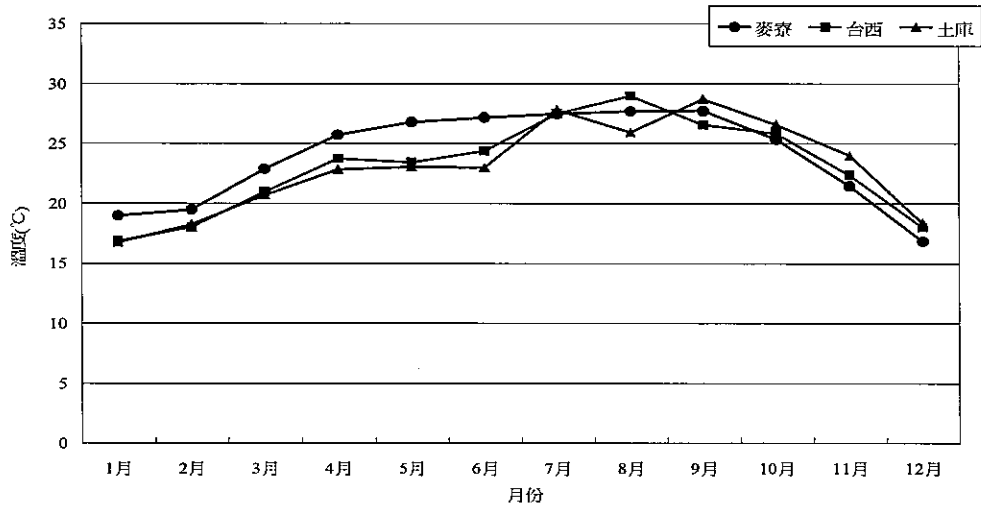
圖 2.1.6-10 88年台塑三測站月平均溫度資料比較圖
