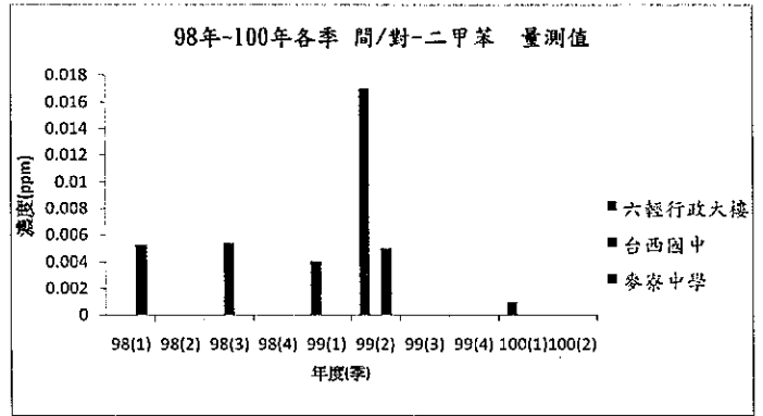
圖 2.1.4-18 98 年至 100 年 1-2 季 間/對-二甲苯 物
