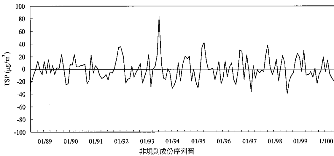
圖 2.1.5-20 台西站 88-100 年第二季間總懸浮微粒 TSP 濃度趨勢圖
