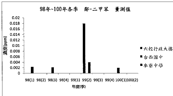
圖 2.1.4-17 98 年至 100 年 1-2 季 鄰-二甲苯 物
