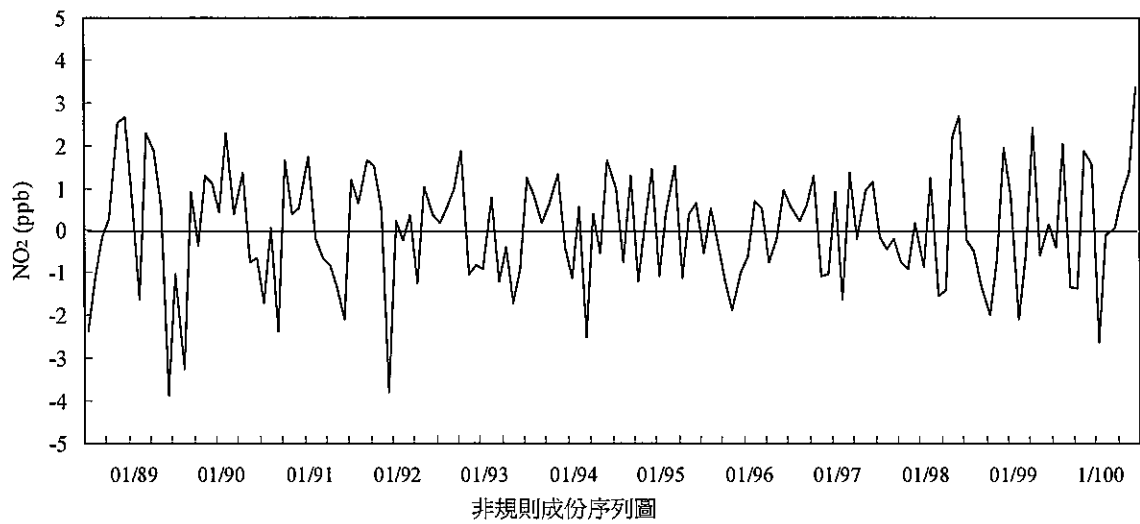
圖 2.1.5-15 土庫站 88-100 年第二季間二氧化氮濃度趨勢圖
