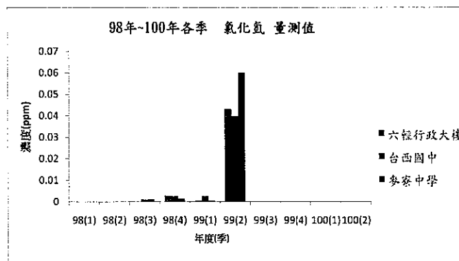
圖 2.1.4-11 98 年至 100 年 1-2 季 氯化氫 物種
