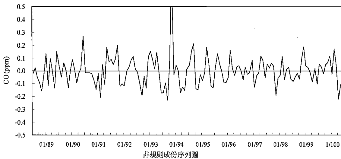
圖 2.1.5-6 土庫站 88-100 年第二季間一氧化碳濃度趨勢圖
