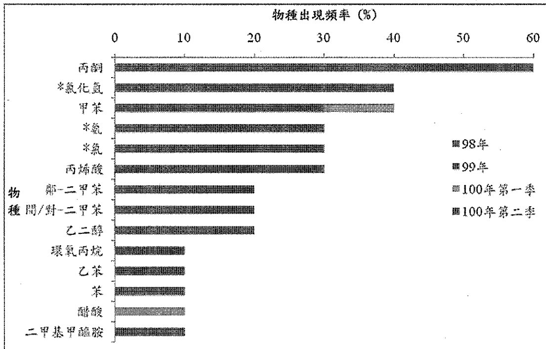
圖 2.1.4-4 麥寮中學歷年 (98、99~100年1季~2季) 共十季物種測得頻率排序
