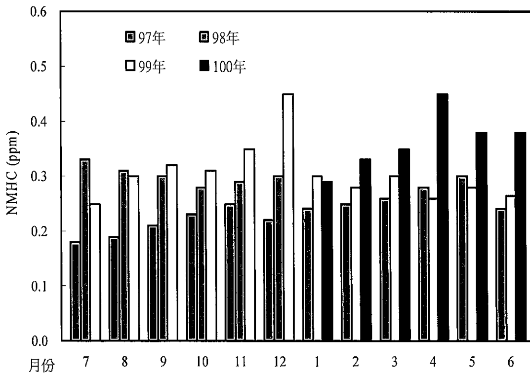
圖 2.1.5-61 麥寮站 100 年第二季與 99 年及 98 年 NMHC 月平均比較圖
