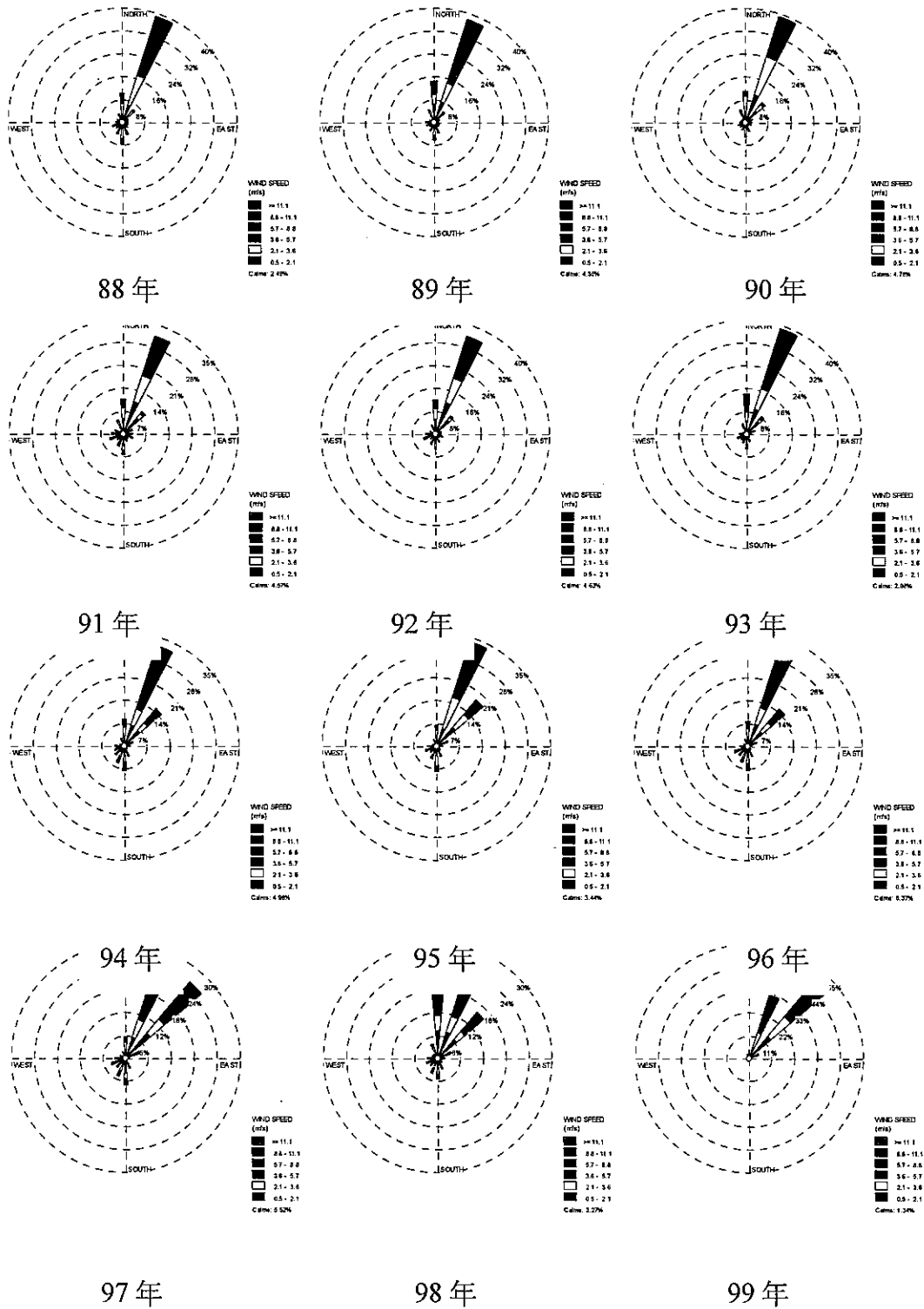
圖 2.6.1-4 88-99 年歷年麥寮站之風花圖
