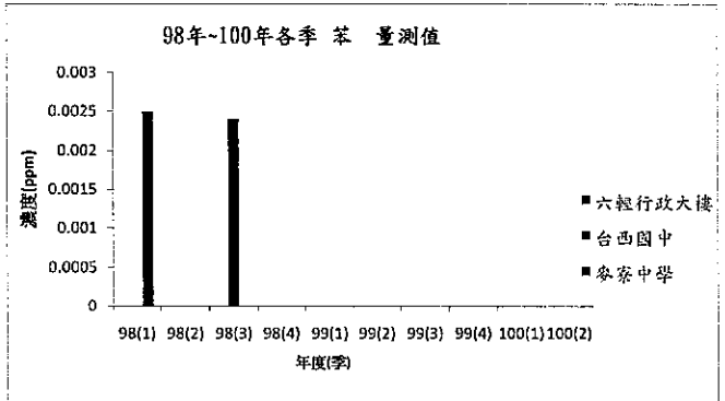
圖 2.1.4-20 98 年至 100 年 1-2 季 苯 物種彙
