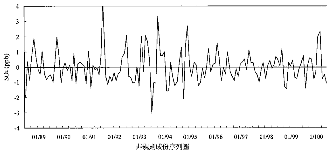
圖 2.1.5-3 土庫站 88-100 年第二季間二氧化硫濃度趨勢圖
