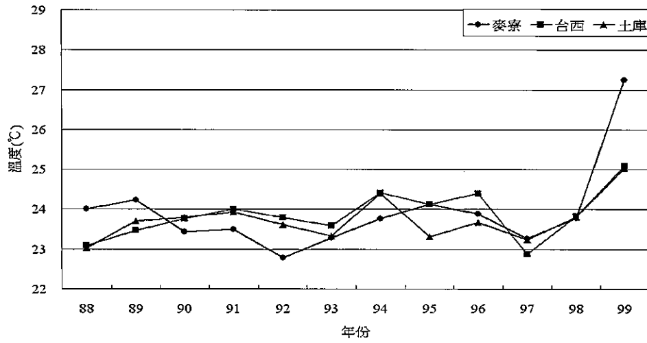
圖 2.1.6-2 台塑三測站歷年平均溫度資料比較圖
