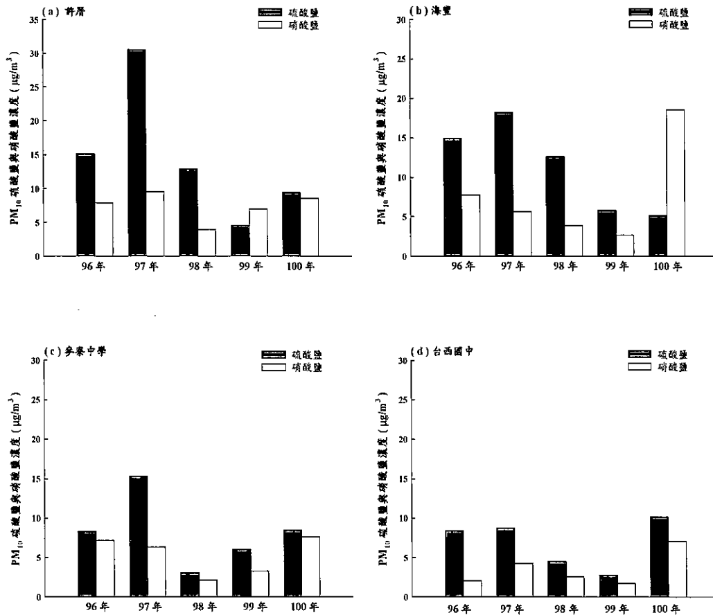
圖 2.1.2-2 96 - 100 年第二季各採樣點 PM 10 硫酸鹽與硝酸鹽濃度
