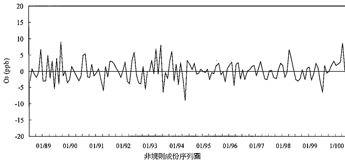
圖 2.1.5-9 土庫站 88-100 年第二季間臭氧濃度趨勢圖
