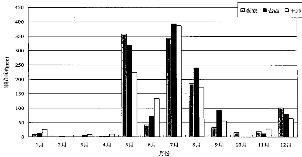
圖 2.1.6-14 91年台塑三測站月總雨量資料比較圖
