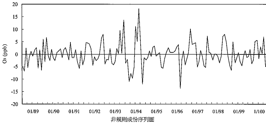
圖 2.1.5-7 麥寮站 88-100 年第二季間臭氧濃度趨勢圖
