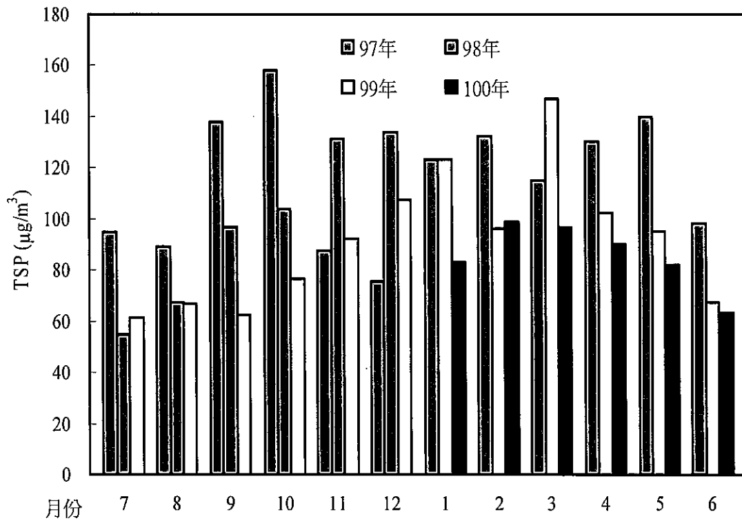
圖 2.1.5-65 台西站 100 年第二季與 99 年及 98 年總懸浮微粒 TSP 月平均比較圖
